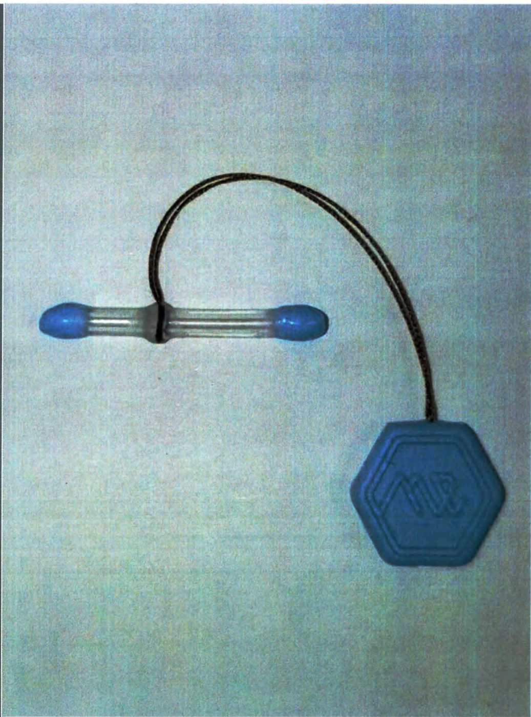
Внешний вид медицинского изделия «Шунт интракоронарный «МЕДИНЖ» по МЛЦК.942511.025 ТУ», размер 2,75
