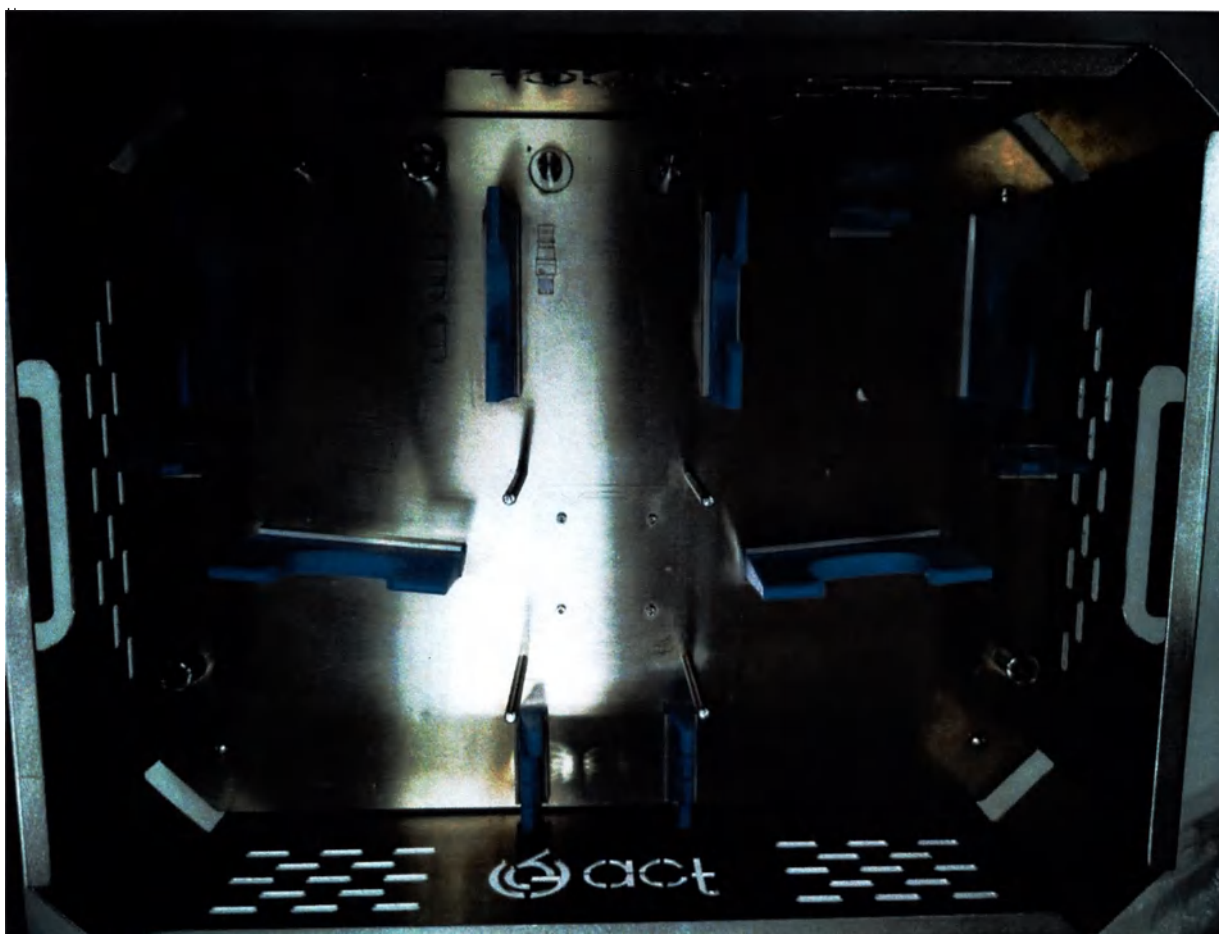
Рисунок 10. Стерилизационный контейнер (тип 3)
