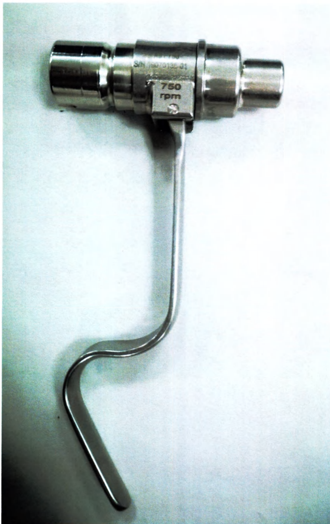
Рисунок 18. Насадка для проводки спиц (0.5-1.5 REF A01 740; 1.6-2.5 REF A01 741; 2.6-3.2 REF A01 750; 3.3 – 4.0 REF A01 751 мм)
