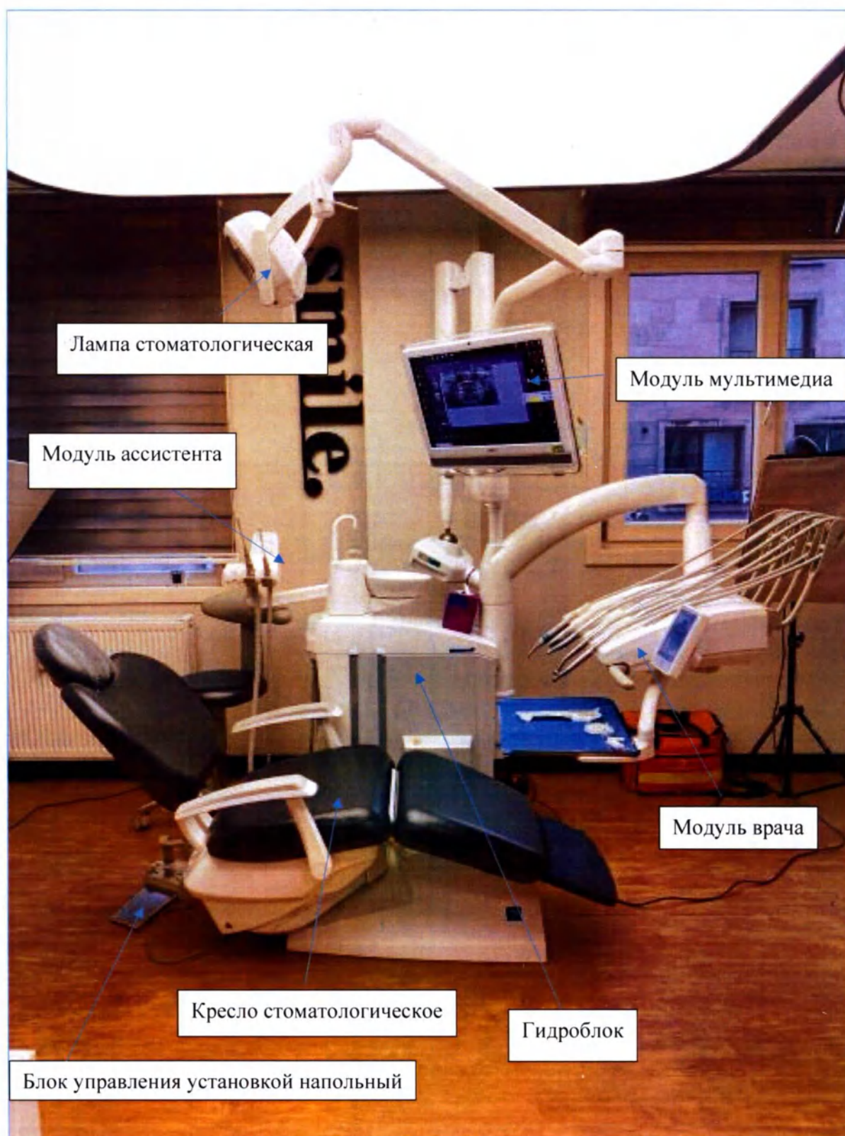
Общий вид стоматологической установки, установленной в кабинете, Установка стоматологическая STERN WEBER S380 TRc, вариант исполнения Continental
