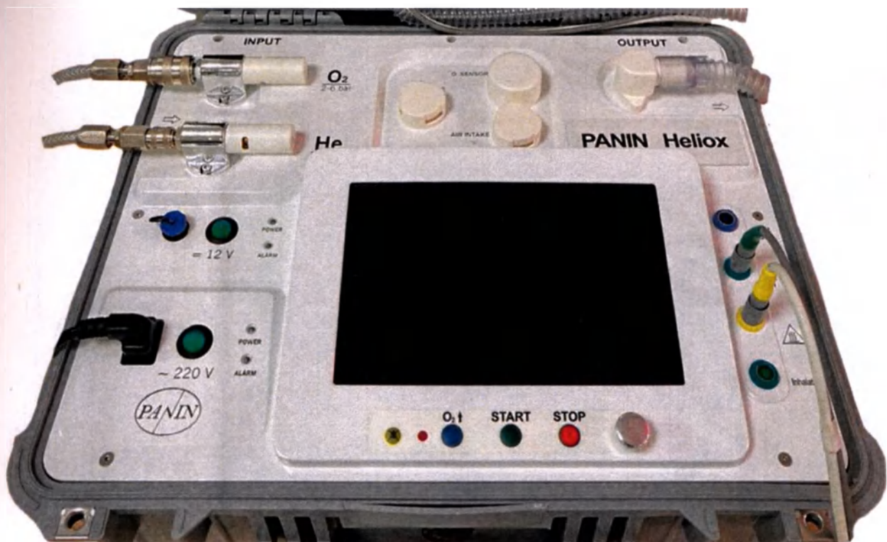
Рисунок 2 – Блок управления, ГЛКС.П.01.00.00.000
