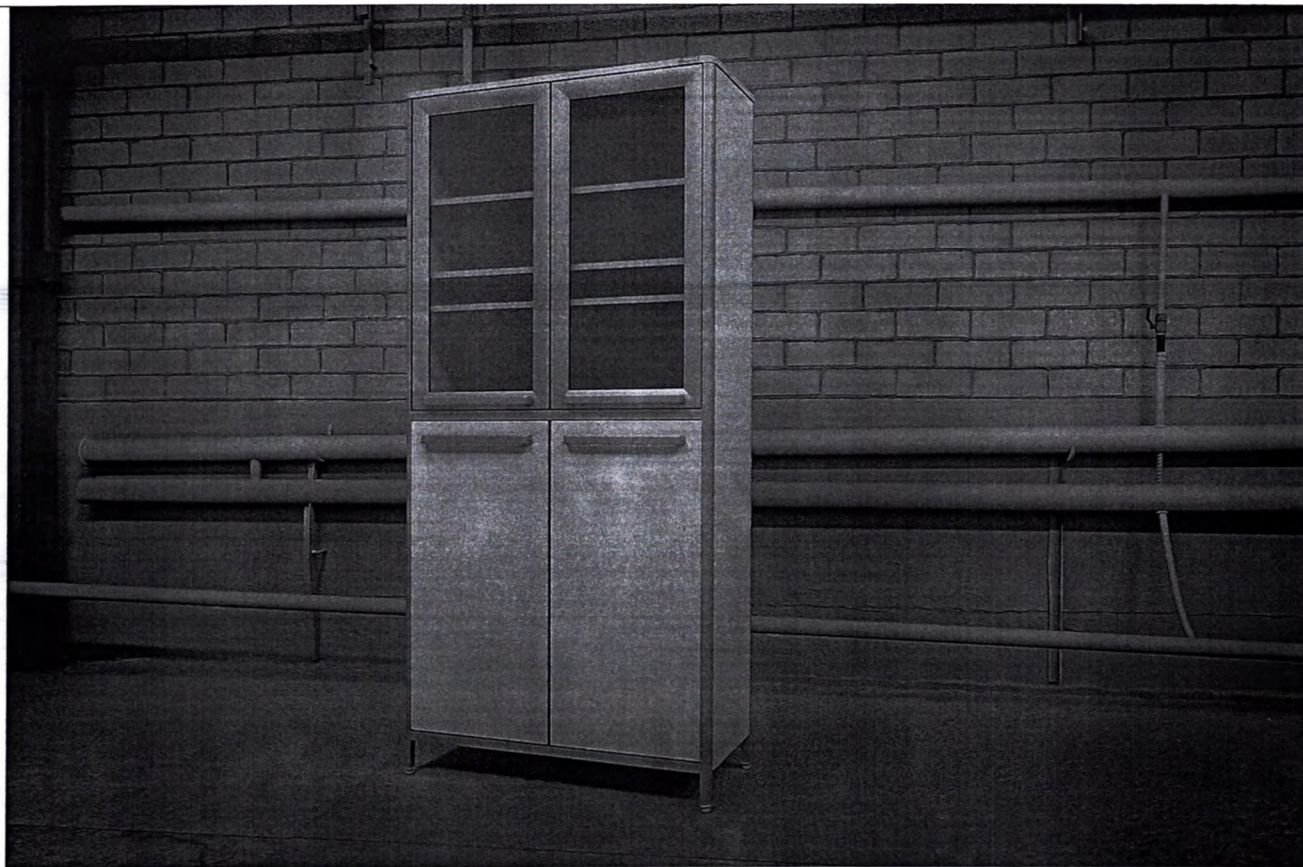
15. Шкаф для хранения лекарственных средств ШМН-2.2М по ТУ 32.50.30-030-51768895-2023
