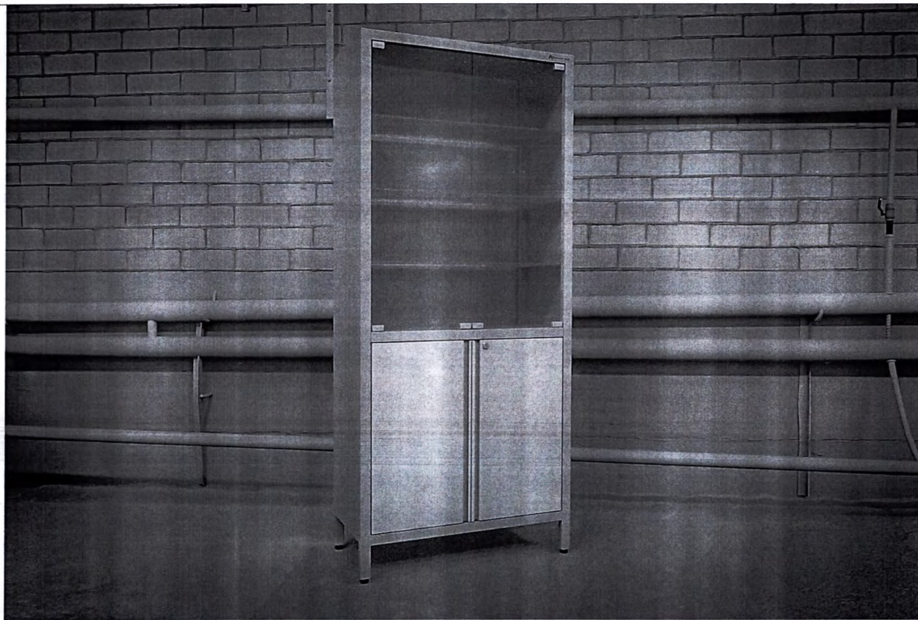
47. Шкаф для хранения лекарственных средств ШК-2.5 по ТУ 32.50.30-030-51768895-2023
