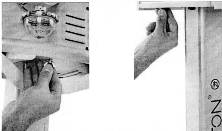
Рисунок 3.2 – Закрепление электронного блока на тележке
