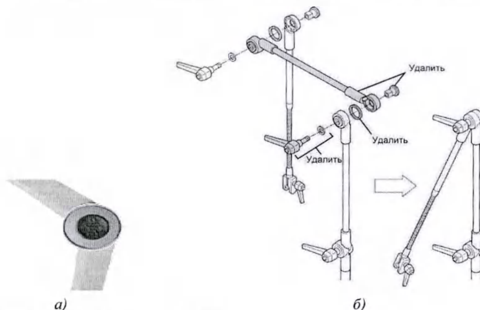
Рисунок 3.4 – Регулирование положения сегментов штанги: а) модель WYAM030; б) модель WYAM010
