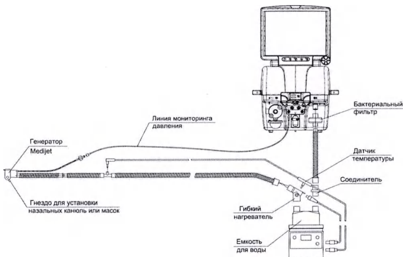
Рисунок 3.14 – Схема сборки для режима nCPAP (с использованием генератора потока Medijet®) с увлажнителем MR850 или TEBJAP (с сервоконтролем)
