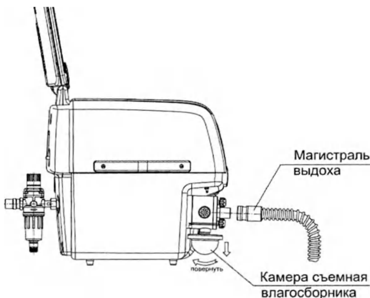
Рисунок 3.20 – Удаление жидкости из съемной камеры влагосборника
