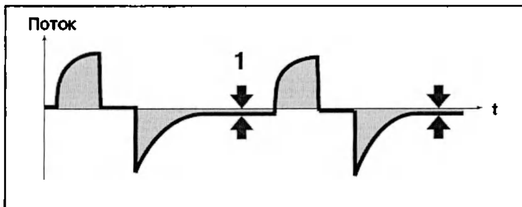
Рисунок 4.14 – Эффект затягивания потока выдоха по причине увеличения сопротивления фильтра
