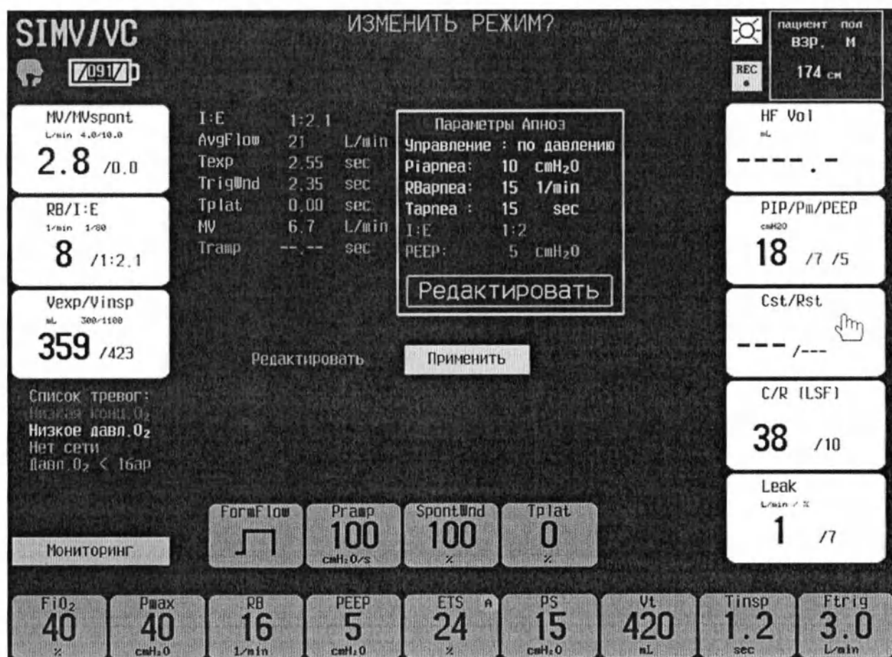
Рисунок 4.2 – Основной экран с окном связанных параметров
