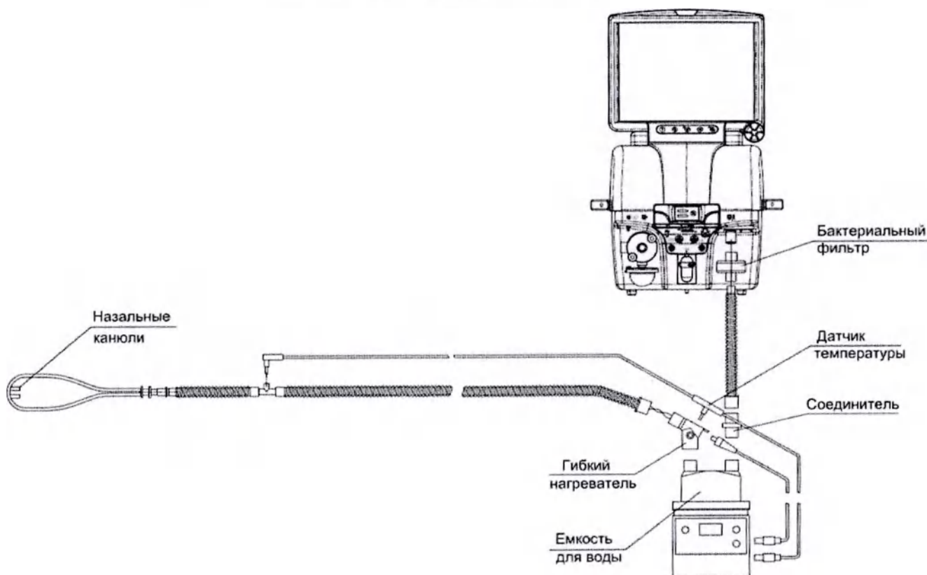
Рисунок 3.16 а) – Схема сборки для режима HF_O2_неонатальный с увлажнителем MR850 или ТЕВЛАР (с сервоконтролем)
