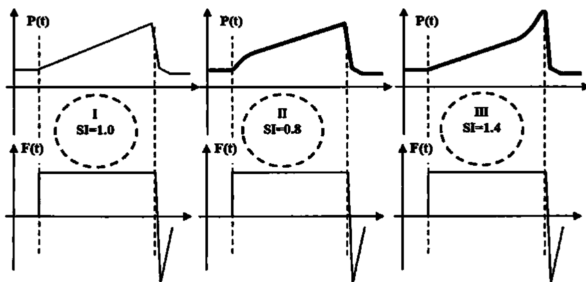
Рисунок 1 Пр. 2.7 – графики давления при нормальном ( SI = 1 ), низком ( SI < 1 ) и высоком ( SI > 1 ) стресс-индексе
