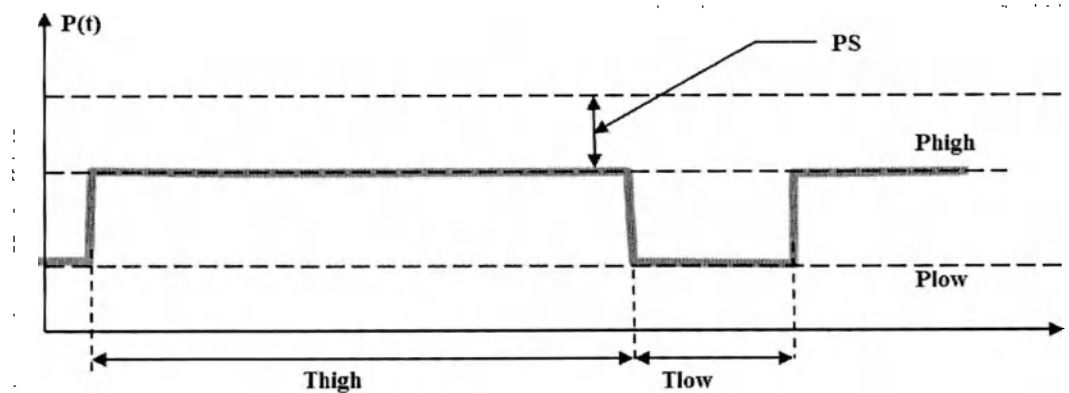
Рисунок Пр. 1.8 – Работа аппарата в режиме APRV
