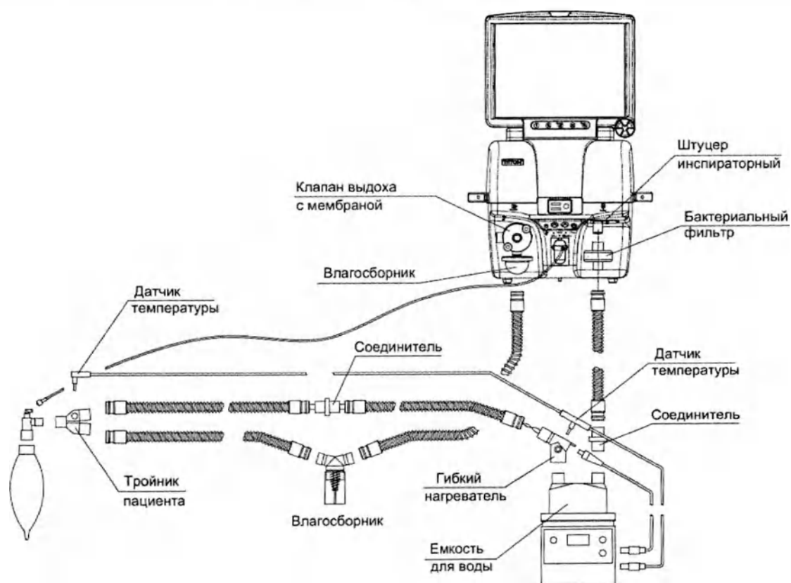
Рисунок 3.8 б) – Схема сборки дыхательного контура TECH.233015 с подогреваемым шлангом и датчиком температуры для увлажнителя MR850 или ТЕВЛАР (с сервоконтролем)
