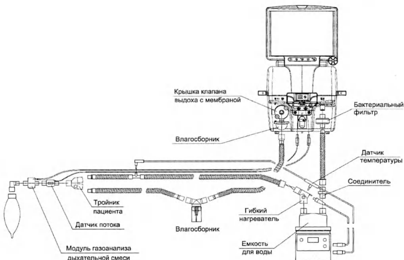
Рисунок 3.13 – Схема сборки неонатального контура с датчиком потока с одним влагосборником с увлажнителем MR850 или TEBJAP (с сервоконтролем)
