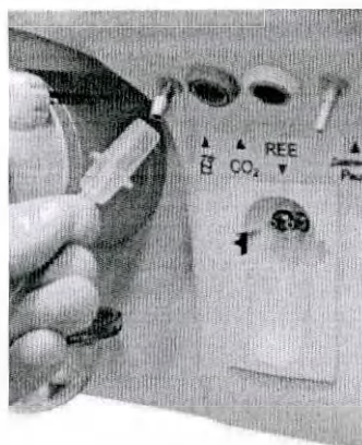
Рисунок 4.15 – Подключение соединительной трубки небулайзера к штуцеру на передней панели аппарата
