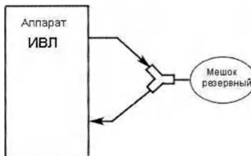
Рисунок 6.6 – Схема для проверки задаваемого объема
