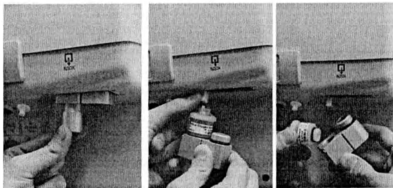
Рисунок 6.4 – Замена датчика \text{FiO}_2
