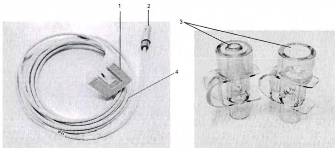
Рисунок 5.1 – Внешний вид капнографа прямого потока
