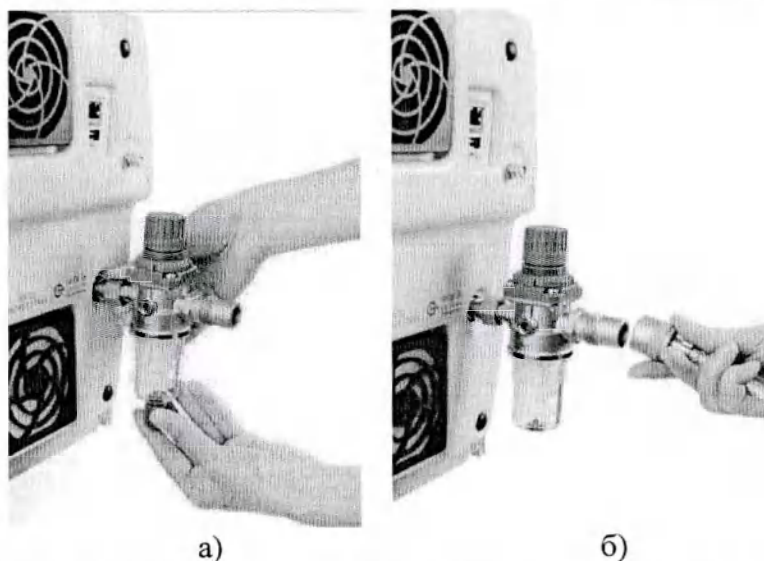
Рисунок 3.21 – Подключение фильтра-регулятора (а) и кислородного шланга (б) к аппарату
