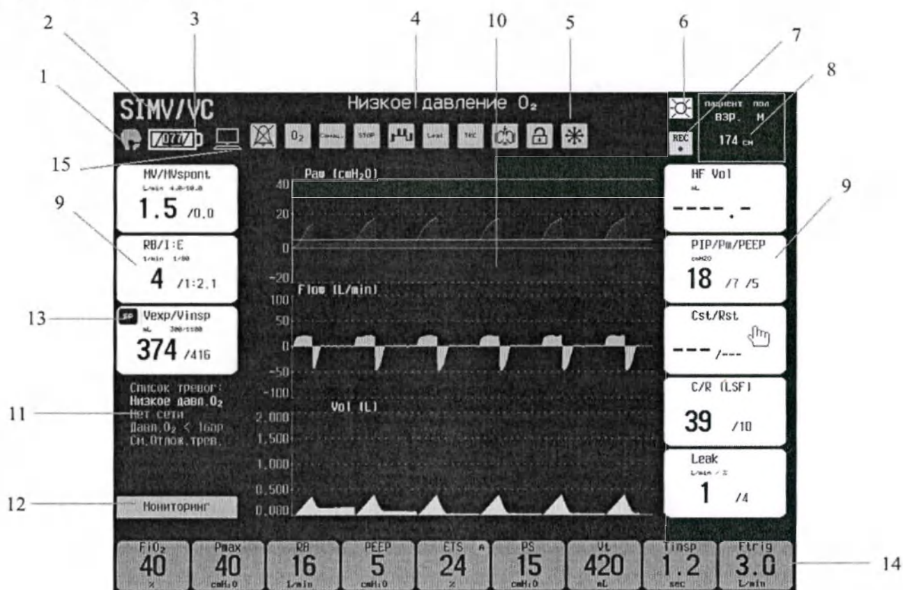
Рисунок 4.3 – Окно основного экрана
