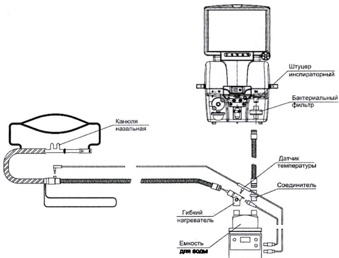
Рисунок 3.16 б) – Схема сборки для режима HF_O2 (детский, взрослый) с увлажнителем MR850 или ТЕВЛАР (с сервоконтролем)
