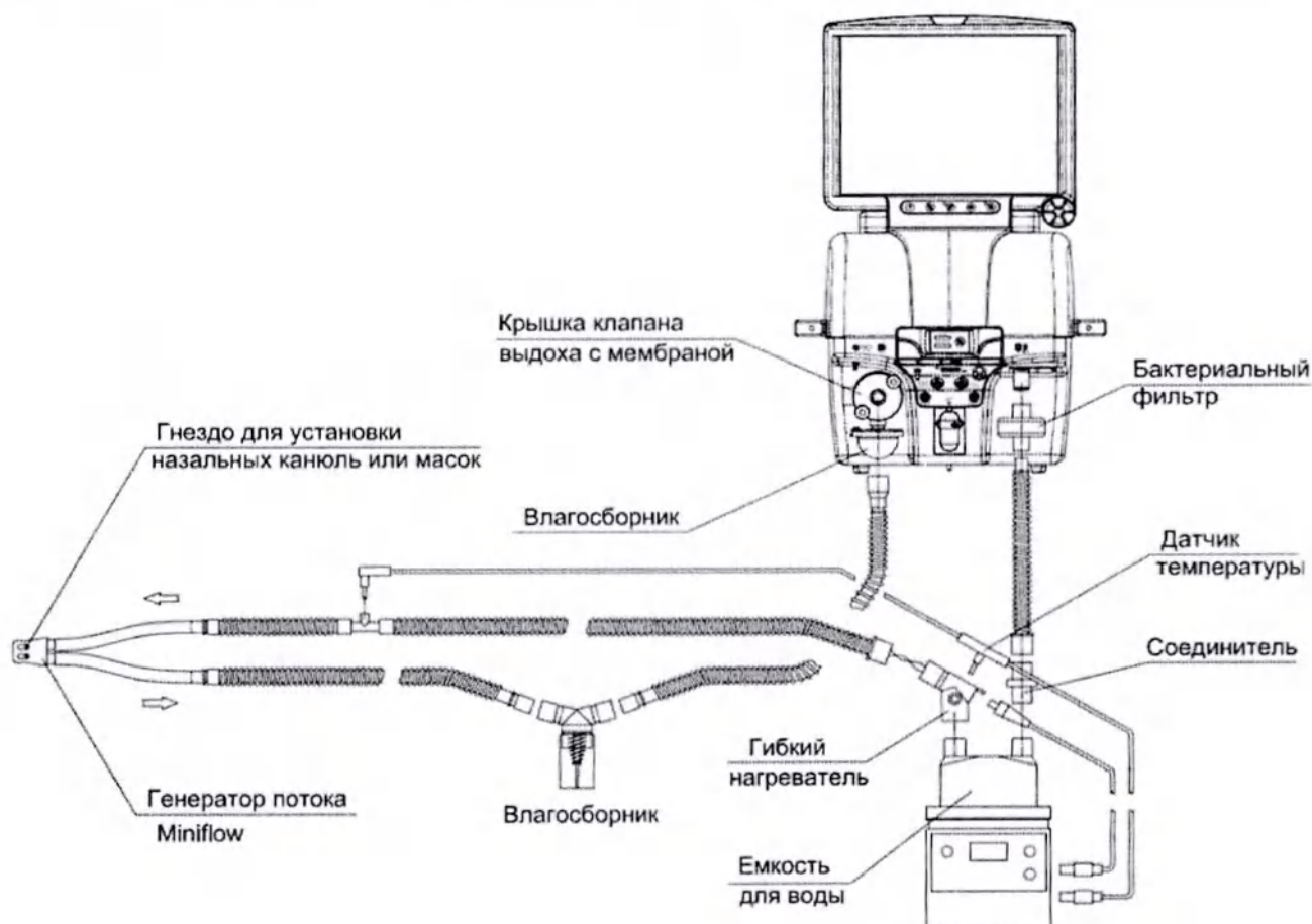
Рисунок 3.18 – Схема сборки для режима nIMV (с использованием генератора потока Miniflow) с увлажнителем MR850 или ТЕВЛАР (с сервоконтролем)
