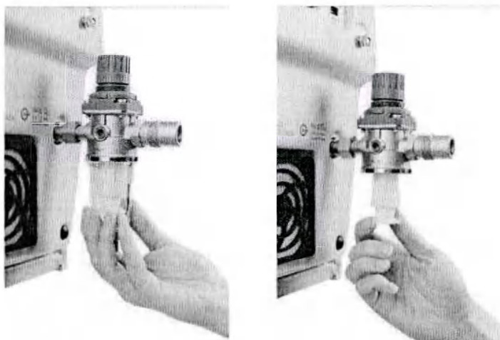
Рисунок 6.2 – Отсоединение корпуса фильтра-регулятора
