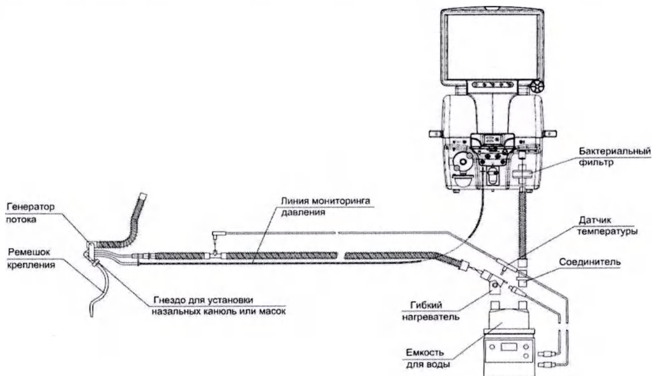
Рисунок 3.15 – Схема сборки для режима nCPAP с увлажнителем MR850 или ТЕВЛАР (с сервоконтролем)
