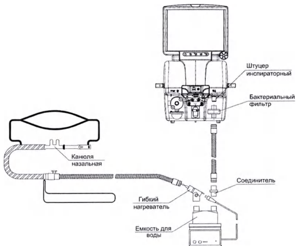
Рисунок 3.17 – Схема сборки для режима HF_O2 с увлажнителем MR810
