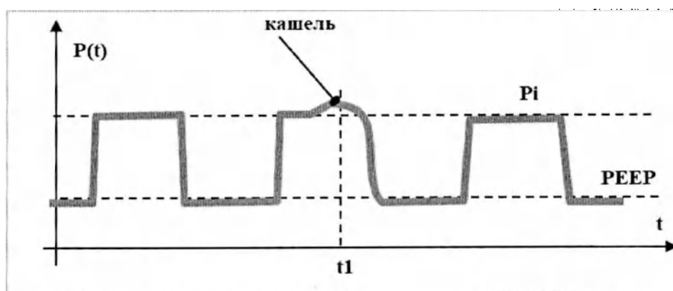
Рисунок 2 Пр. 1.15 – Кашель в режимах с контролем по давлению
