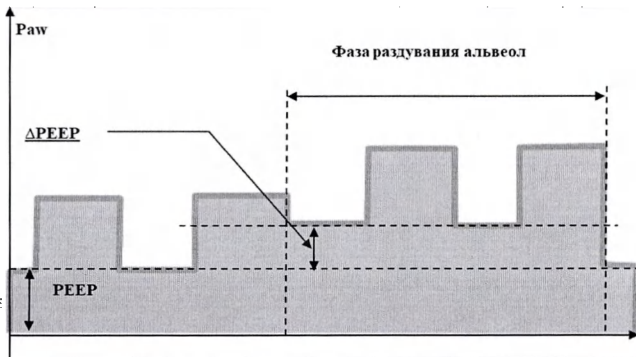
Рисунок 4.7 – Форма P_{aw} при активной фазе маневра раскрытия альвеол
