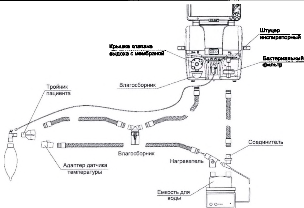
Рисунок 3.10 – Схема сборки многоразового и одноразового дыхательного контура с увлажнителем MR810
