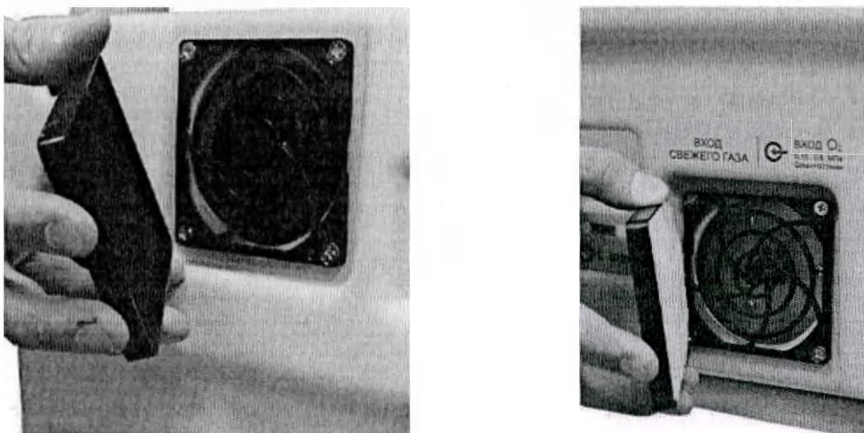
Рисунок 6.1 – Очистка и замена пылевого фильтра
