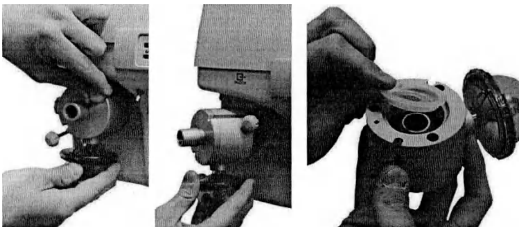
Рисунок 6.3 – Отсоединение съемной части клапана выдоха
