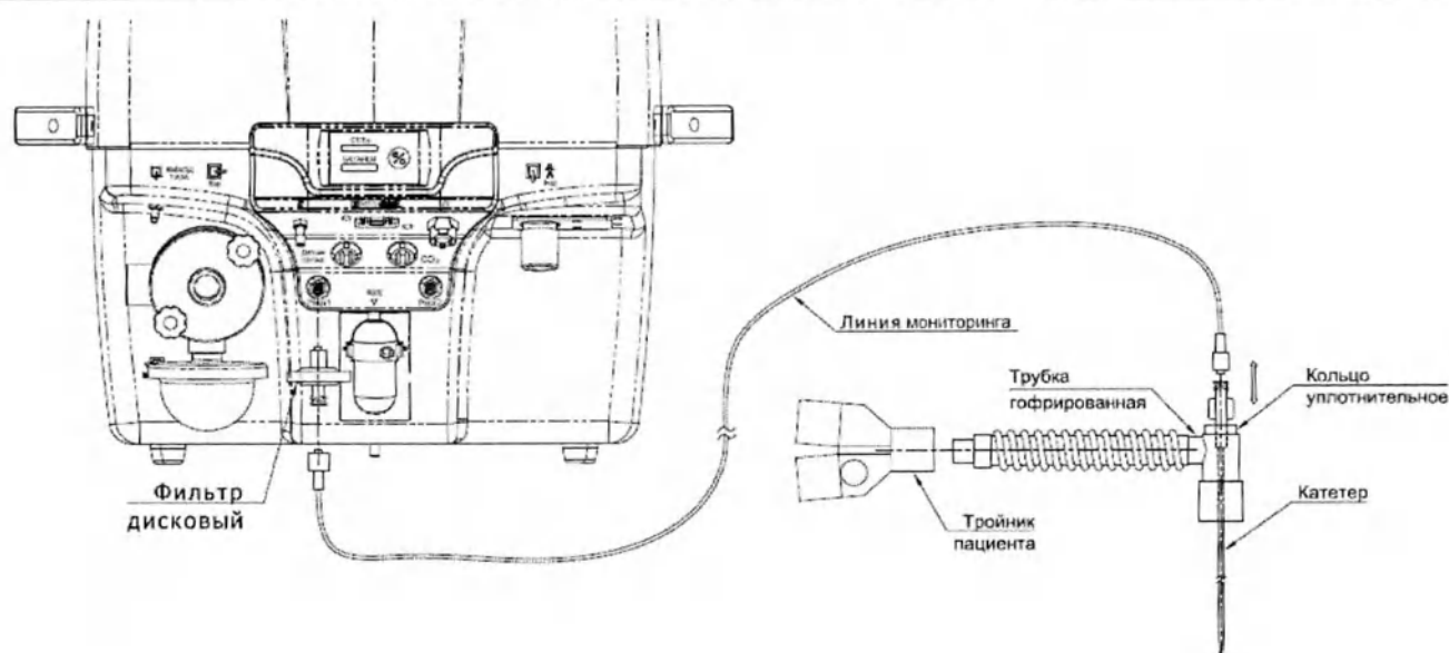
Рисунок 5.16 б – Схема подключения трахеального катетера (вариант с двумя штуцерами)
