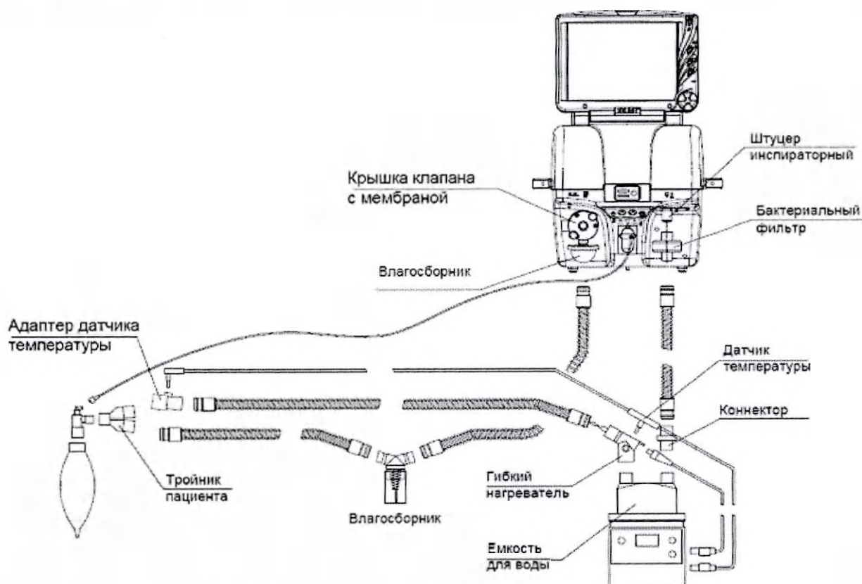
Рисунок 3.8 а) – Схема сборки дыхательного контура многоразового и одноразового типа с подогреваемым шлангом и датчиком температуры для увлажнителя MR850 или ТЕВЛАР (с сервоконтролем)
