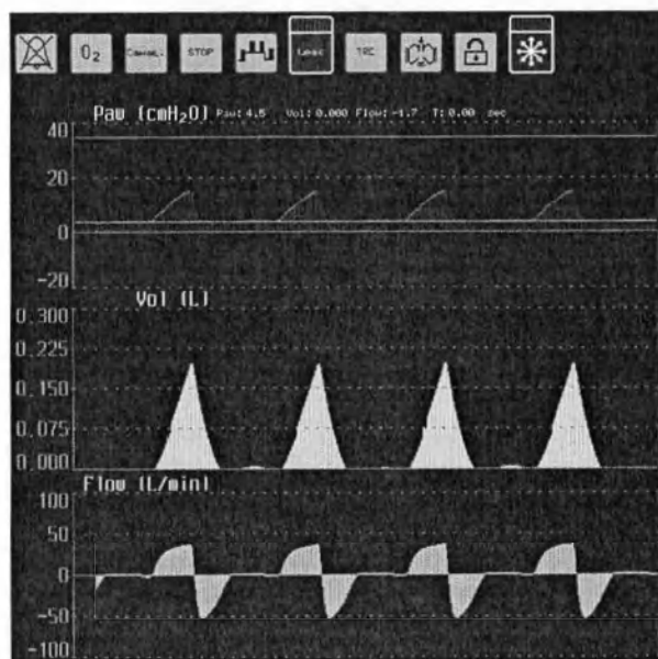
Рисунок 4.9 – Нажатая кнопка «заморозки» кривых
