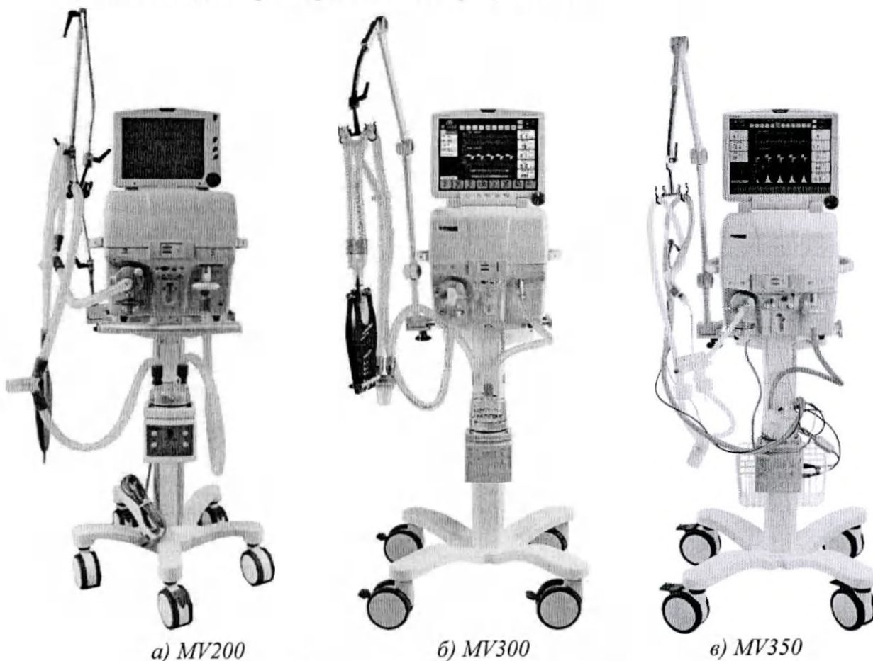
Рисунок 1.1 - Внешний вид аппарата
