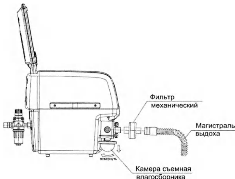
Рисунок 3.7 – Подключение фильтра выдоха
