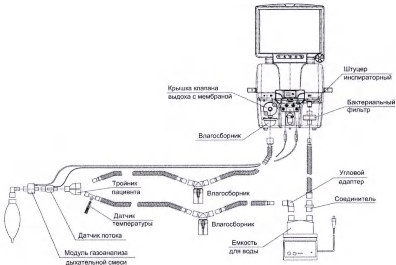
Рисунок 3.12 – Схема сборки неонатального контура с датчиком потока с двумя влагоборниками с увлажнителем VH-2000 или ТЕВЛАР (без сервоконтроля)
