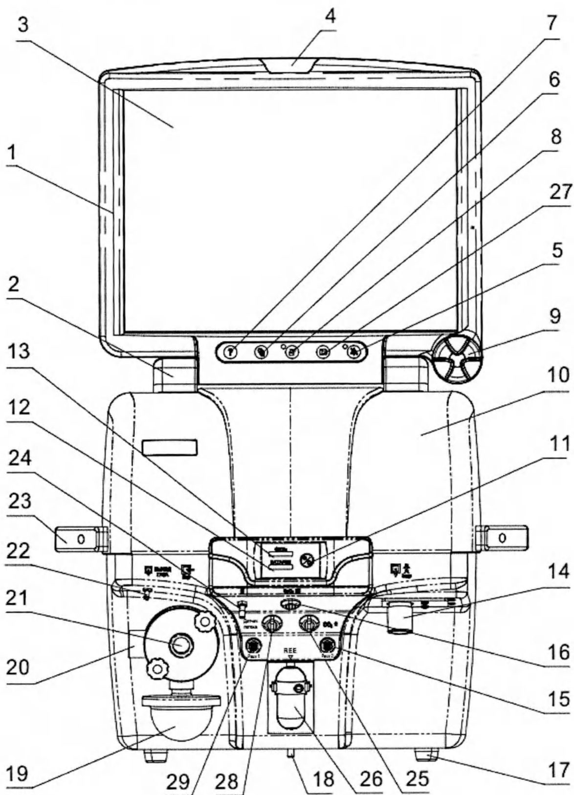
Рисунок 2.1 б) – Вид электронного блока спереди (MV300, MV350)
