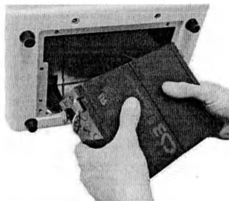
Рисунок 6.5 – Замена встроенных аккумуляторов
