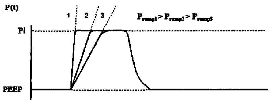
Рисунок 4.5 – Настройка Pramp
