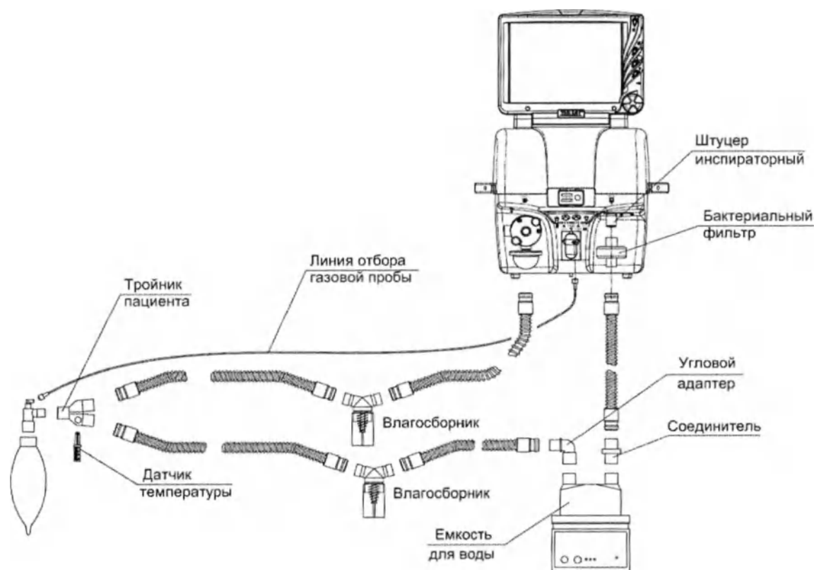
Рисунок 3.11 – Схема сборки дыхательного контура многоразового и одноразового типа с увлажнителем VH-2000 или ТЕВЛАР (без сервоконтроля)
