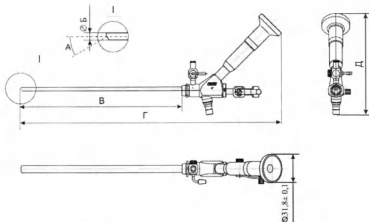
Рисунок 1. Цистоуретроскоп конструкционного исполнения 3
