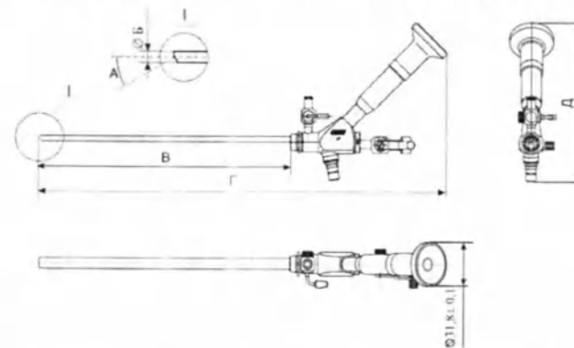
Рисунок 1. Цистоуретроскоп конструктивного исполнения 3
