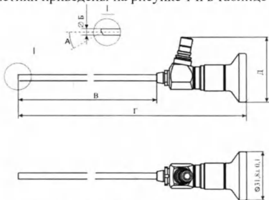
Рисунок 1. Цистоуретроскоп конструктивного исполнения 1
