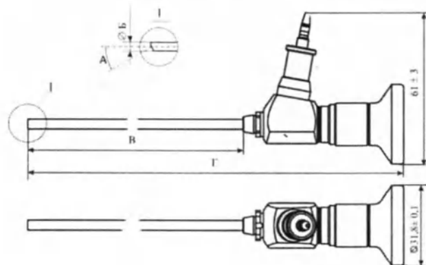
Рисунок 1. Цистоуретроскоп конструкционного исполнения 2
