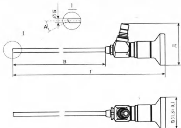
Рисунок 1. Цистоуретроскоп конструкционного исполнения 1
