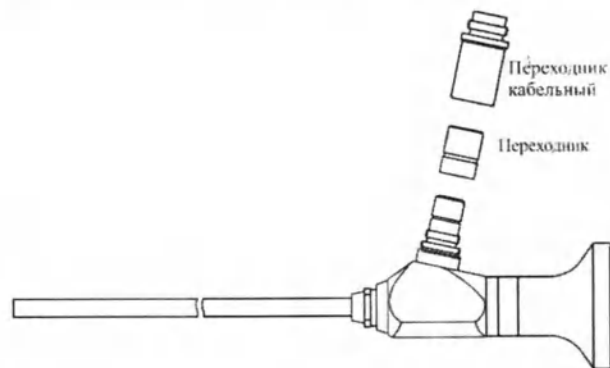
Рисунок 2. Цистоуретроскоп «ЭлеПС» конструкционного исполнения 1
