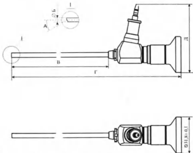
Рисунок 1. Цистоуретроскоп конструкционного исполнения 2
