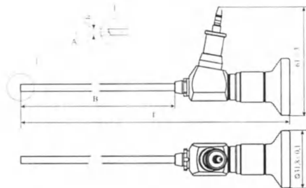
Рисунок 1. Гистероскоп конструкционного исполнения 2
