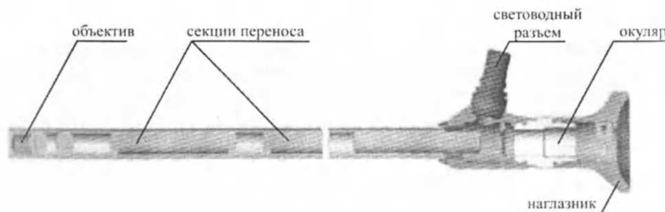
Рисунок 3. Эндоскоп «ЭлеПС»
