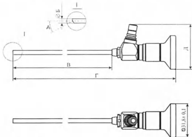
Рисунок 1. Гистероскоп конструктивного исполнения 1
