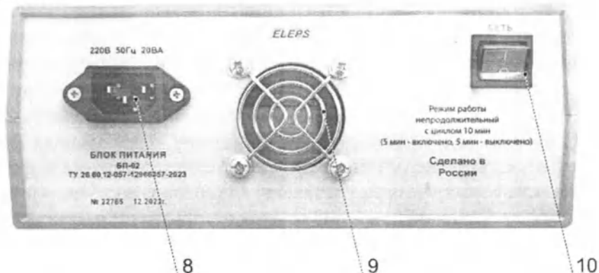
Рисунок 7. Блок питания БП02. Задняя панель
