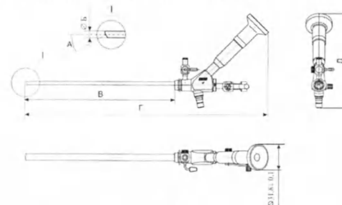
Рисунок 1. Гистероскоп конструкционного исполнения 3
