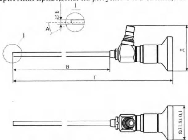
Рисунок 1. Гистероскоп конструктивного исполнения 1
