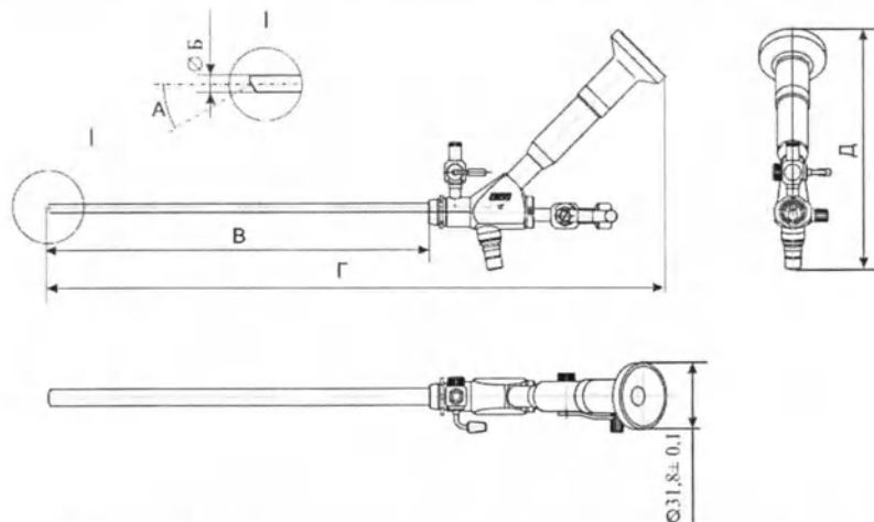
Рисунок 1. Гистероскоп конструкционного исполнения 3
