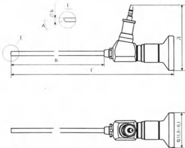
Рисунок 1. Гистероскоп конструкционного исполнения 2
