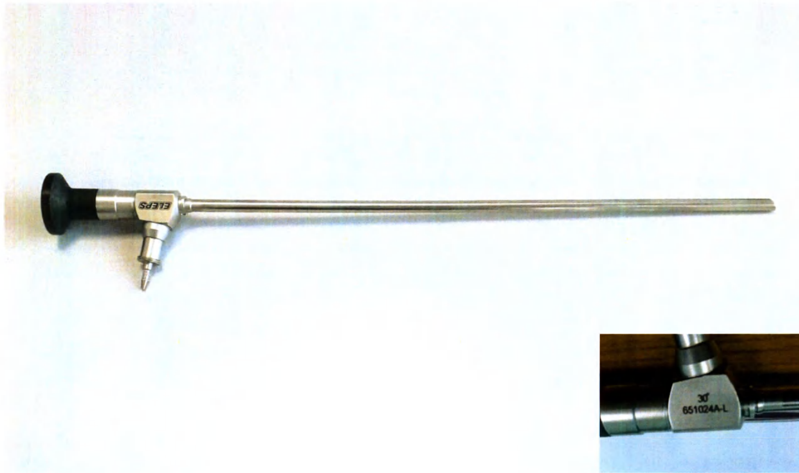
Торакоскоп «ЭлеПС» по ТУ 26.60.12-057-12966357-2023 в вариантах исполнения с общими принадлежностями Торакоскоп ТО2-065-290-30 «ЭлеПС» ТУ 26.60.12-057-12966357-2023 (конструкционное исполнение 2)
