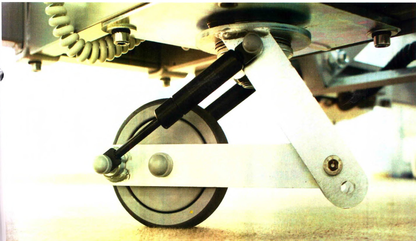
Рисунок 16. Пятое колесо
