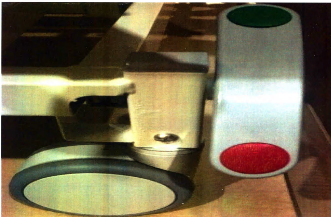
Рисунок 11. Колесо в исполнении: с тормозом диаметром 125 мм
