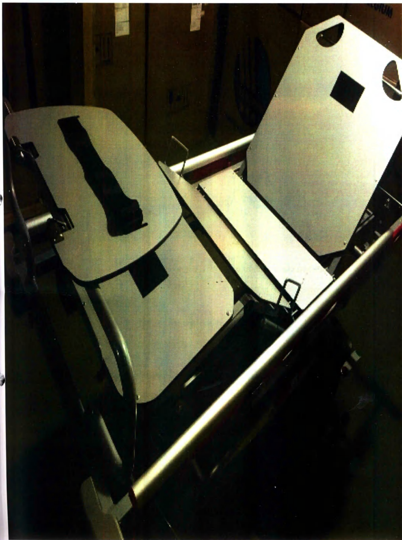
Рисунок 8. Ложемент каталки
