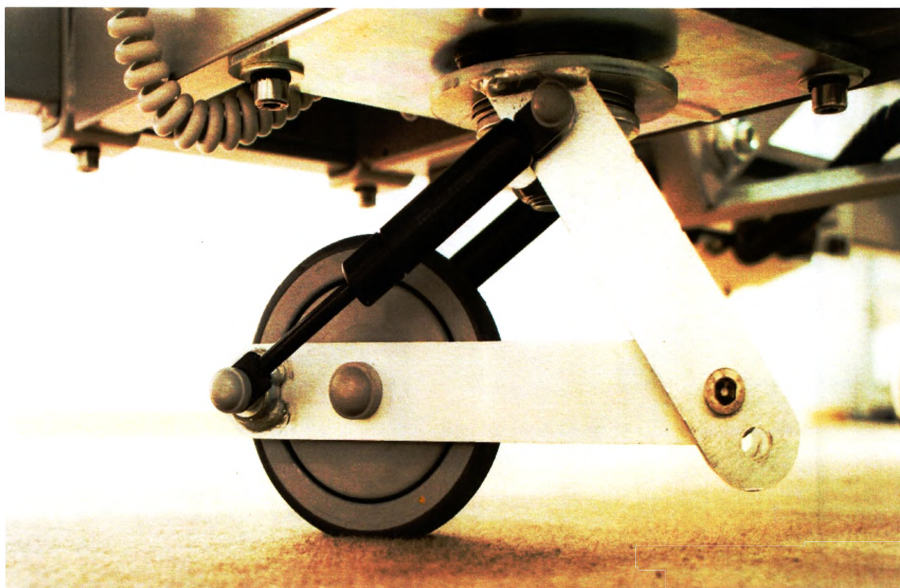
Рисунок 32. Пятое колесо
