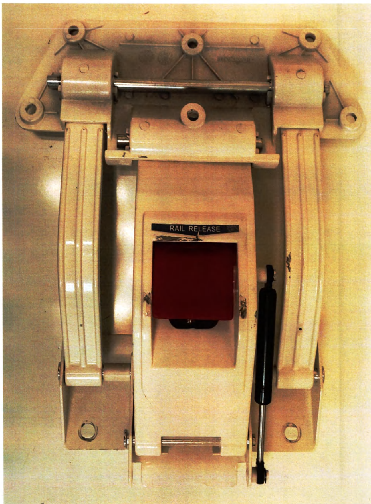
Рисунок 47. Держатель бокового ограждения
