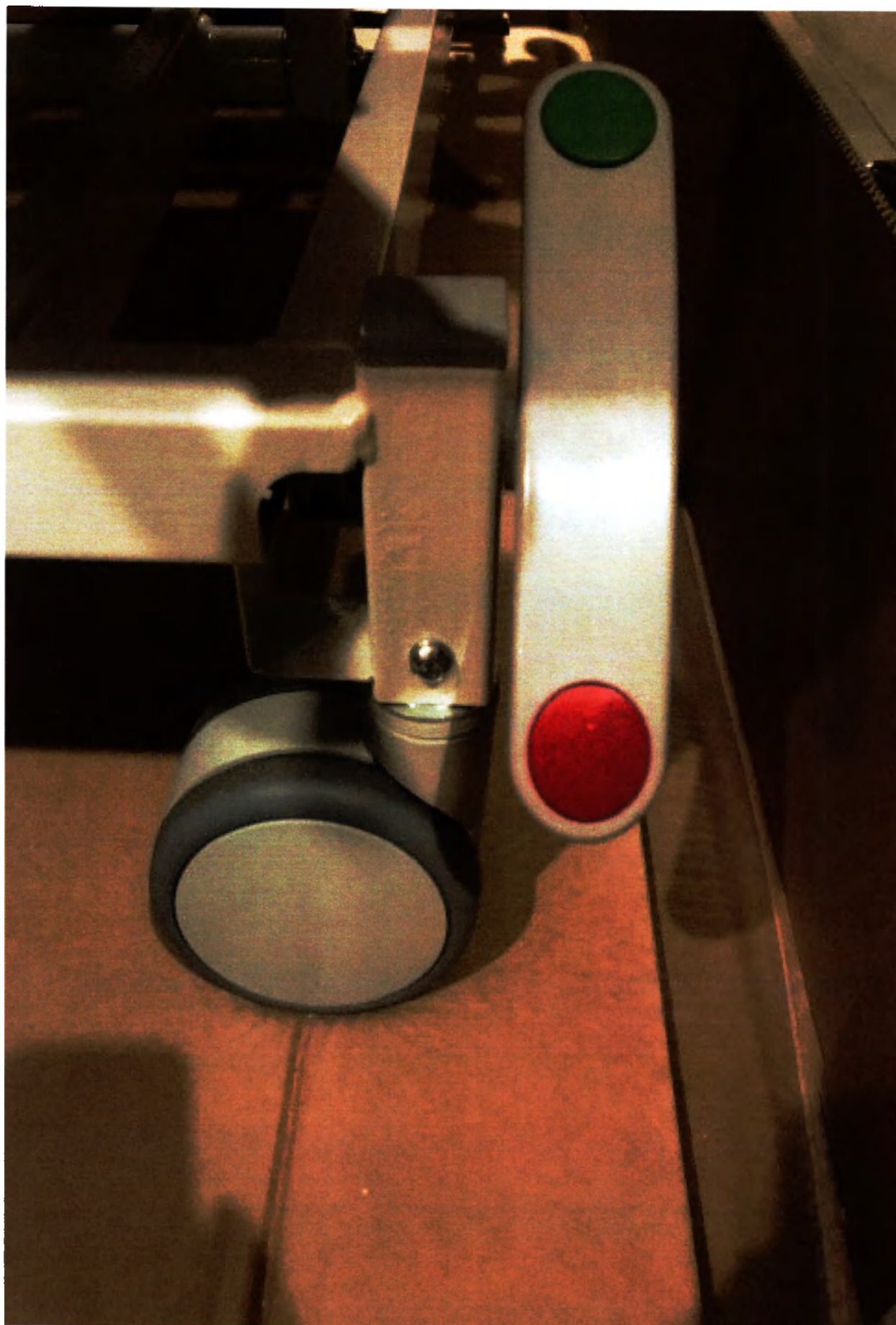
Рисунок 21. Привод тормоза на 4 колеса
