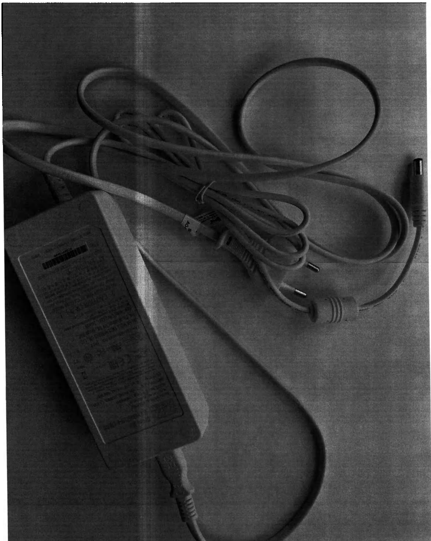
Фотографическое изображение 15. Концентратор кислорода портативный HORIZON® P5. Кабель и блок питания переменного тока, модель GSM90B19.
