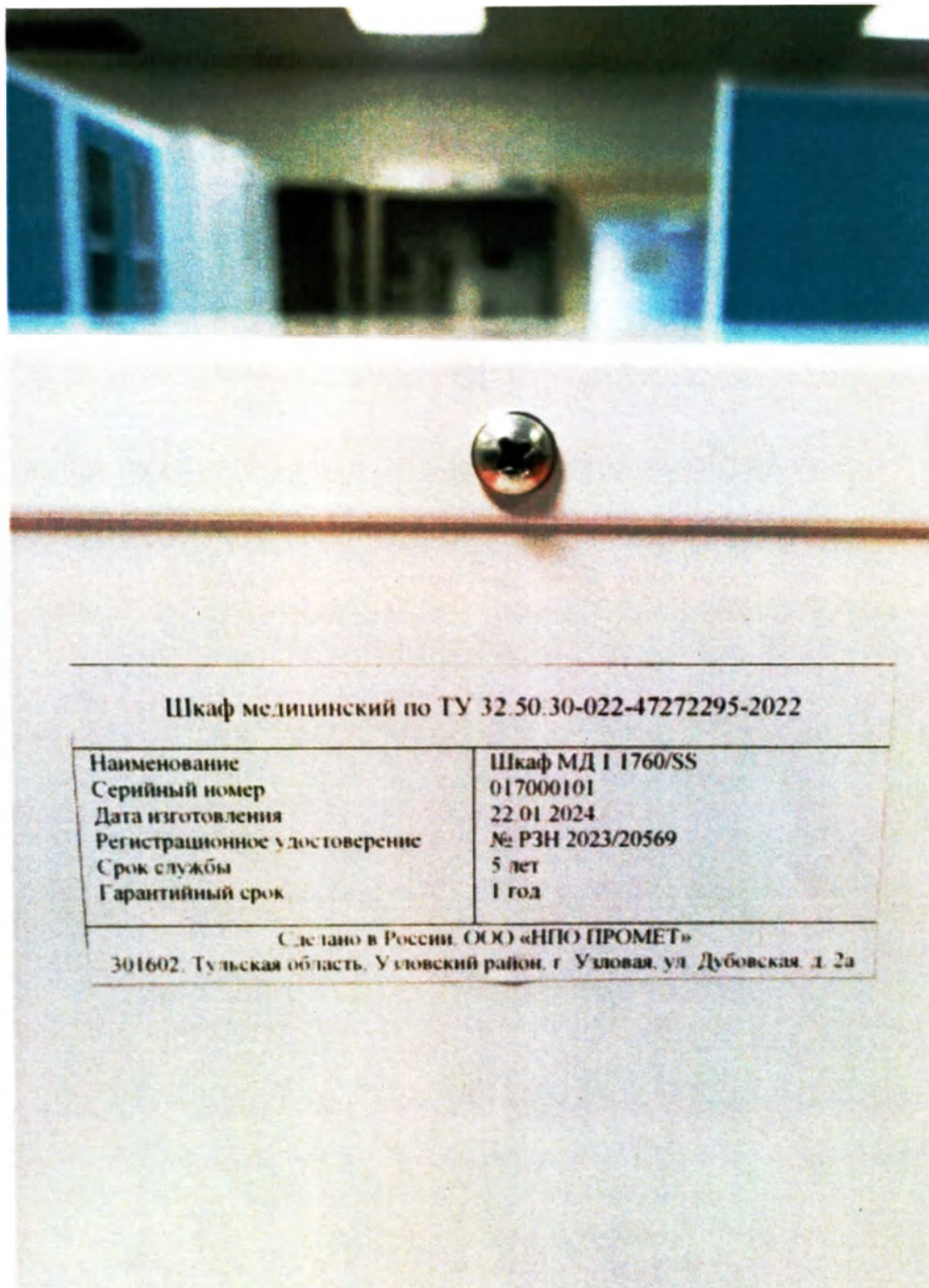
13.3. Шкаф МД 1 1760/SS (вид с этикеткой)
