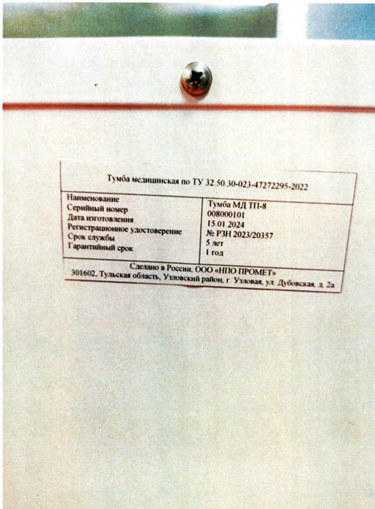
8.3. Тумба МД ТП-8 (вид с этикеткой)
