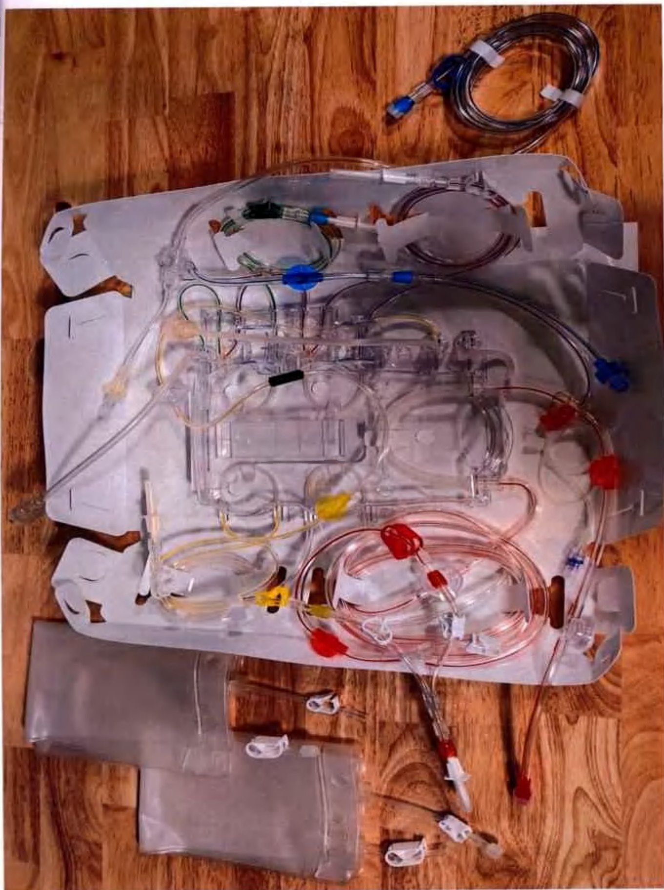
Рисунок 5 - Комплект магистралей с дренажным мешком NOVADIAL, в раскрытом виде
