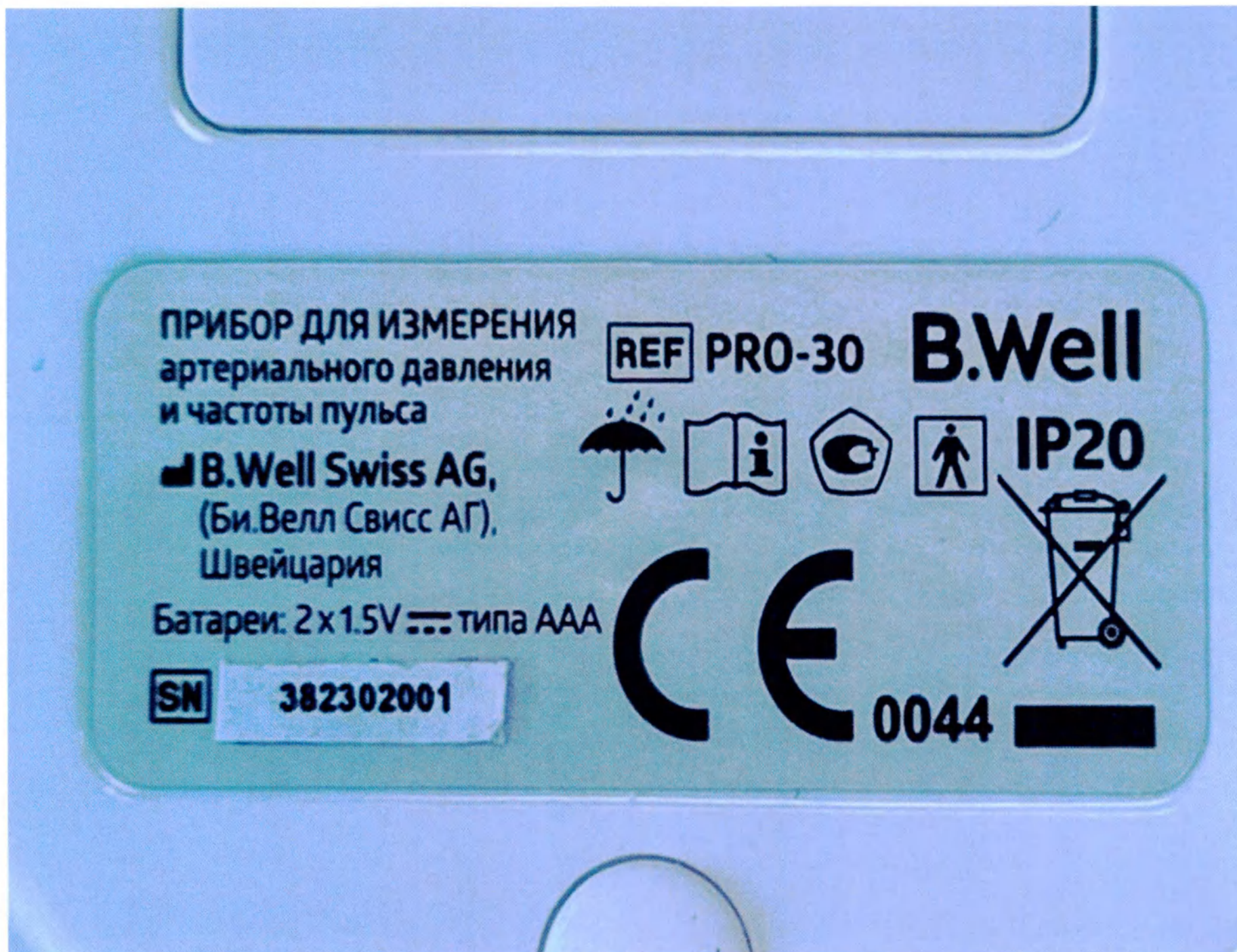
Рис. 11 Этикетка модели PRO-30
