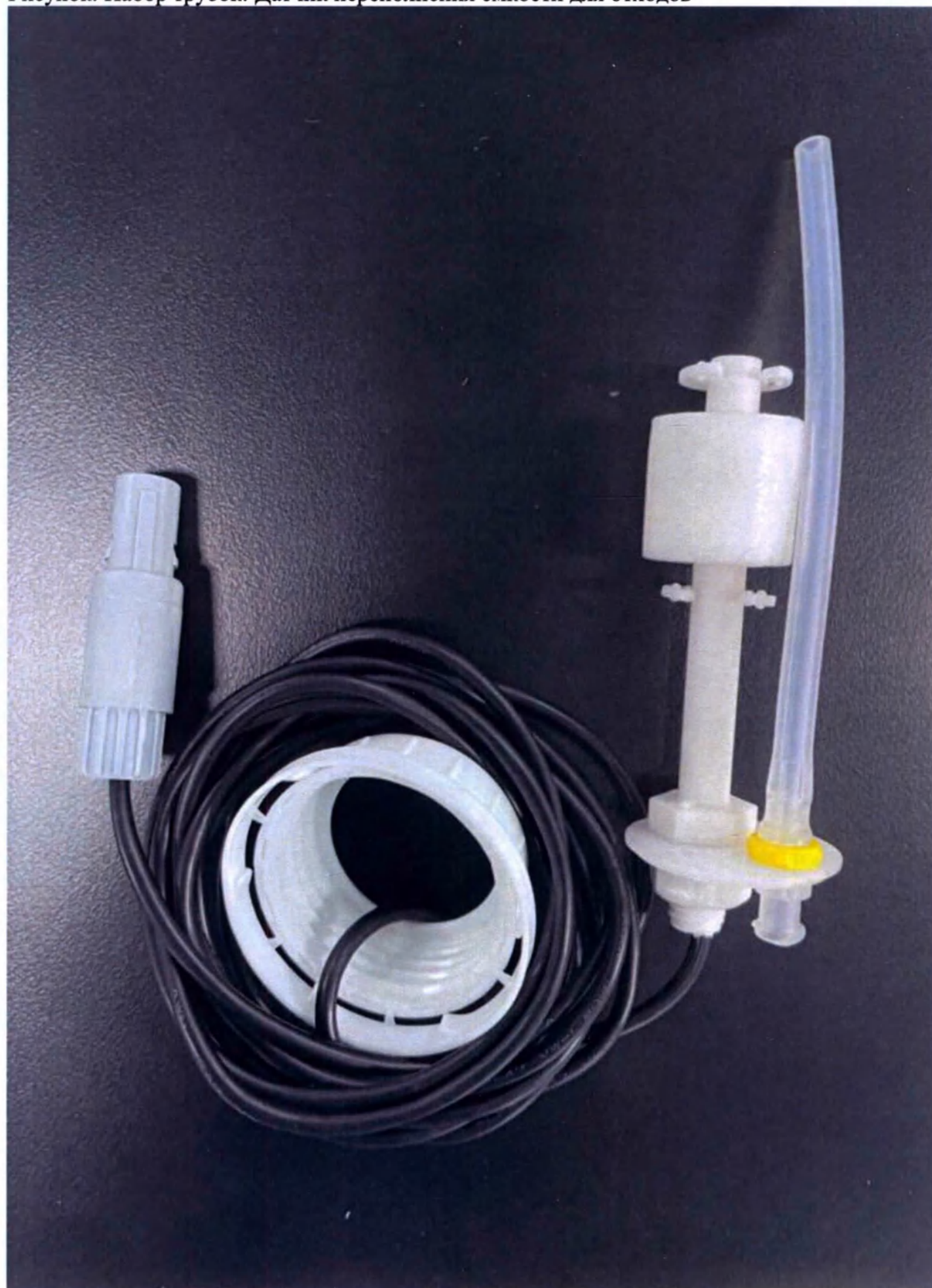
Рисунок. Набор трубок: Датчик переполнения емкости для отходов
