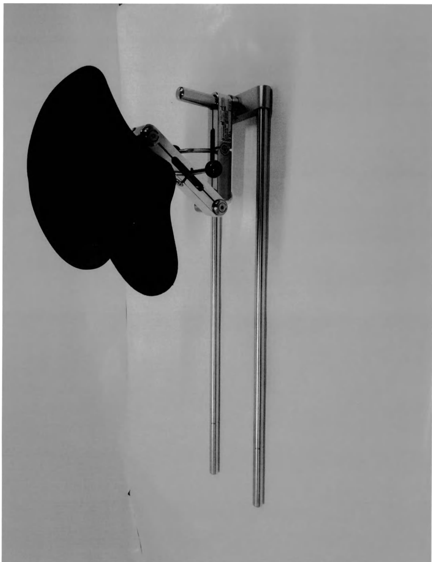
Опора для головы специальная для спинной секции для артроскопии плечевого сустава
