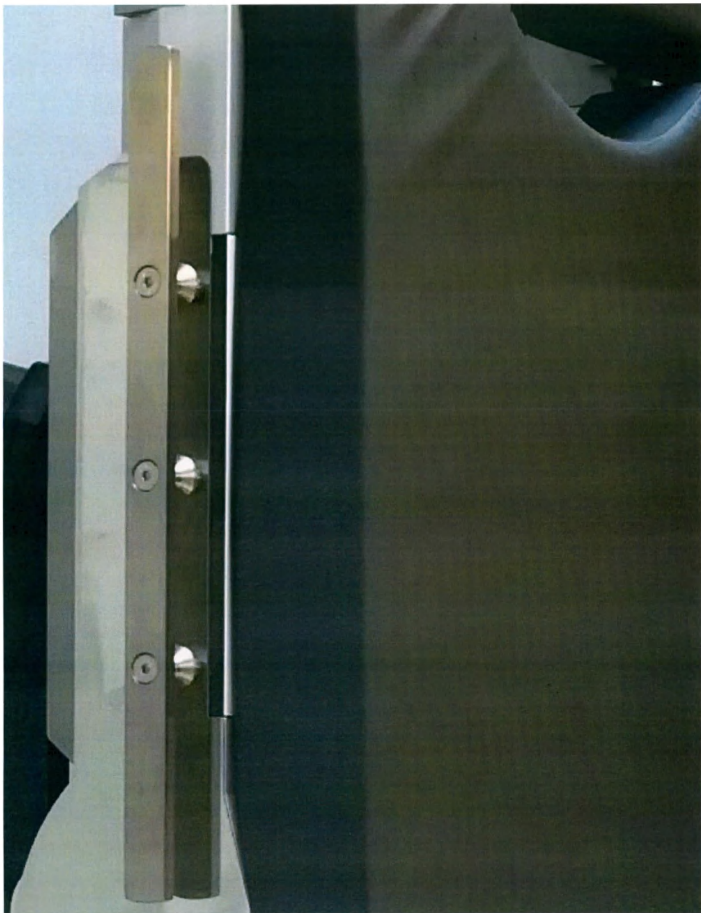
Пластины для крепления комплектующих к секциям стола
