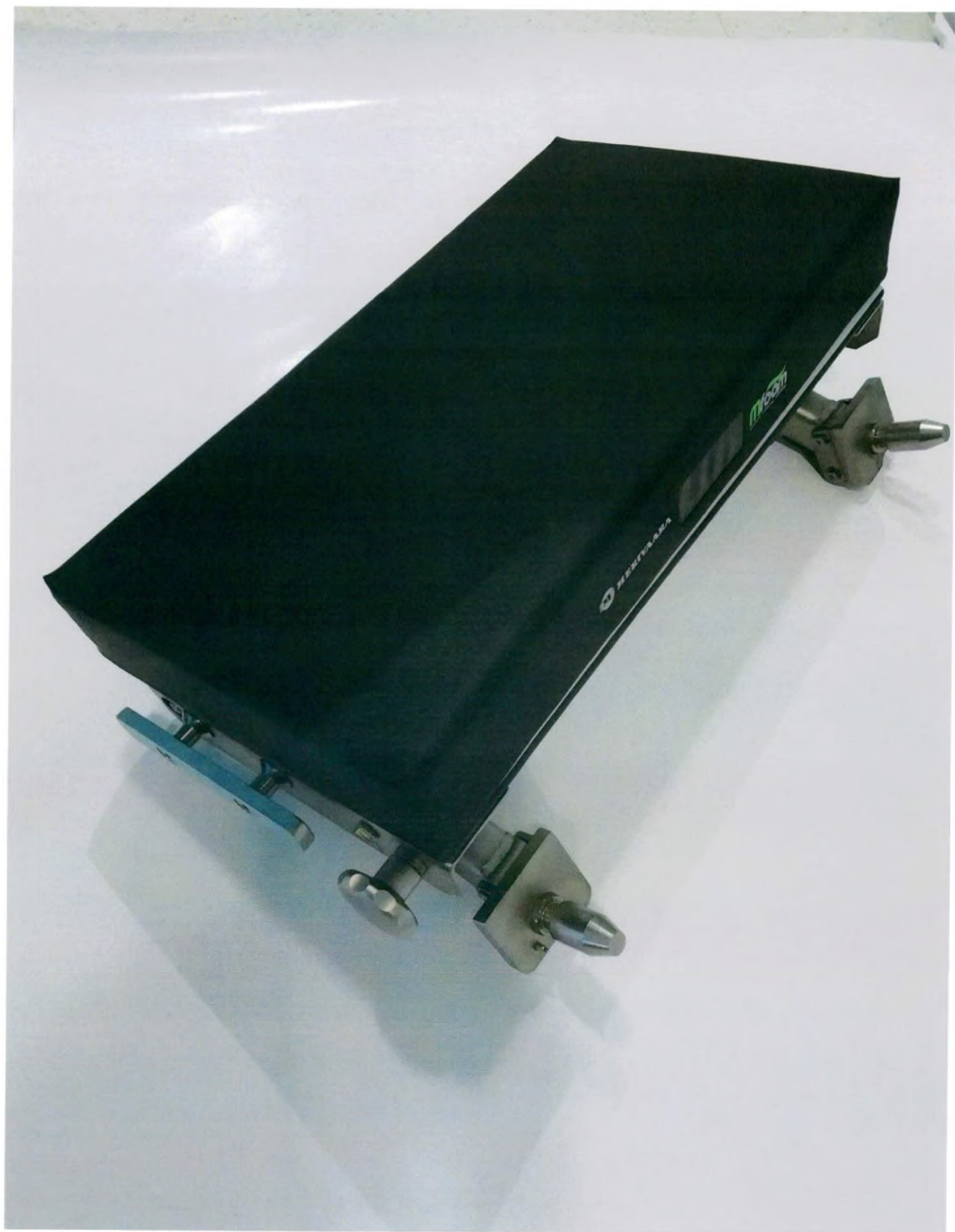
Опора для головы, регулируемая 3-мя газовыми пружинами, с двойной артикуляцией
