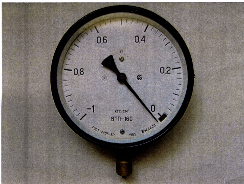
21. Вакуумметр
