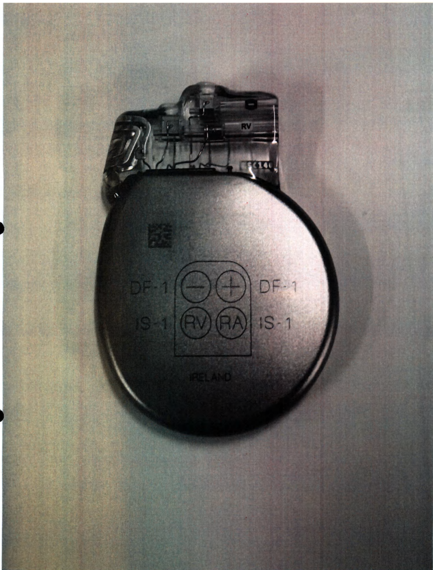
Фото 42. INOGEN MINI ICD DR модель D013. Общий вид.
