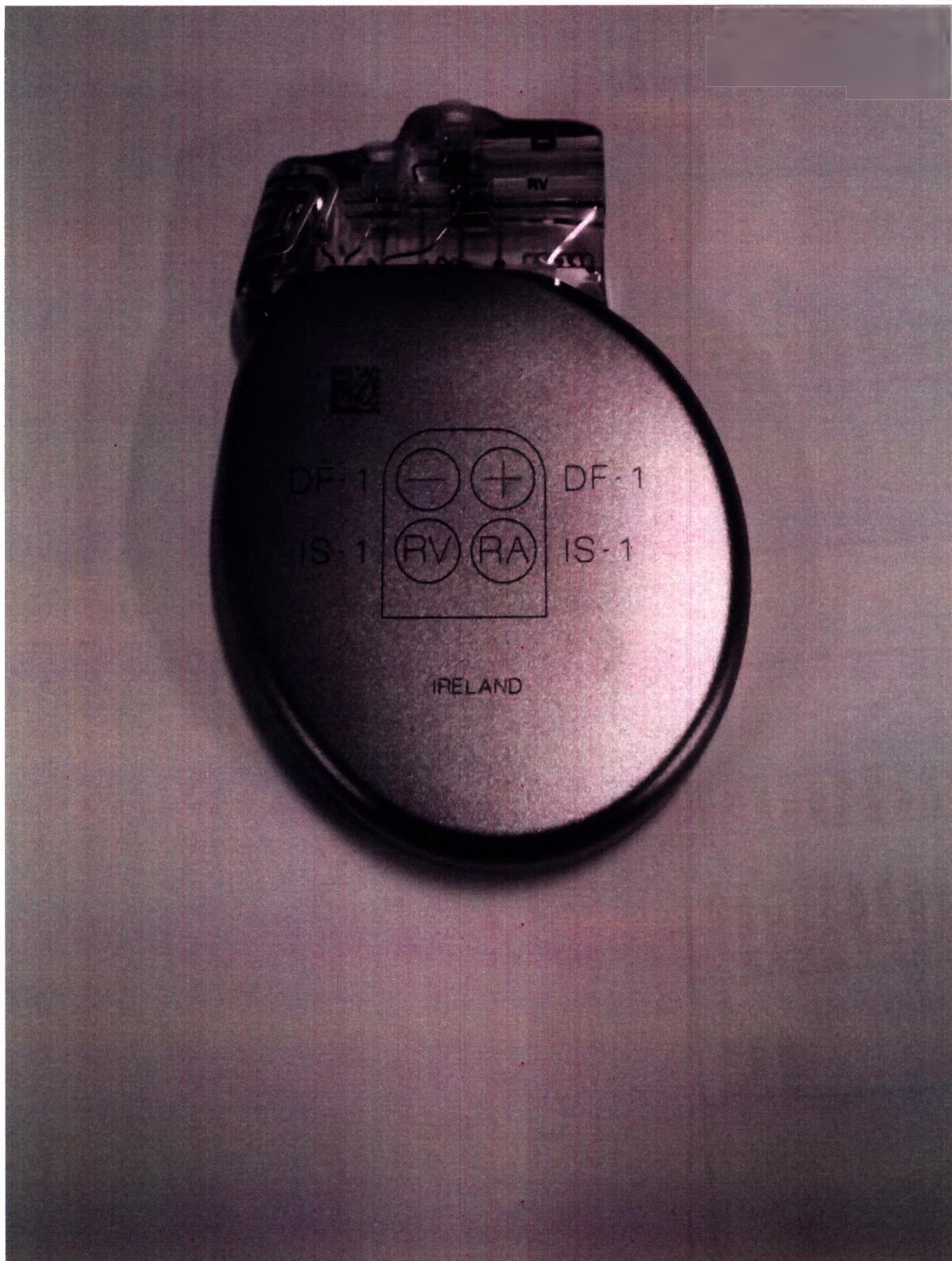
Фото 40. INOGEN EL ICD модель D141. Общий вид.
