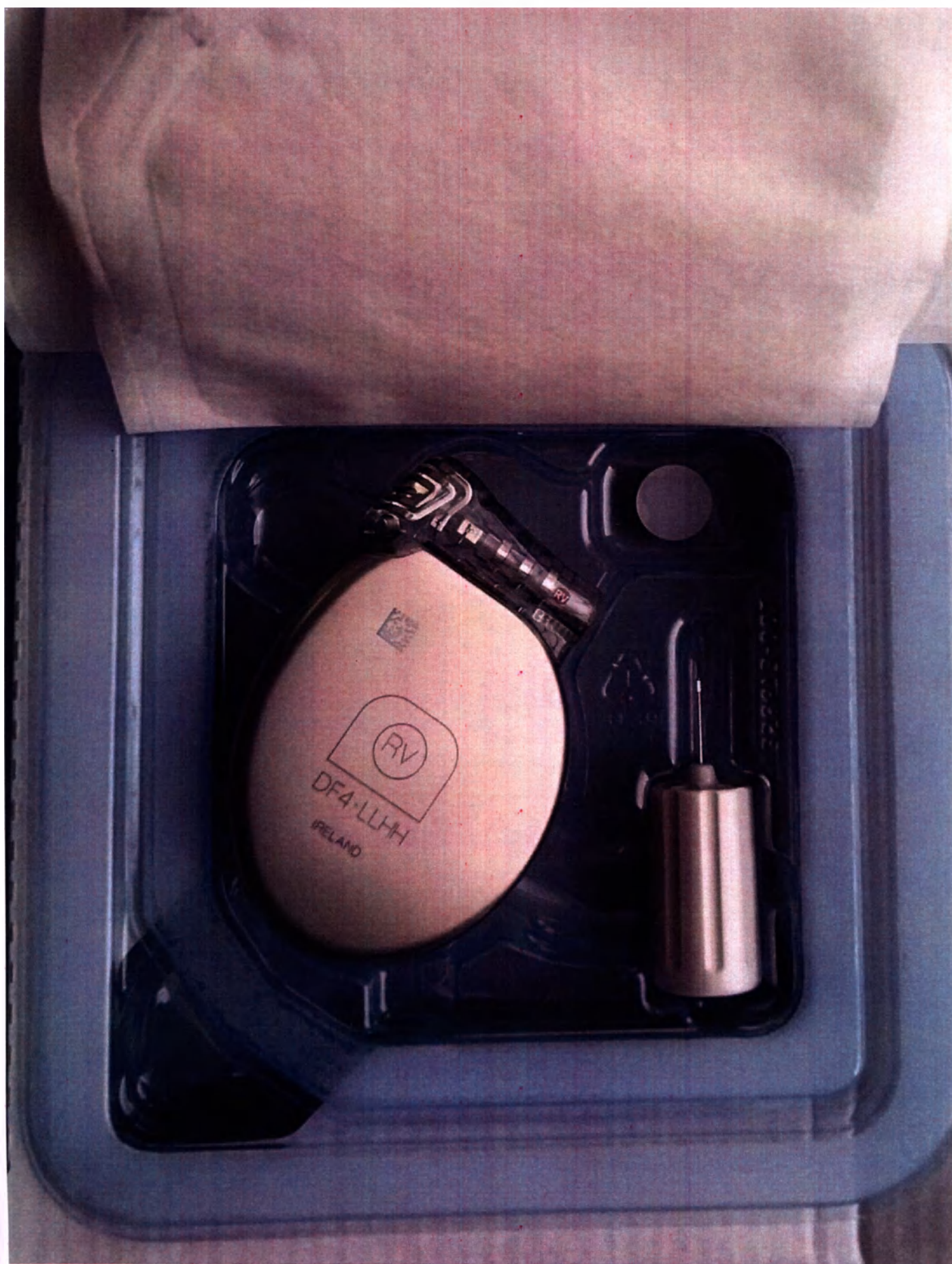
Фото 30. INOGEN EL ICD VR (MRI) модель D140. Общий вид.
