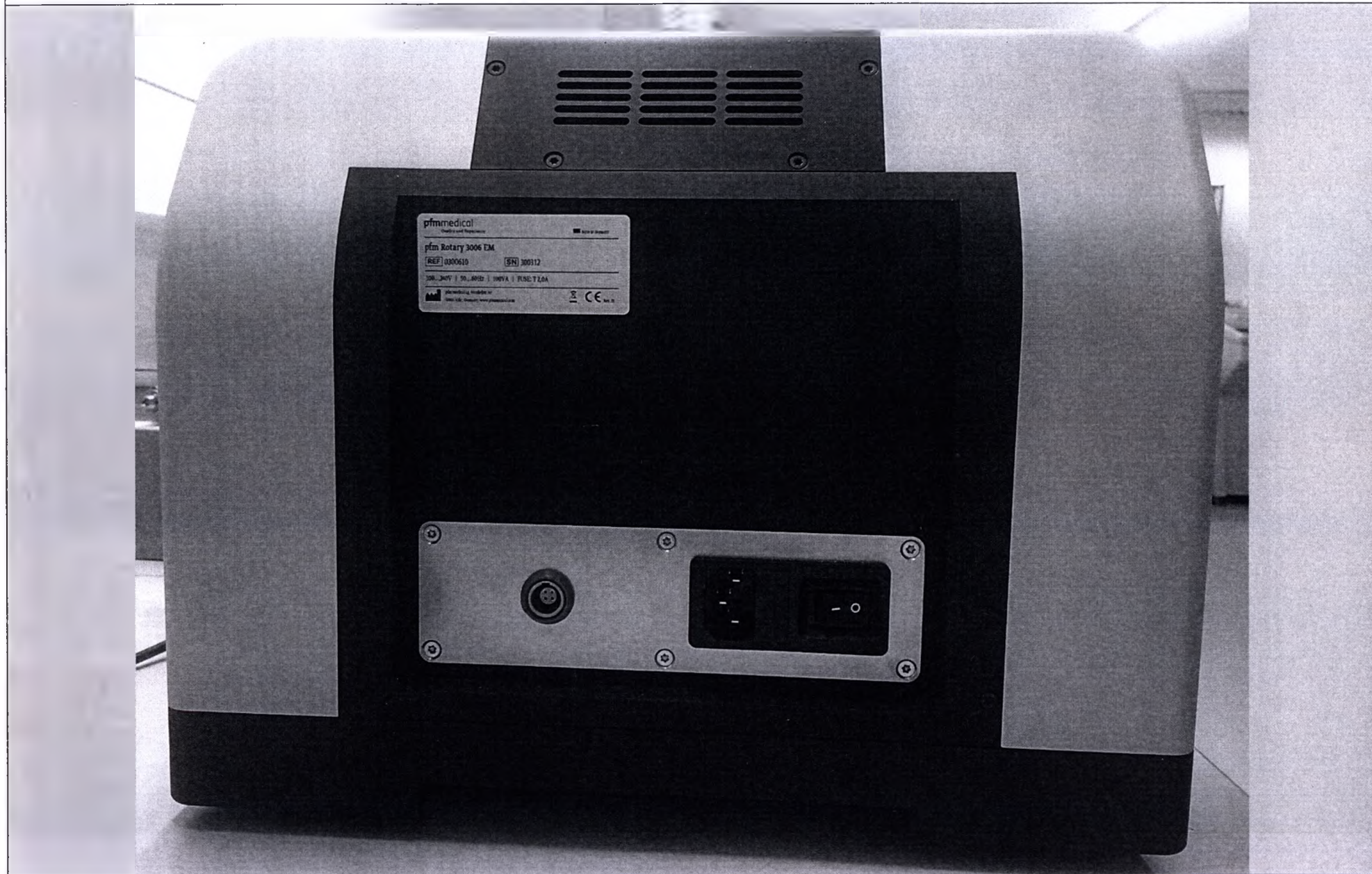
Блок микротомы основной (вид сзади)
