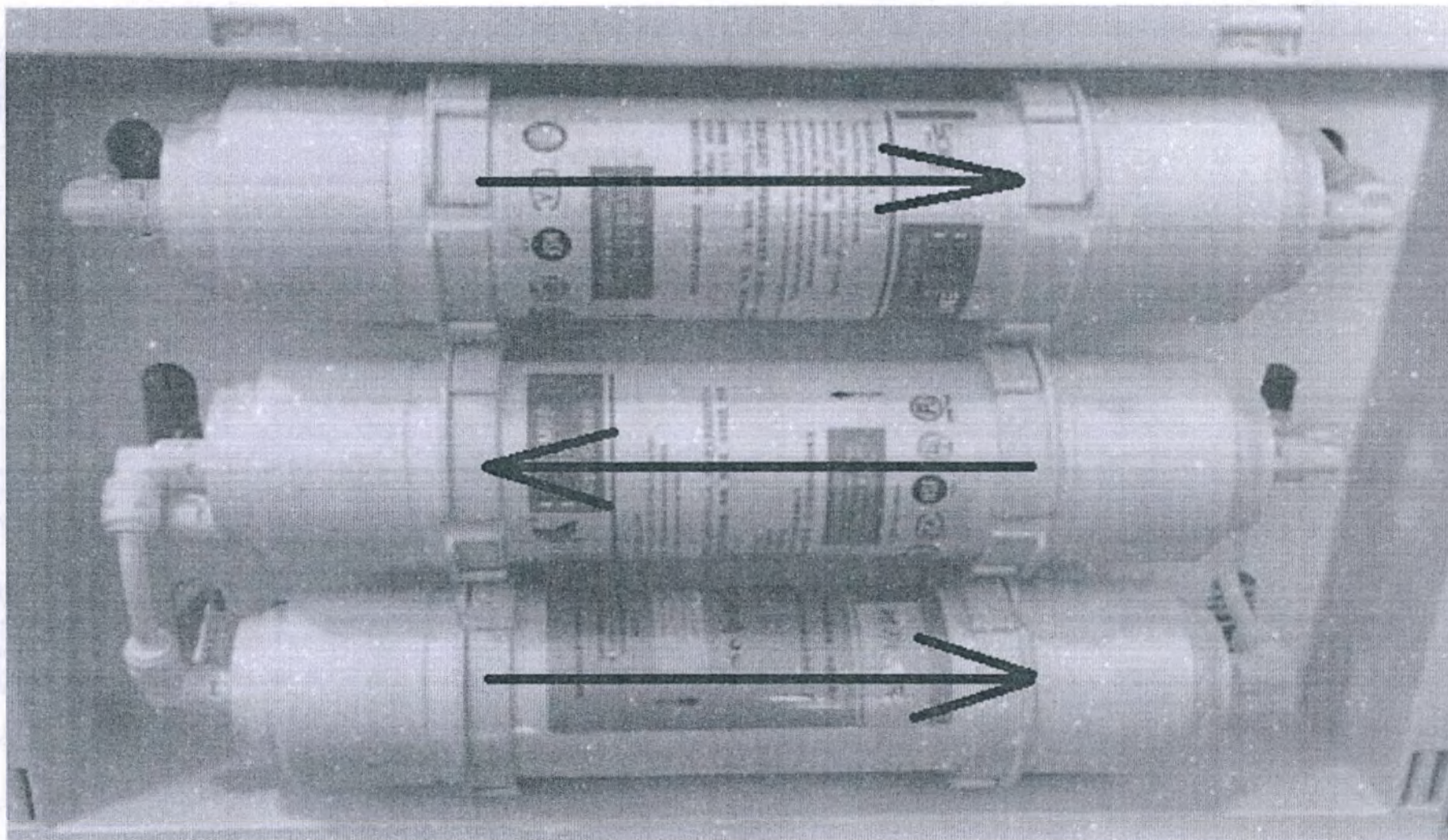
Фильтры для устройства очистки воды RW1 (сверху вниз): I (фильтр механической очистки), III (фильтр деионизации), II (фильтр обратного осмоса)
