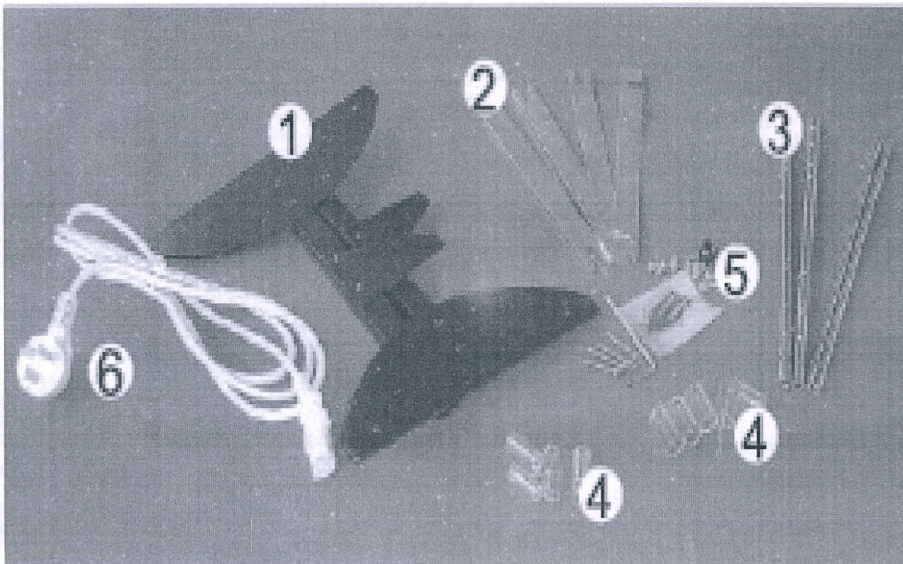
Принадлежности и комплектующие SEAL F300: 1. Опора; 2. Перегородки; 3. Рулонодержатель; 4. Пластиковые насадки для рулонодержателей; 5. Рукоятка резака; 6. Кабель питания
