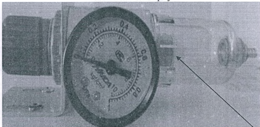
Клапан регулирования давления с манометром + воздушный фильтр
