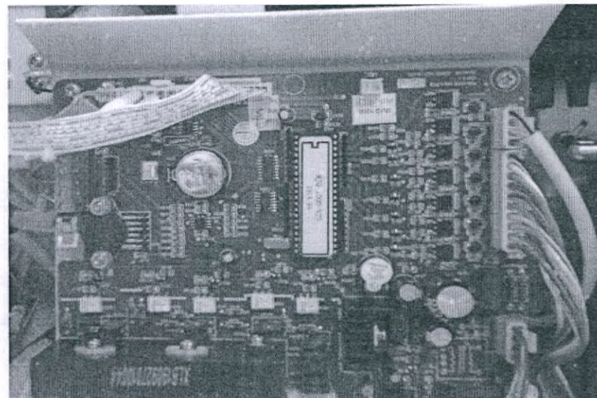
Плата управления
