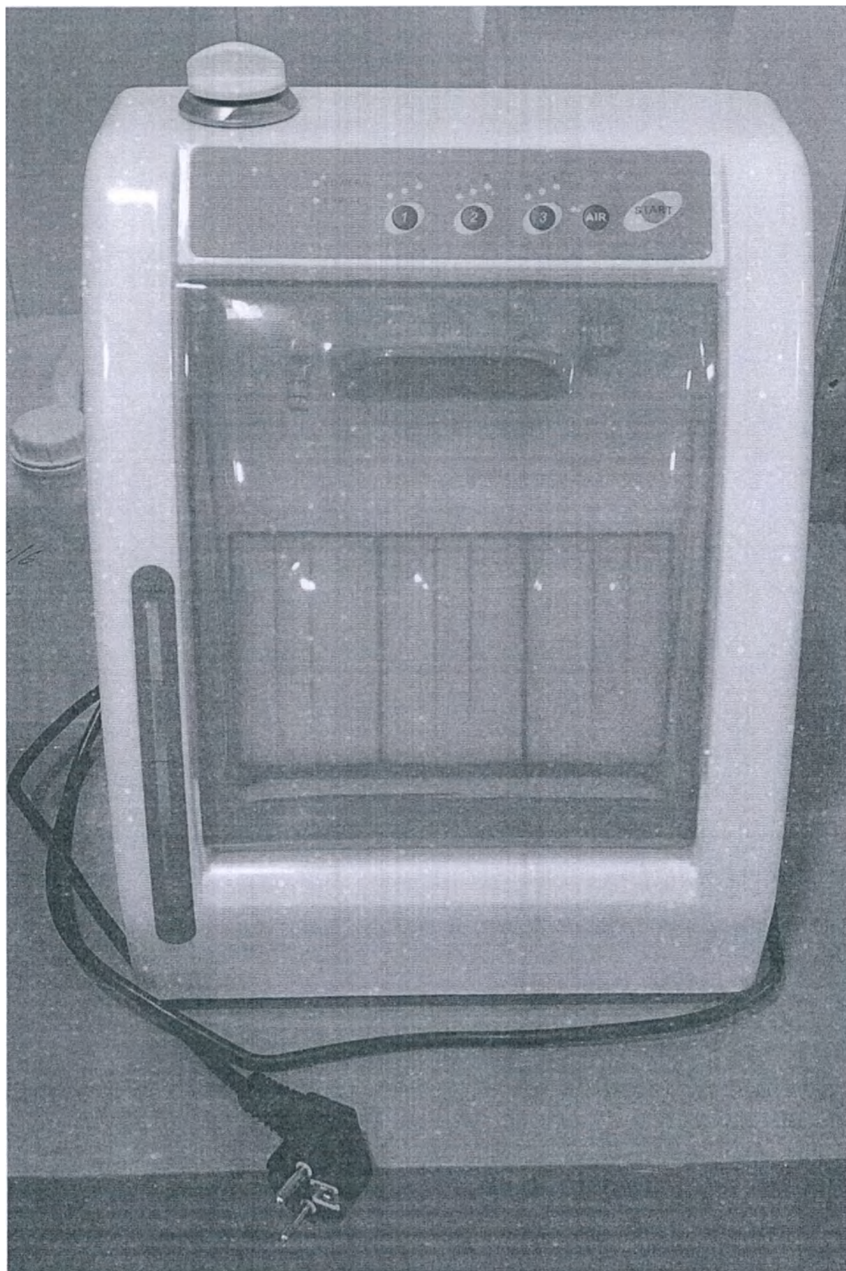
Устройство для смазки наконечников LUB-900B + кабель питания
