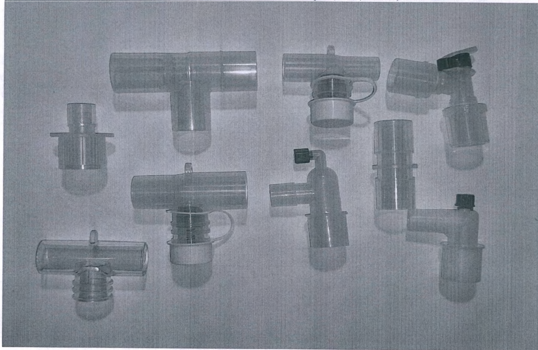
26. Держатели для масок (длиной 440 мм и 700 мм), производитель "ЭйчСинер Ко., Лтд.", Тайвань, РУ № ФСЗ2012/11566
