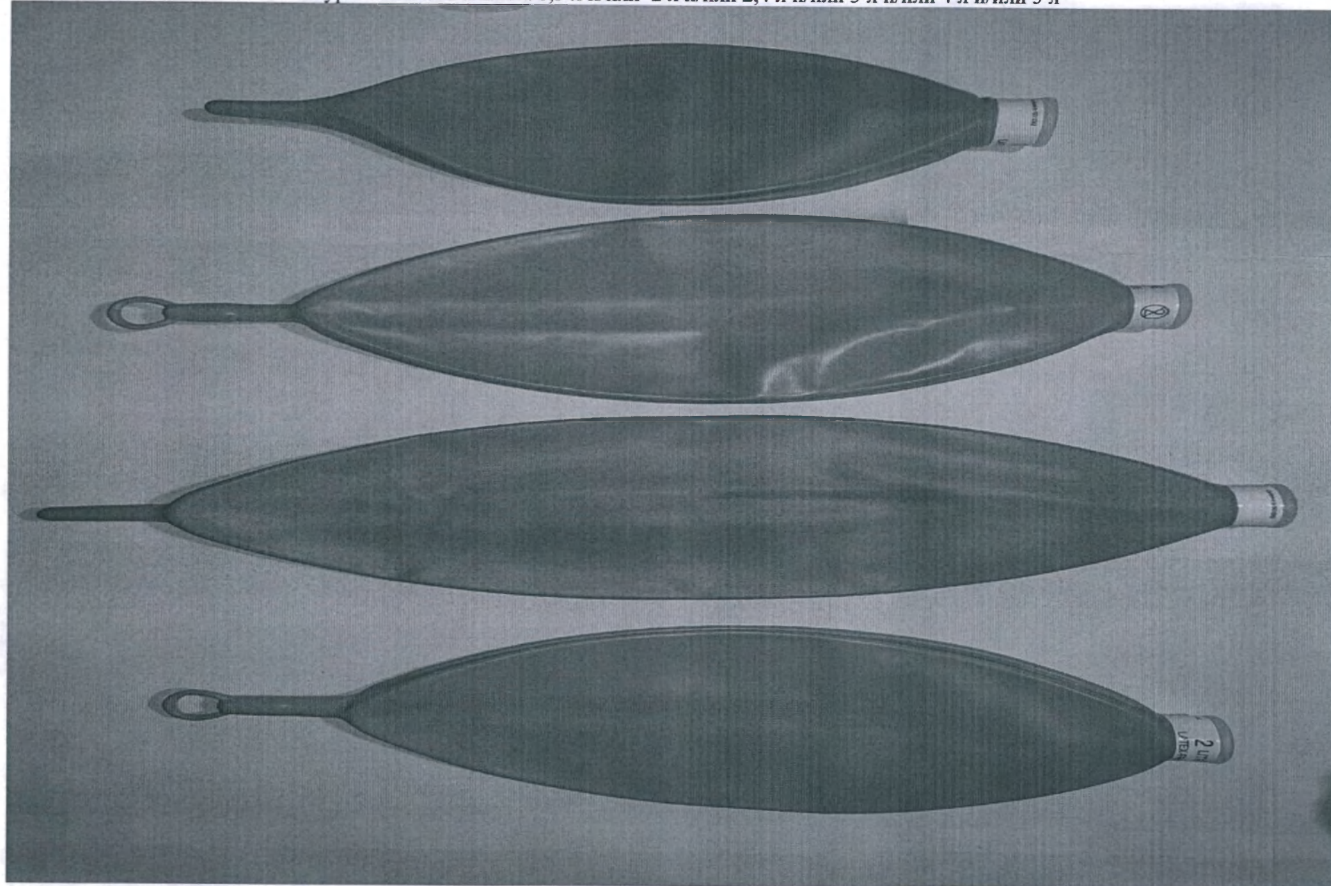
9. Мешок для дыхательного контура с петлей 1 л и/или 1,3 л и/или 2 л и/или 2,4 л и/или 3 л и/или 4 л и/или 5 л
