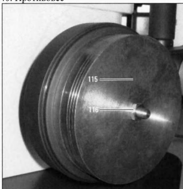
40. Противовес
