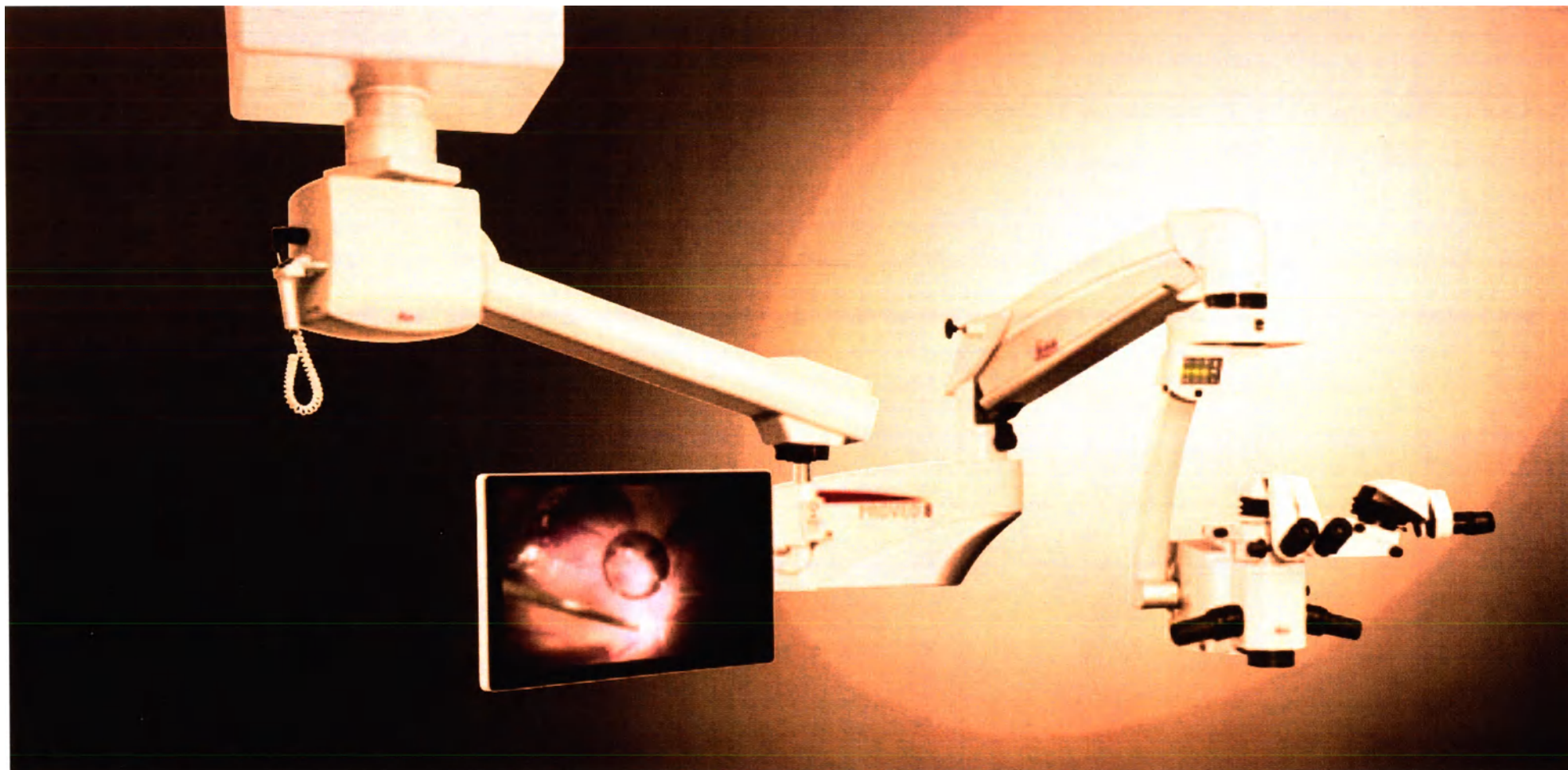
Рисунок 2 –Штатив потолочный.
