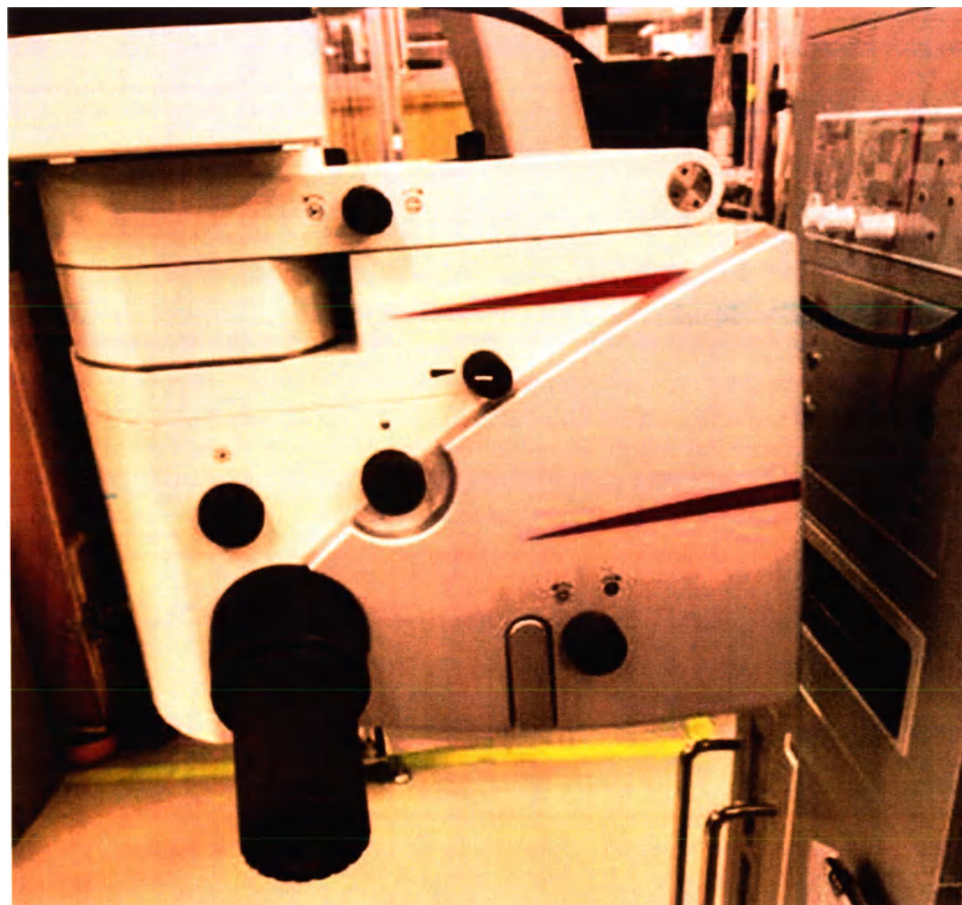
Рисунок 4 – Блок микроскопа оптический с ХУ модулем, механизмом фокусировки и наклона.
