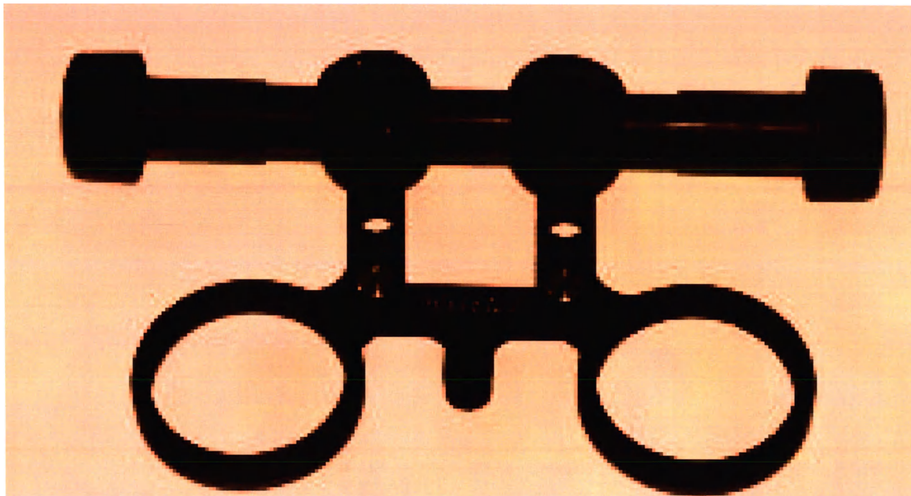
Рисунок 16 – Модуль установки межзрачкового расстояния.
