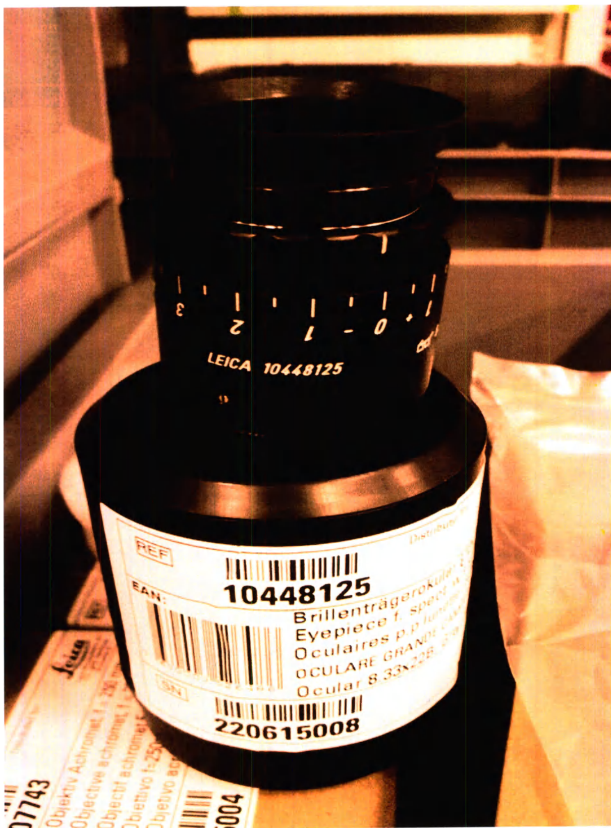
Рисунок 33 – Окуляр подстраиваемый 8,33х/21В.
