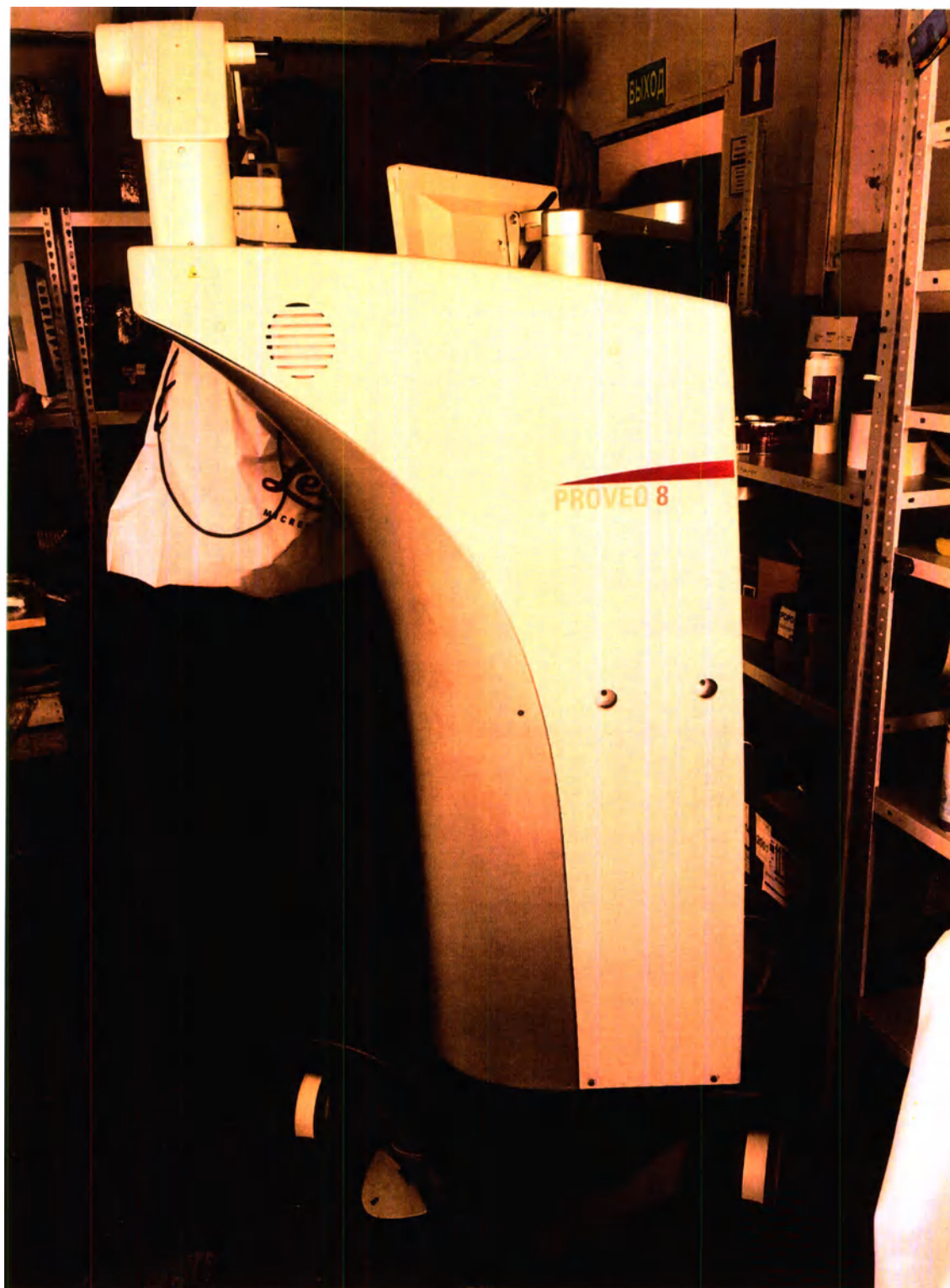
Рисунок 99 – Штатив напольный.
