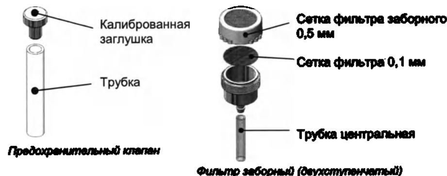
Рис.23 Предохранительный клапан и Фильтр заборный (двухступенчатый)
