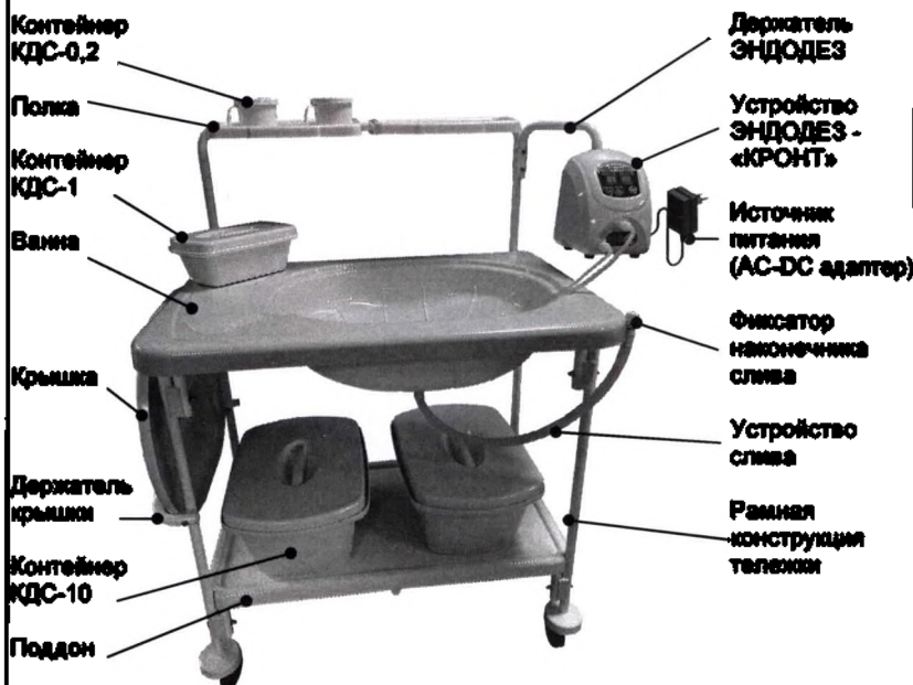
Рис.3 Установка устройства слива на ванну установки
