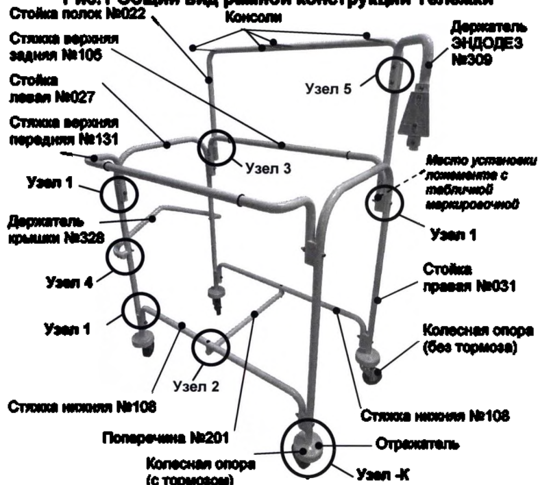
Рис.1 Общий вид рамной конструкции Тележки
