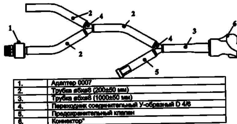
Рис.19 Внешний вид магистрали напорной №2
