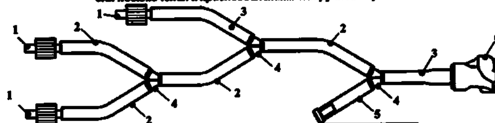
Рис.21/1 Внешний вид манометра напорной №1 (с тремя наконечниками luer-lock) для подключения к приспособлению для ручной обработки
