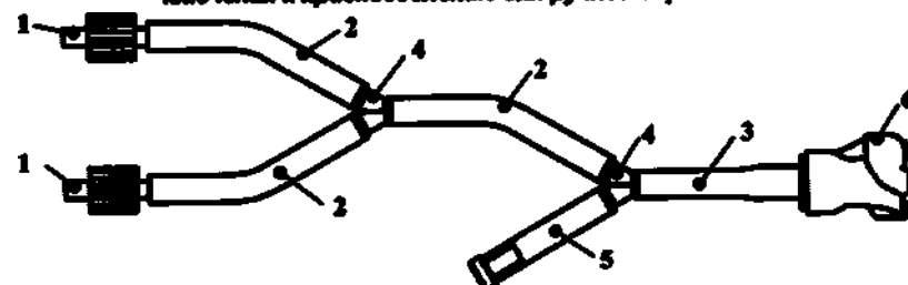
Рис.20 Внешний вид манометра напорной №2 (с двумя наконечниками luer-lock) для подключения к приспособлению для ручной обработки
