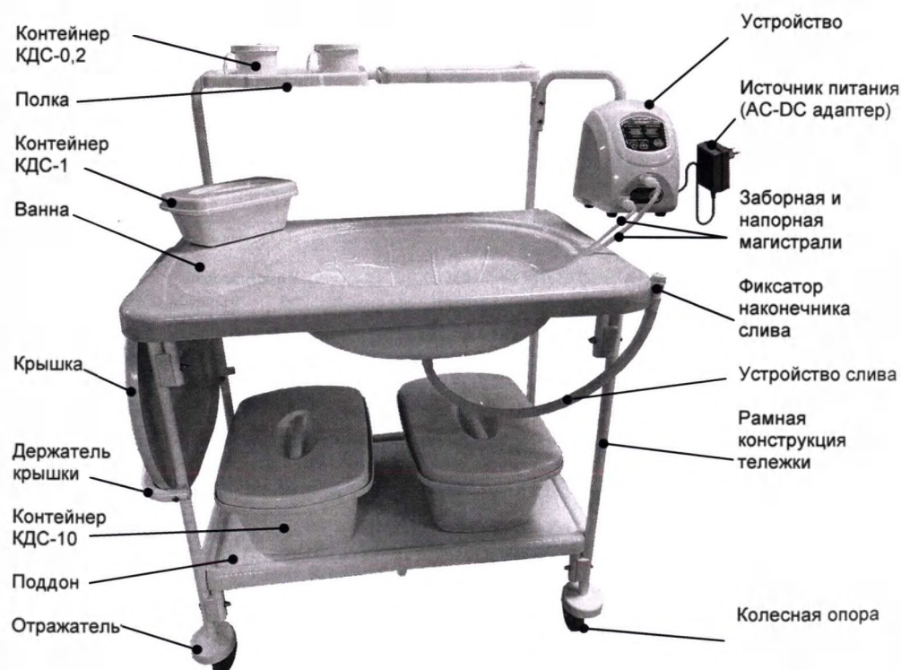
Рис.1 Внешний вид Установки
