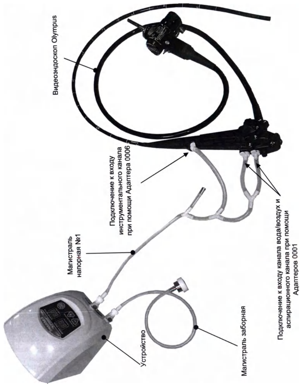
Рис. 24 Вариант подключения магистрали напорной №1 на ПРИМЕРЕ эндоскопа Olympus (для обработки Устройством каналов: аспирационный, инструментальный, вода/воздух)
