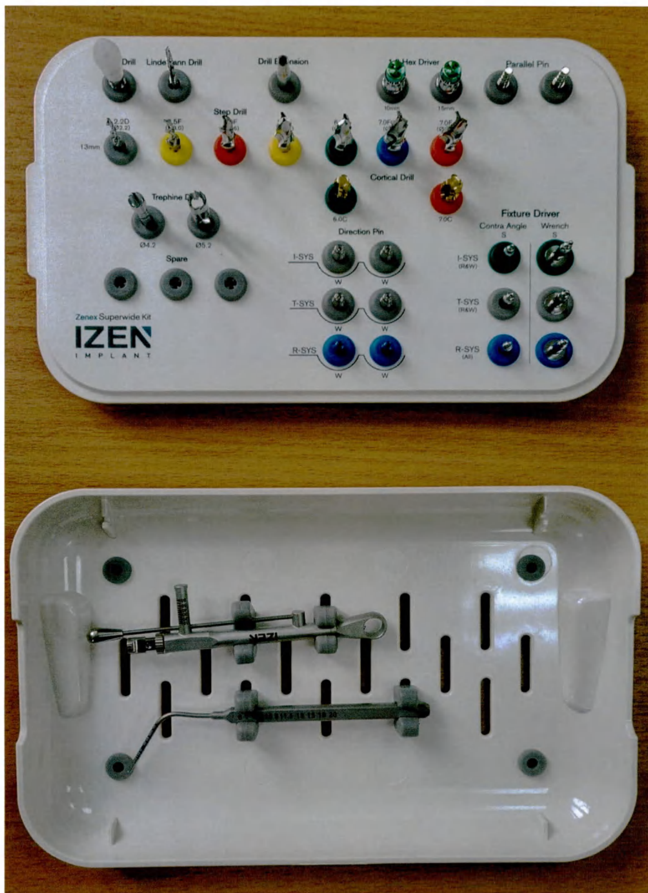
Рис. 3 Набор инструментов стоматологических хирургических ZENEX SUPERWIDE KIT (ZENSWKIT) – общий вид
