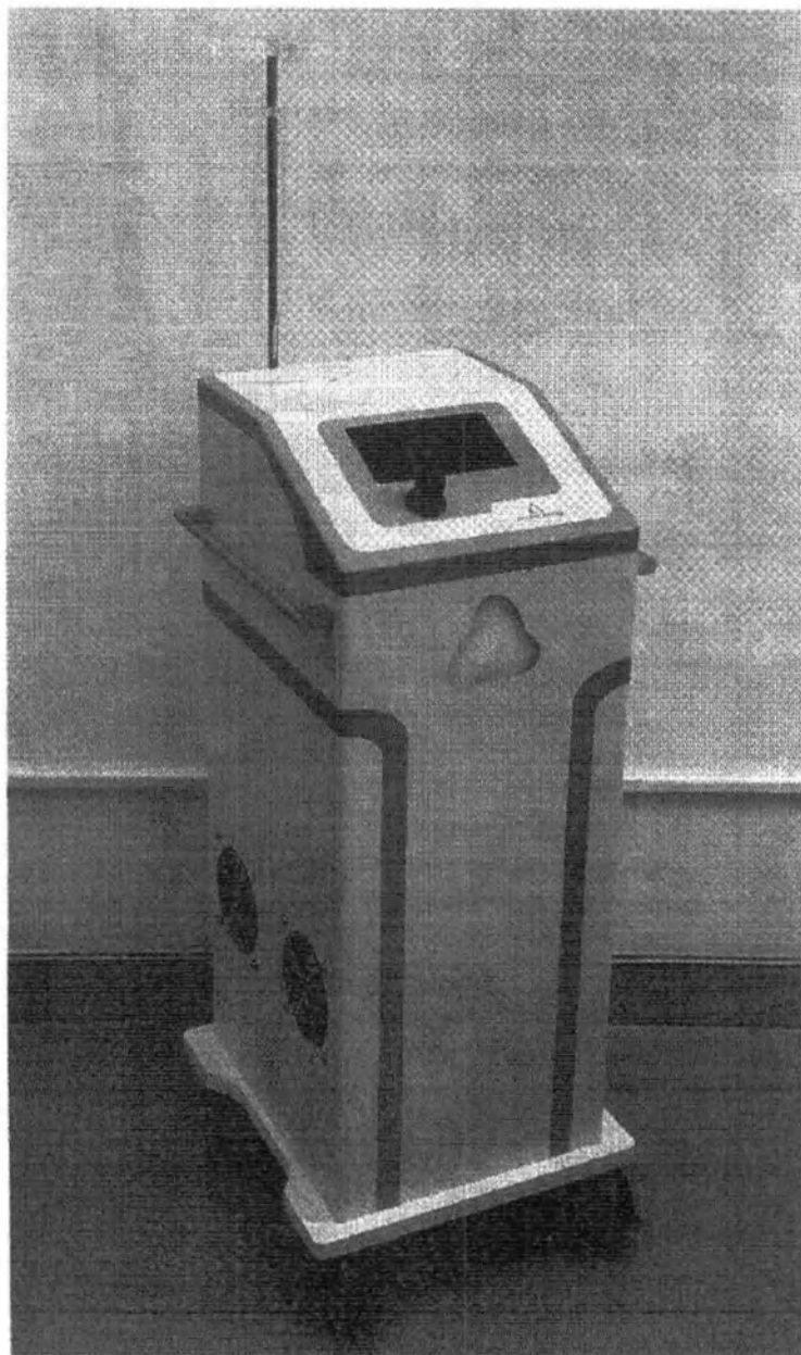
Рисунок 6 – Аппарат косметологический для струйной газожидкостной обработки кожи «АТИСМЕД PRO 7», общий вид.
