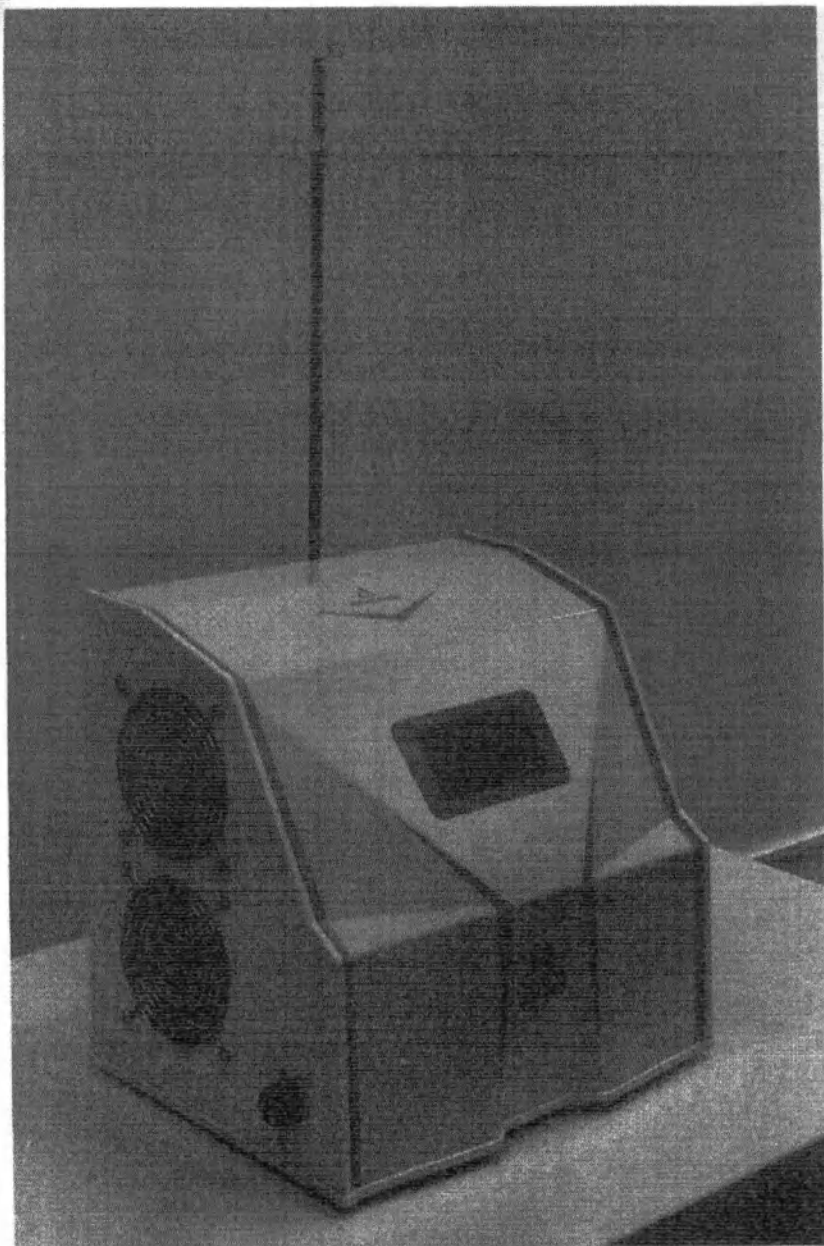
Рисунок 16 – Аппарат косметологический для струйной газожидкостной обработки кожи «АТИСМЕД PRO COMFORT PLUS», общий вид.
