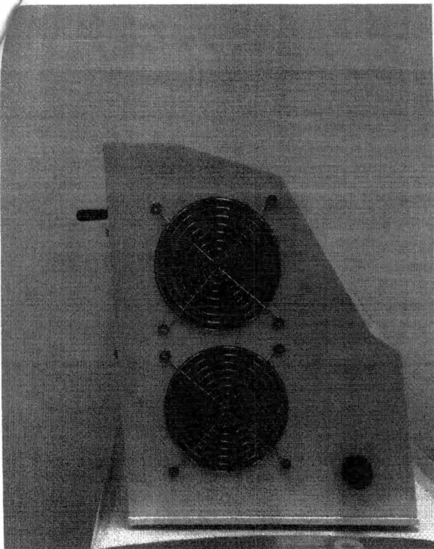
Рисунок 12 – Аппарат косметологический для струйной газожидкостной обработки кожи «АТИСМЕД PRO COMFORT», вид слева.
