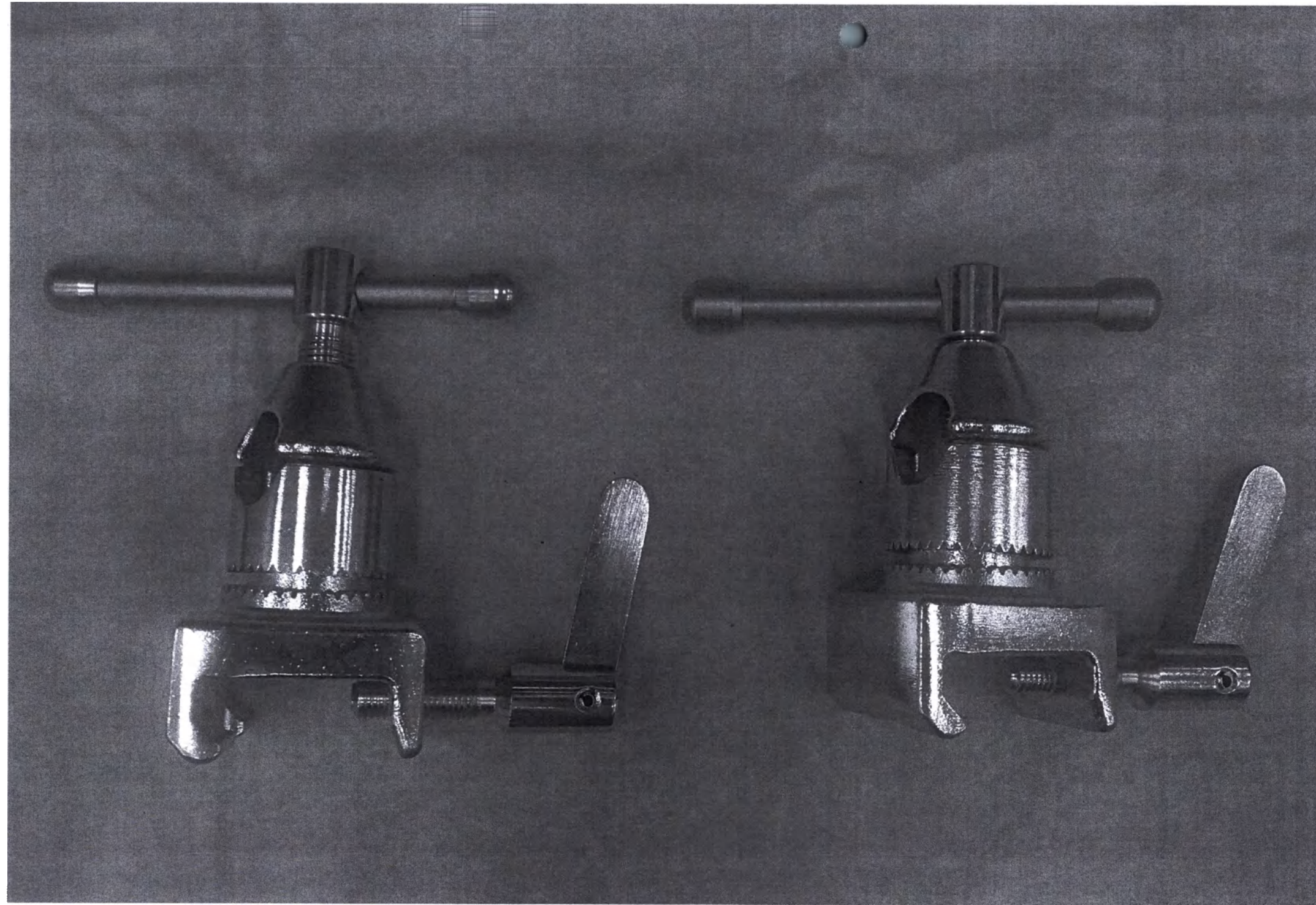
Рис. 19 – Фиксатор опоры для ноги (2 шт.)
