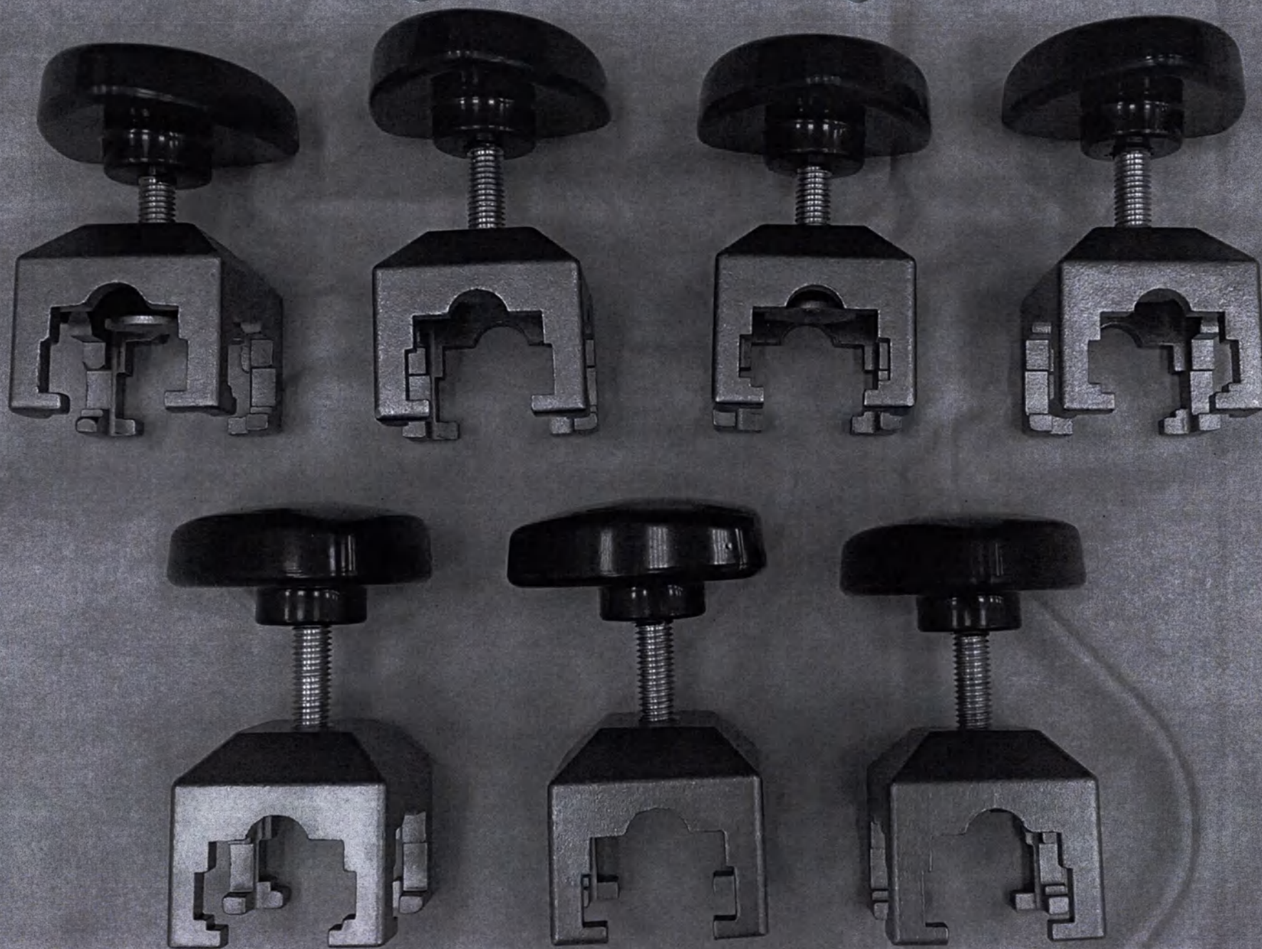
Рис. 63 – Фиксатор навесных элементов (7 шт.)
