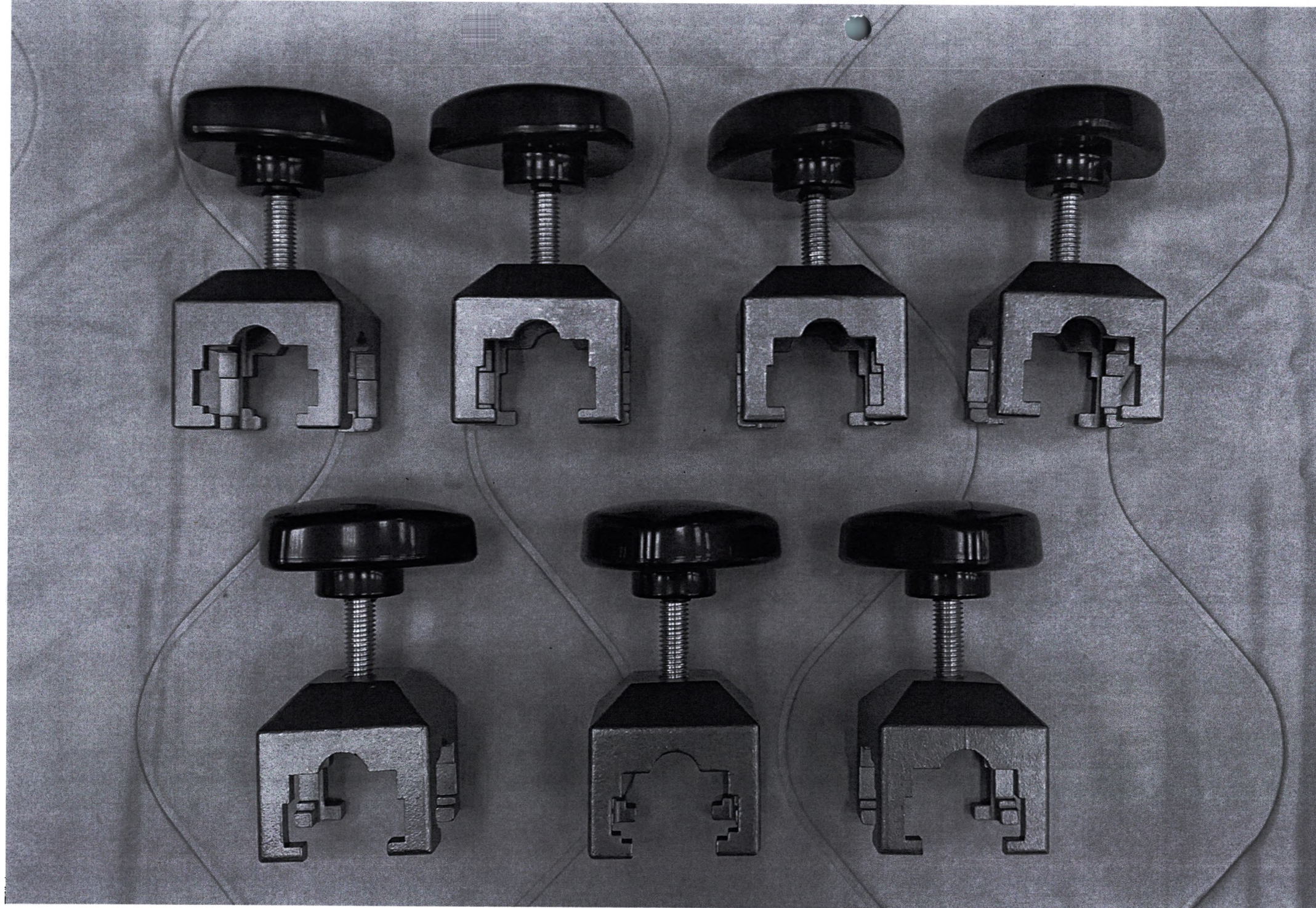
Рис. 49 – Фиксатор навесных элементов (7 шт.)
