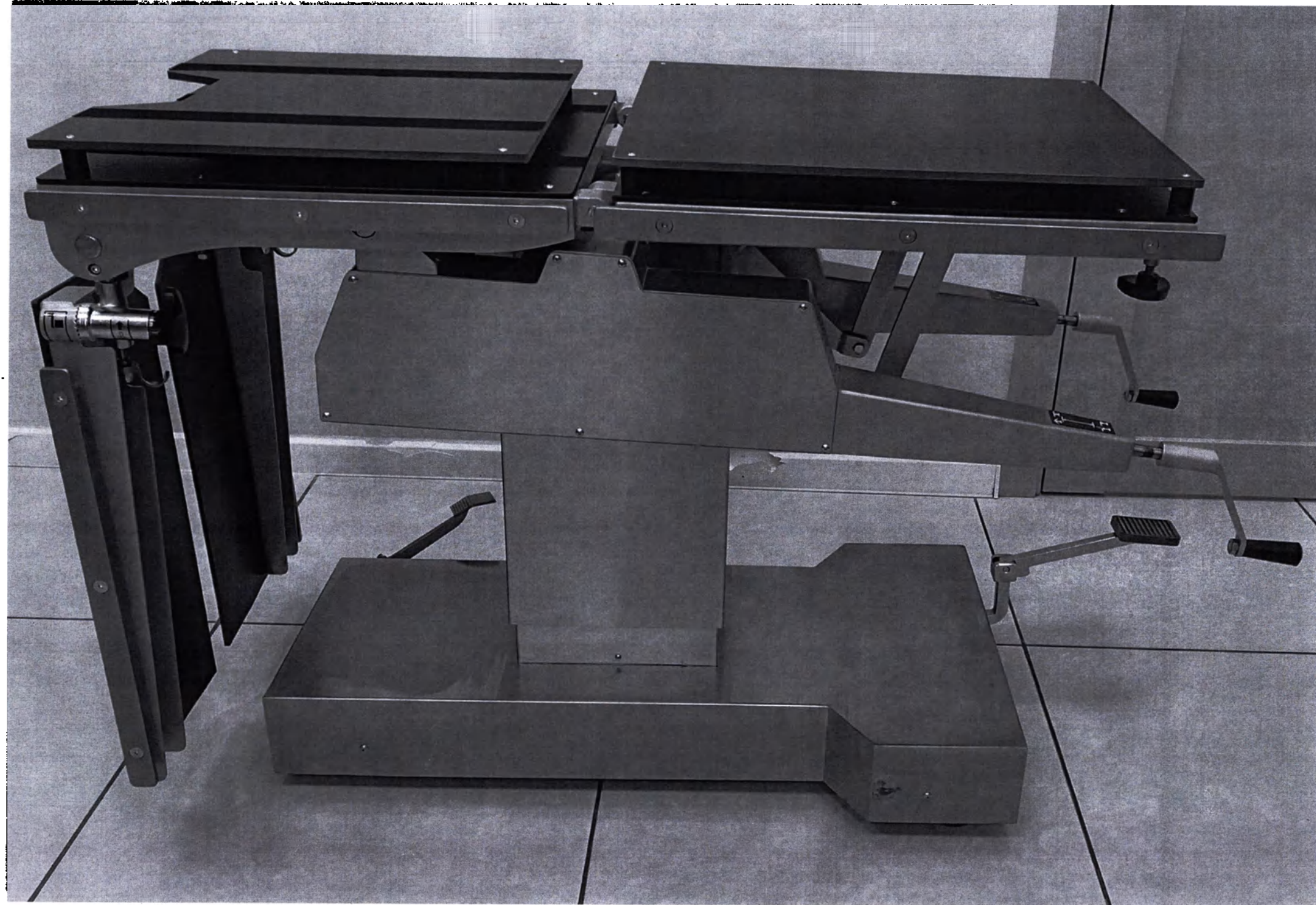
Рис. 2 – Стол (основание)
