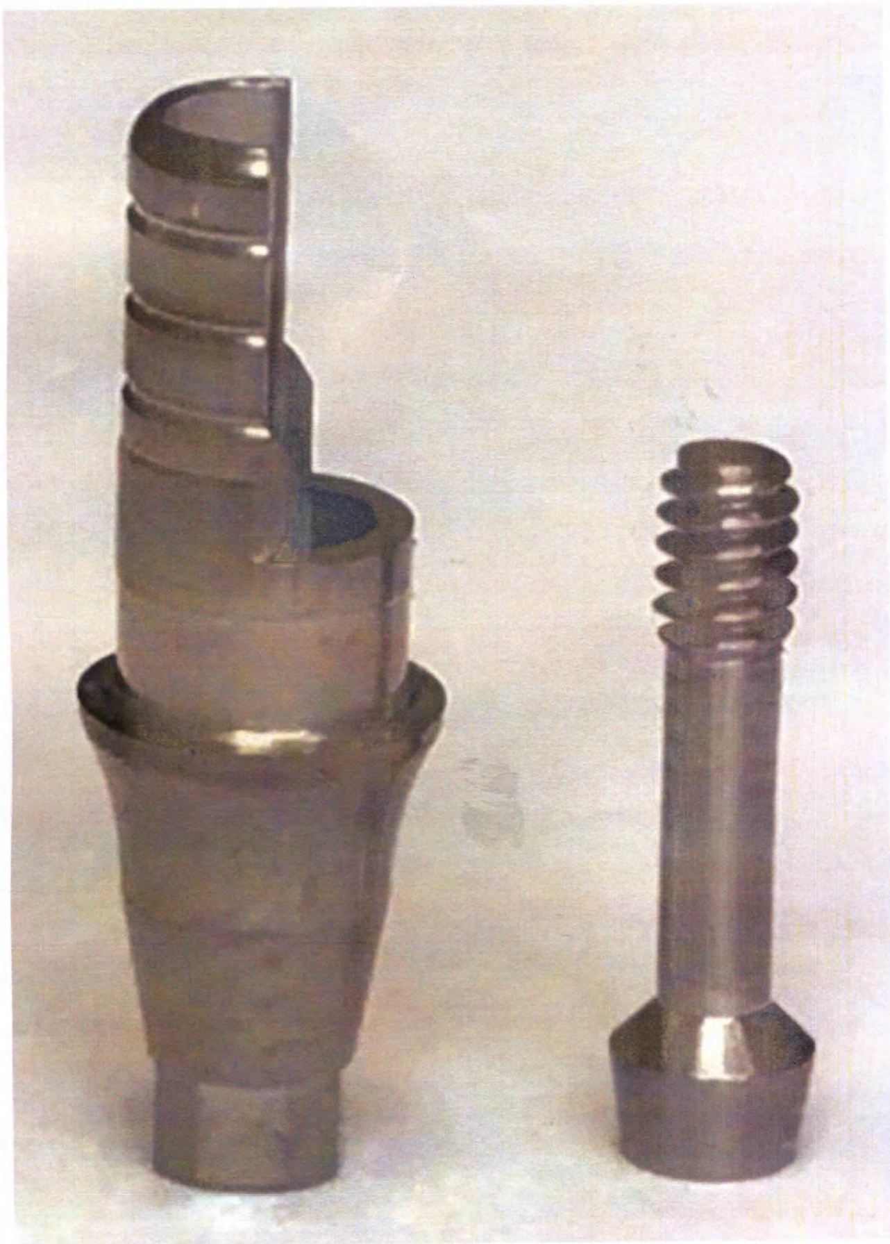
Рис. 3 Абатмент титановое основание ASC Flex, MICROCONE / QUATTROCONE, для коронки, платформа RI, десневая высота 2.5 мм, высота абатмента 3.5-6.5 мм, тип 1 / SF с винтом
