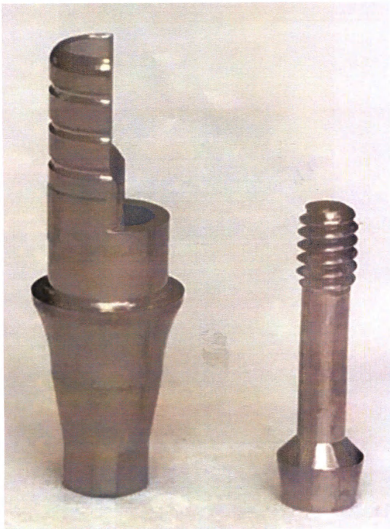
Рис. 4 Абатмент титановое основание ASC Flex, MICROCONE / QUATTROCONE, для коронки, платформа RI, десневая высота 2.5 мм, высота абатмента 3.5-4.5 мм, тип 2 / SC с винтом
