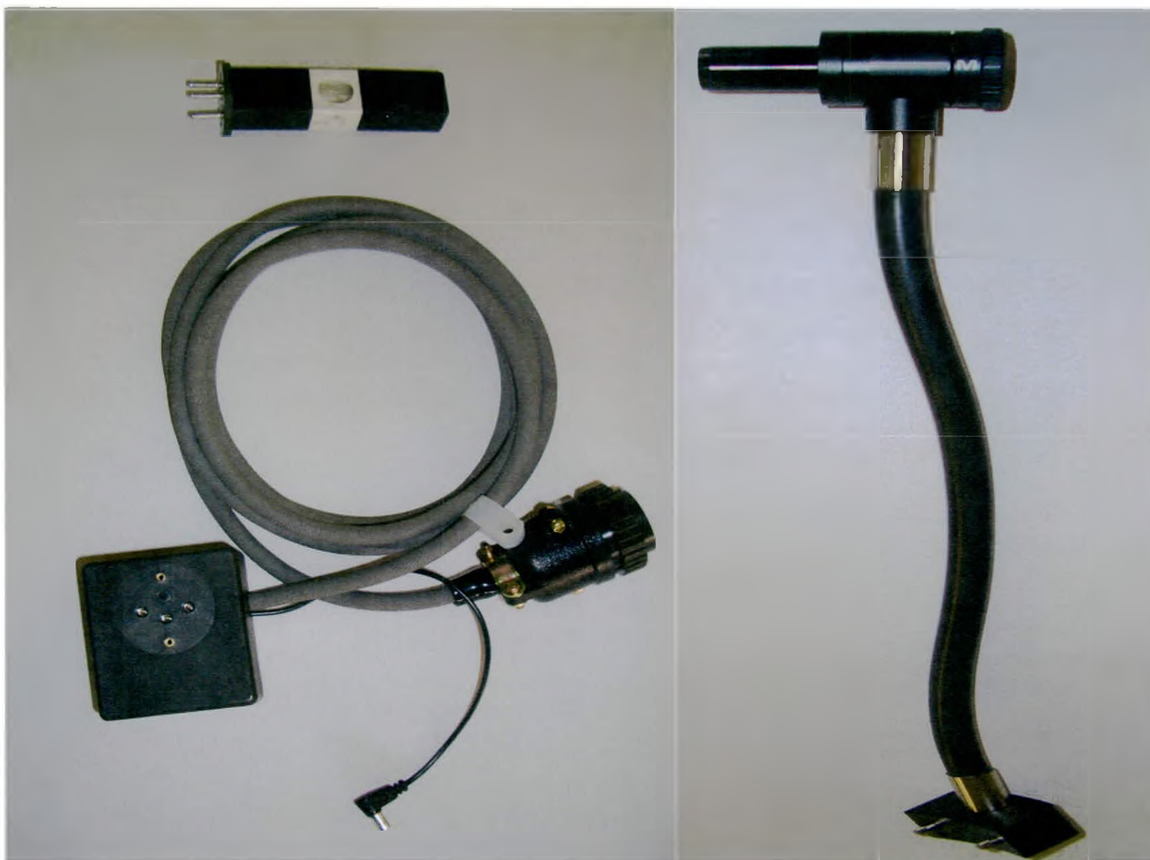
Устройство фонового освещения ( ламповый блок,волоконный световод,осветительная головка)
