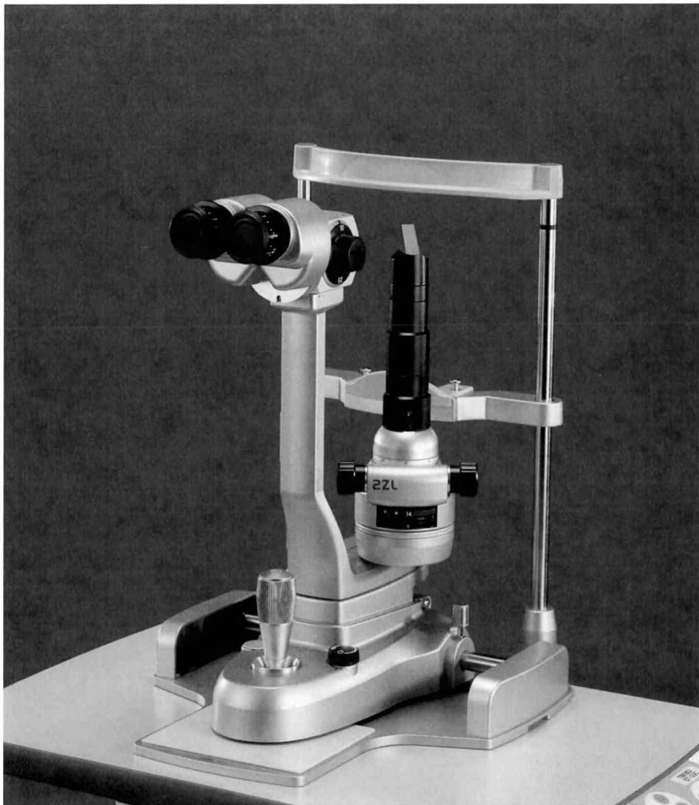
Щелевая лампа 2ZL Основной блок в сборе с лицевым упором
