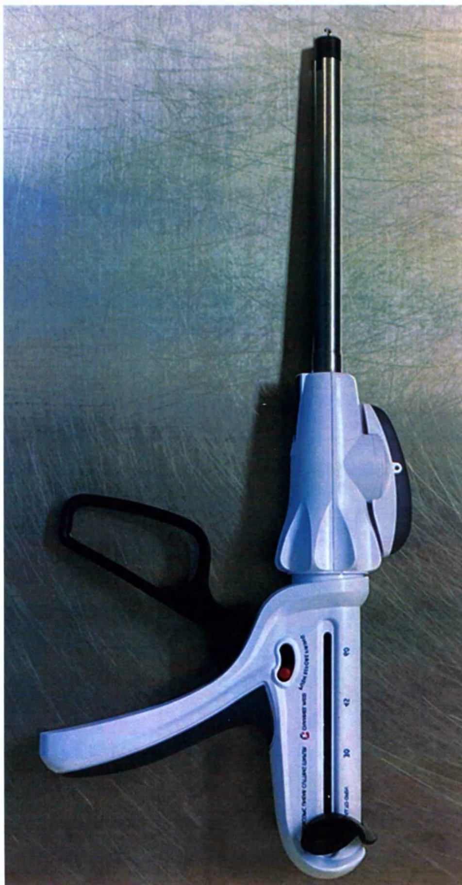
Внешний вид изделия в варианте исполнения с кодировкой CN-ED12 без учёта длины стержня (внешний вид изделия не отличается в зависимости от длины стержня)
