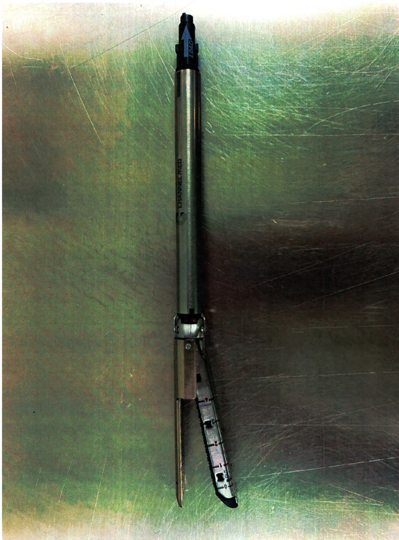
Внешний вид изделия в варианте исполнения CN-CCRE с кодом цвета G - чёрный, без учёта длины шва
