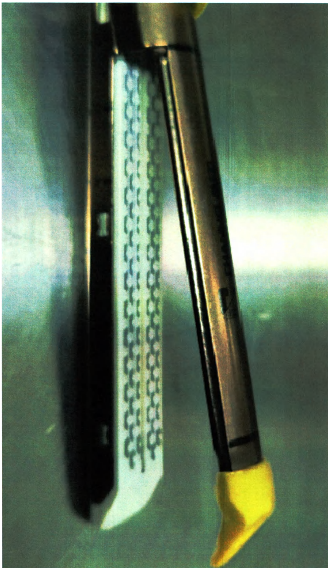
Увеличенное изображение сменного картриджа изделия в варианте исполнения CN-CCRC60 с кодом цвета W – белый, тип 1 (тип 2 выглядит идентично, только с жёлтым съёмным пластиковым наконечником)
