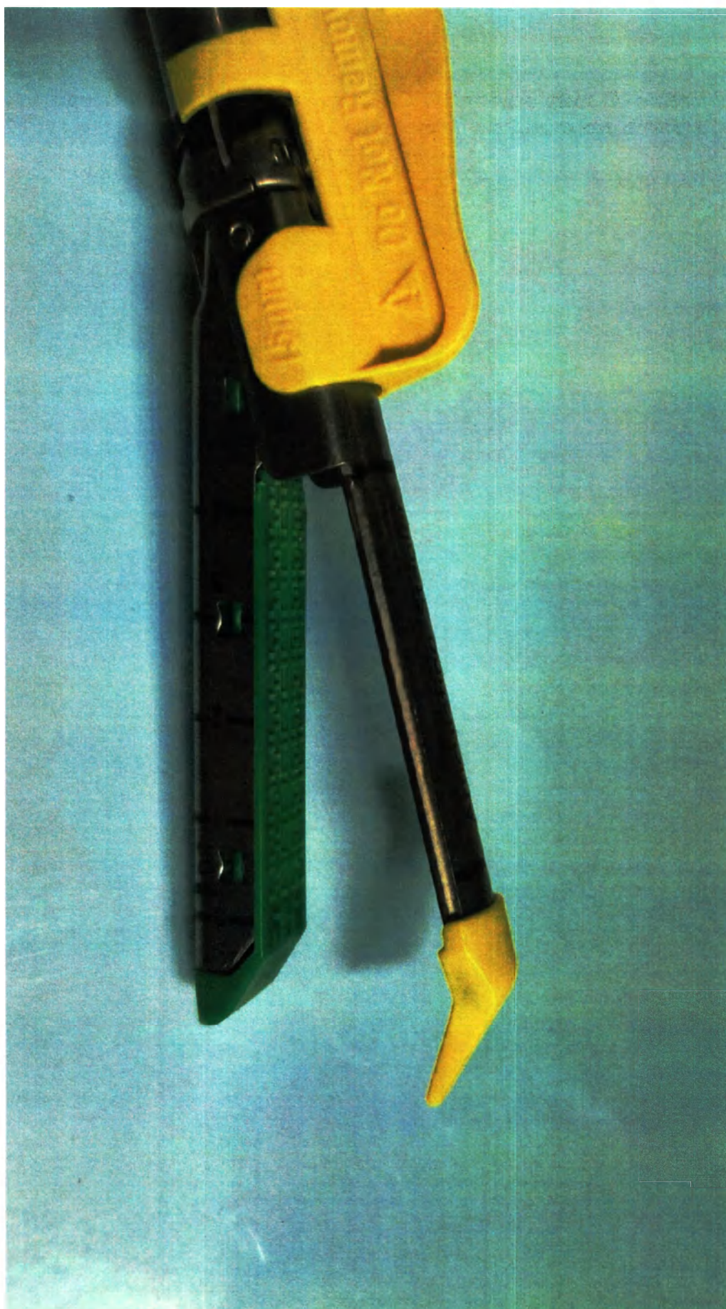
Увеличенное изображение сменного картриджа изделия в варианте исполнения CN-CCRC с кодом цвета G - зелёный, тип 2 (тип 1 выглядит идентично, только без жёлтого съёмного пластикового наконечника), без учёта длины шва
