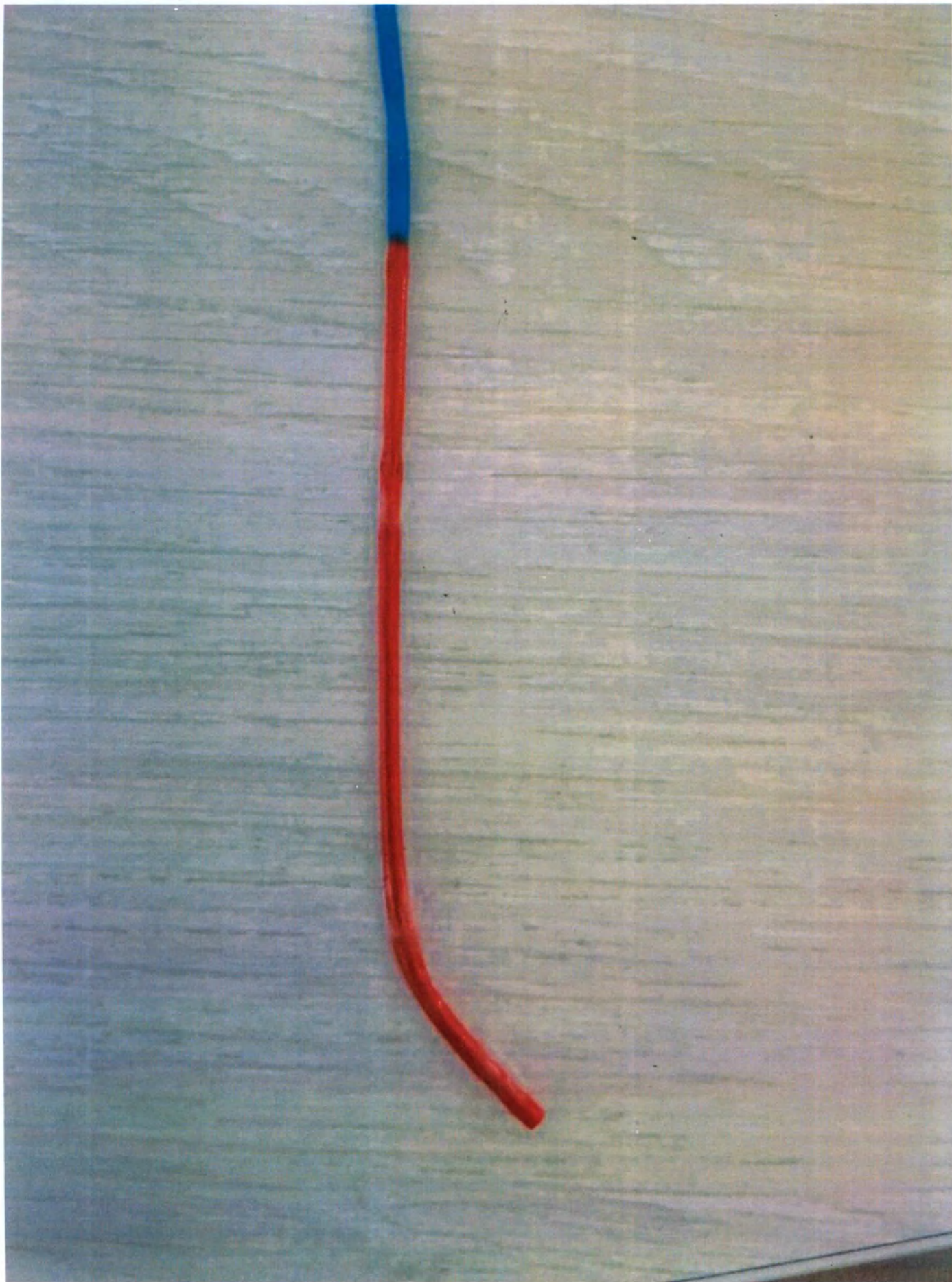
Форма дистального кончика Multipurpose D катетера проводникового для дистального доступа TONBRIDGE Matador
