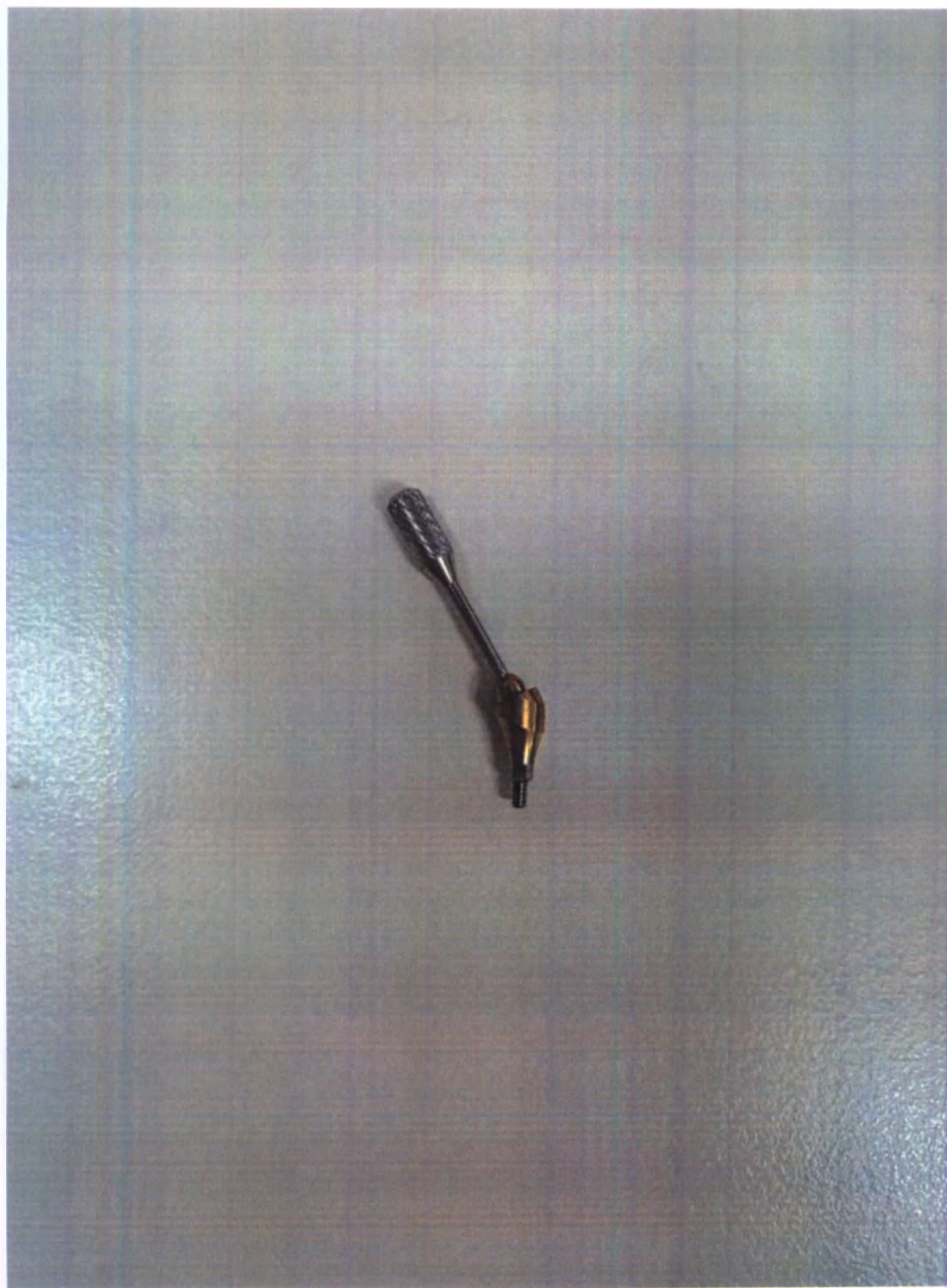
Абатменты Geo для дентальных имплантатов, в варианте исполнения: Абатмент мультивинтовой Geo G-A3035ASR
