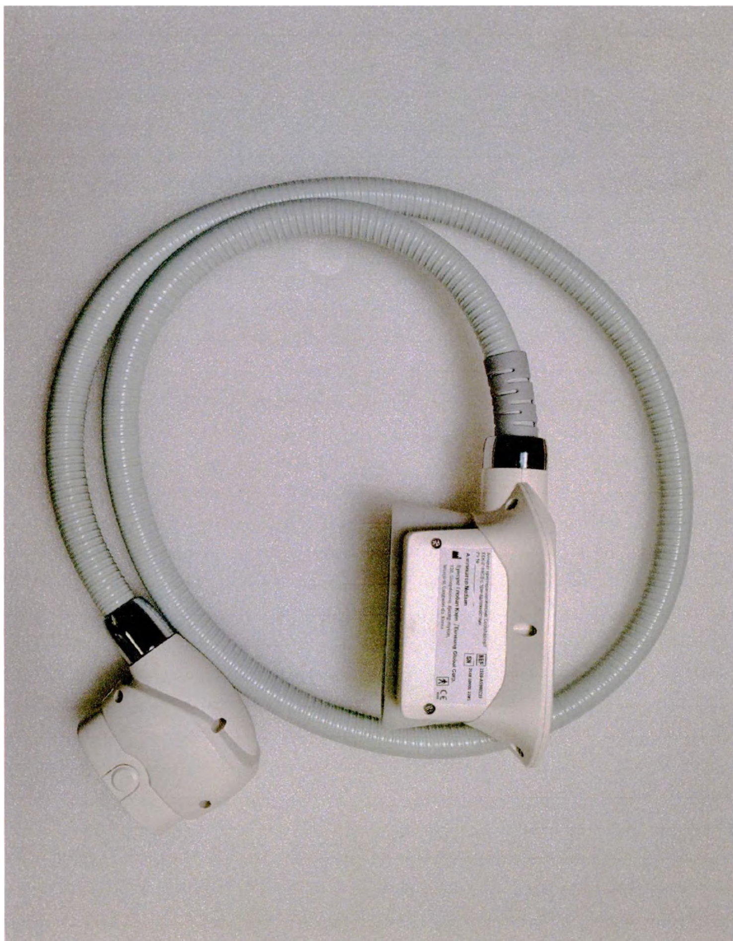
Фотографическое изображение 7. Аппарат криотерапевтический Coolshaping2 ESK-2168CS с принадлежностями. Аппликатор Medium.
