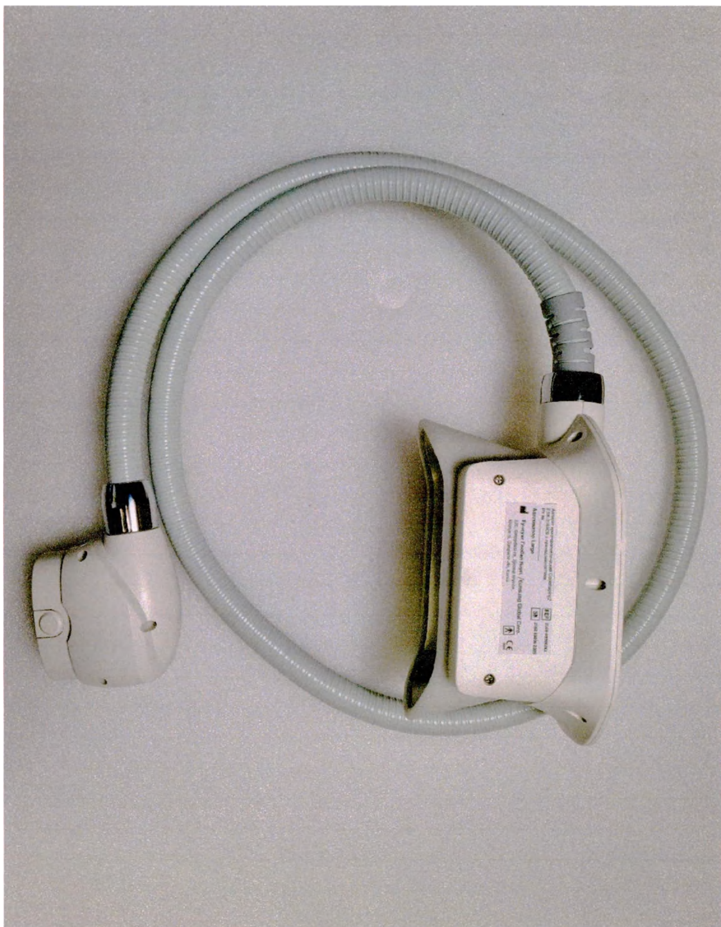
Фотографическое изображение 6. Аппарат криотерапевтический Coolshaping2 ESK-2168CS с принадлежностями. Аппликатор Large.
