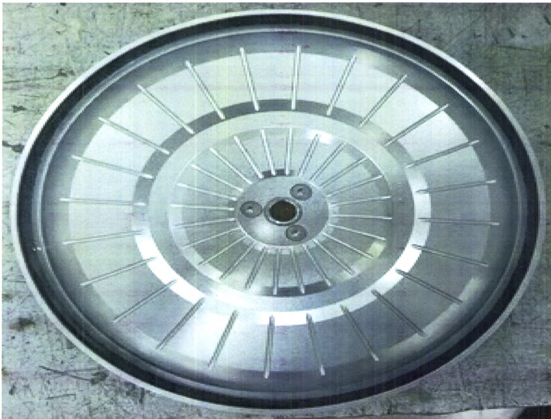
2. Гематокритный ротор на 24 капиллярные пробирки максимальный диаметр пробирки 0,75 мм
