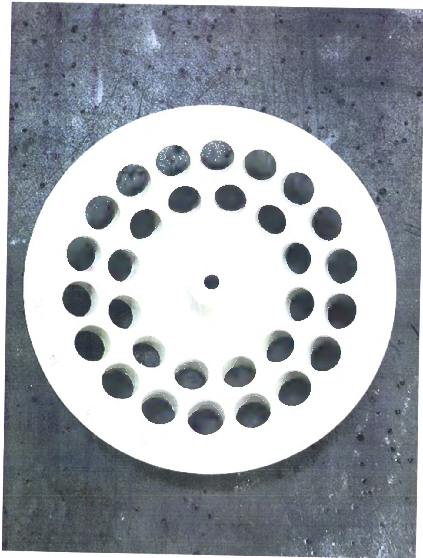
12. Угловой ротор AR 450 30x15 мл для пробирок максимального диаметра 17 мм
