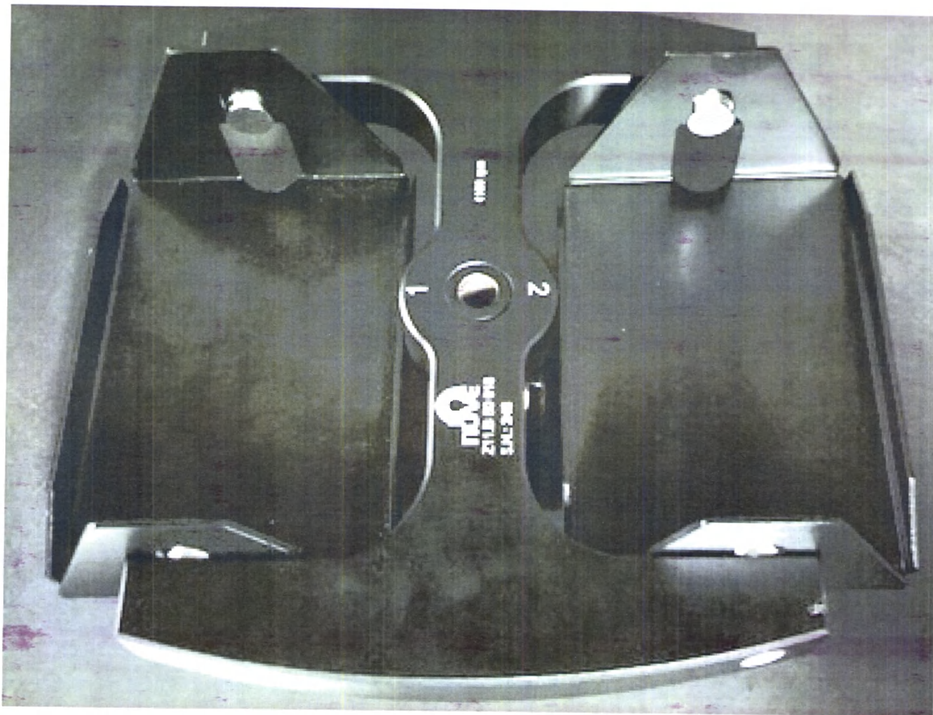
10. Ротор для микротитрования планшетов MP 100
