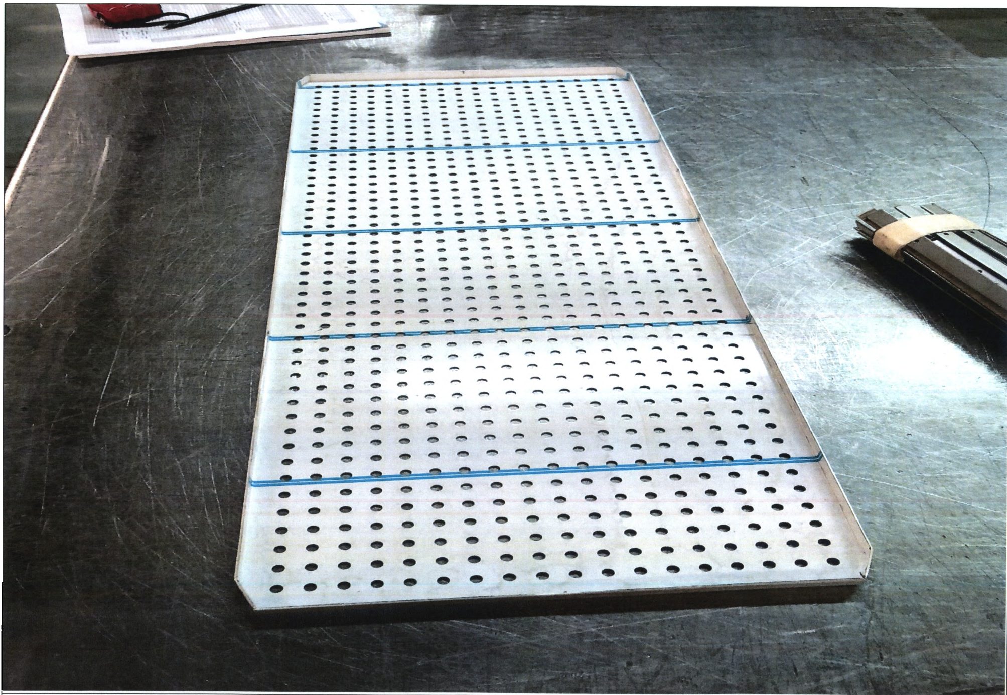
8. Полка (275x740 мм), не более 4 шт. (при необходимости)
