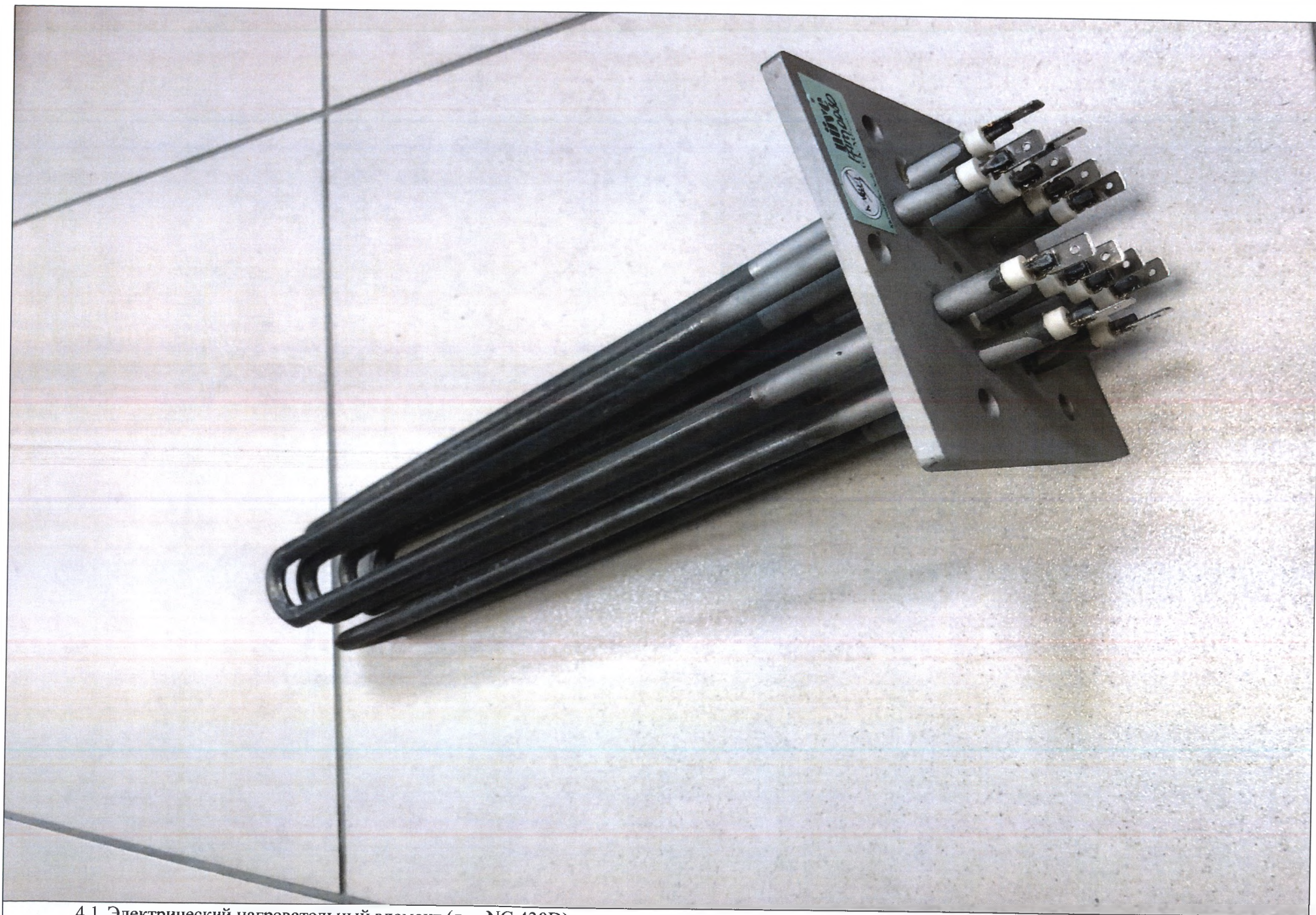
4.1 Электрический нагревательный элемент (для NC 430D)
