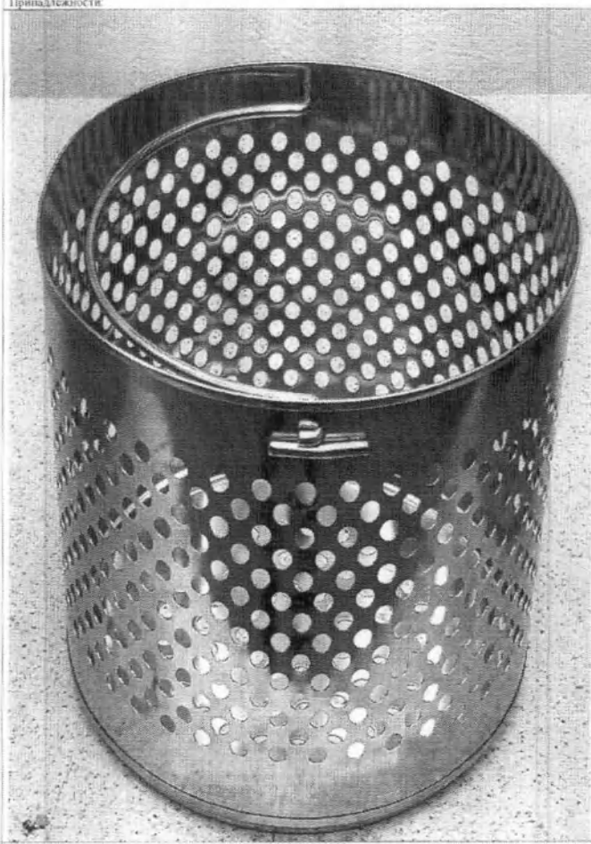
1. Стерилизационная корзина для модели NC 40 M (Ø295 x 345 мм)
