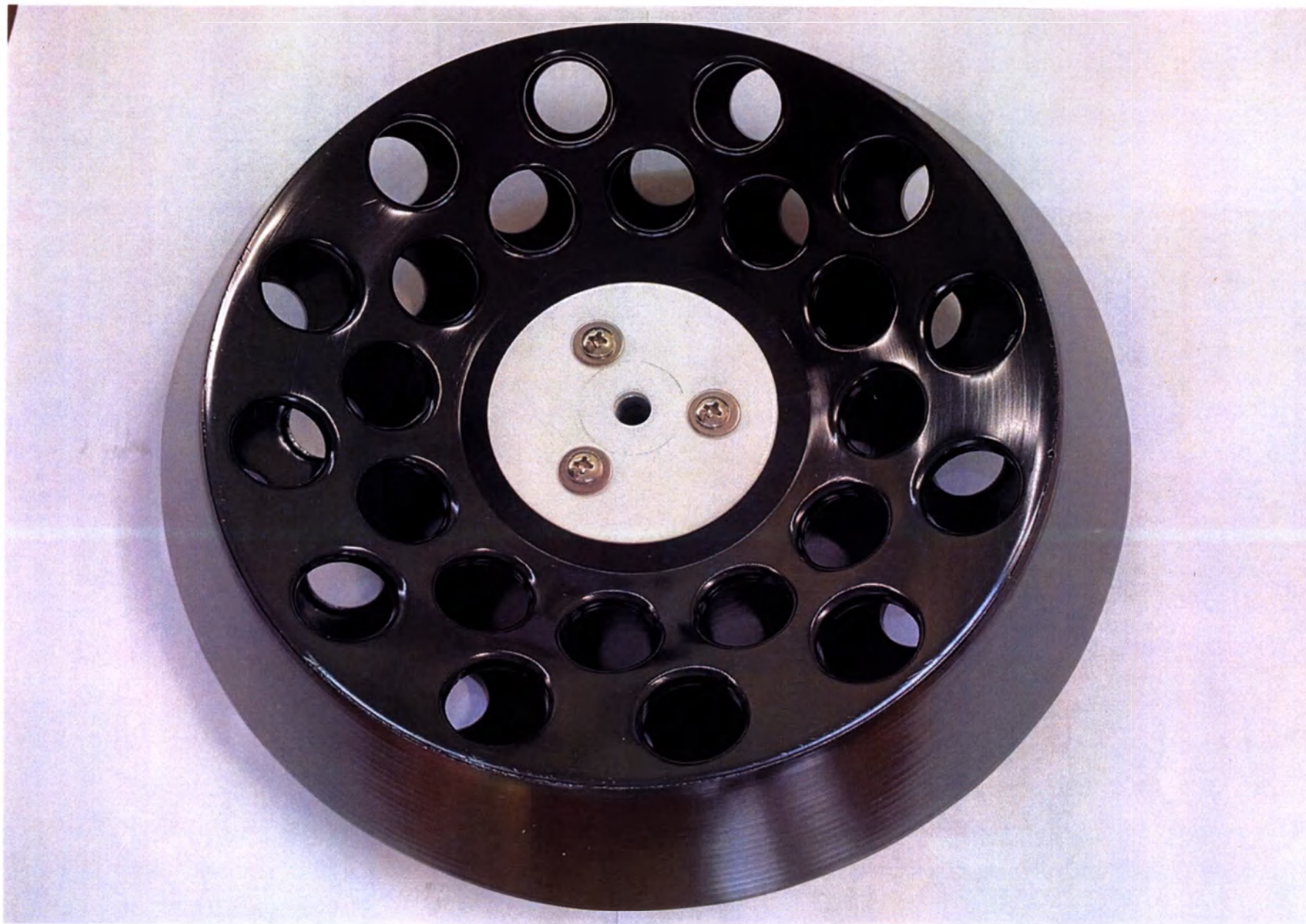
Ротор угловой с 24 лунками
