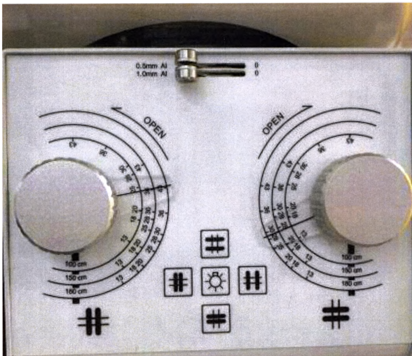
Коллиматор
