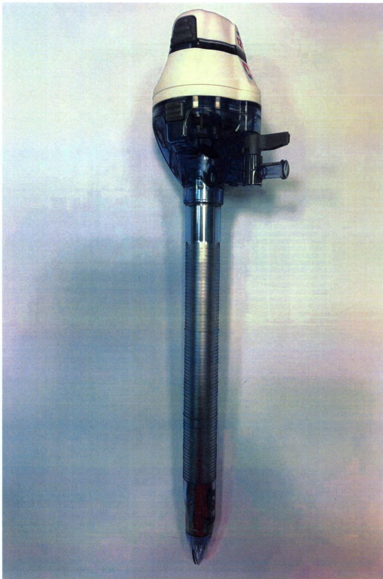
Рисунок 2 – Троакар абдоминальный одноразовый "CHANNEL MED" без дымового фильтра, оптический без лезвия, длинный, вариант исполнения CN-TCI-12L ( в сборе)
