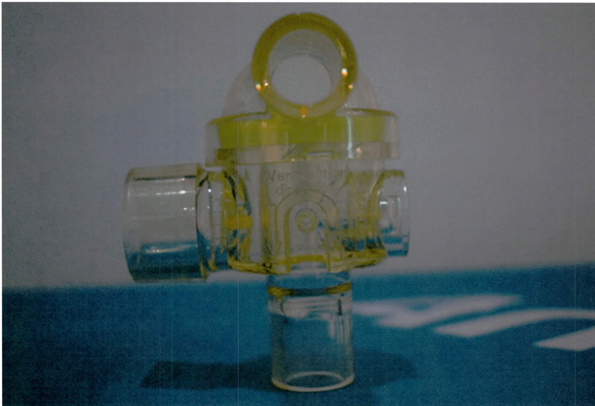
Аппарат искусственной вентиляции легких 6000S с принадлежностями. Клапан пациента
