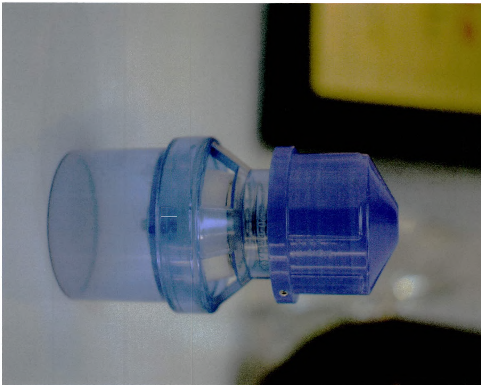
Аппарат искусственной вентиляции легких АП6000М Plus с принадлежностями. Клапан ПДКВ
