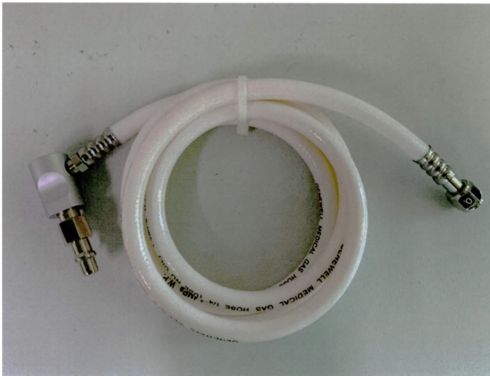
Аппарат искусственной вентиляции легких АИ6000В с принадлежностями. Шланг подачи газа соединительный (для подключения к центральным источникам кислорода)
