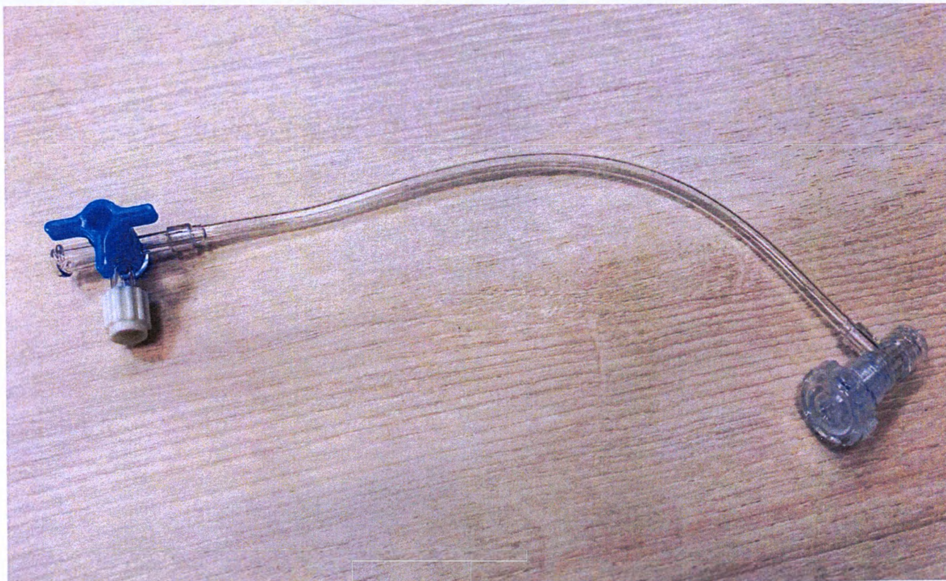
Общий вид гемостатического клапана
