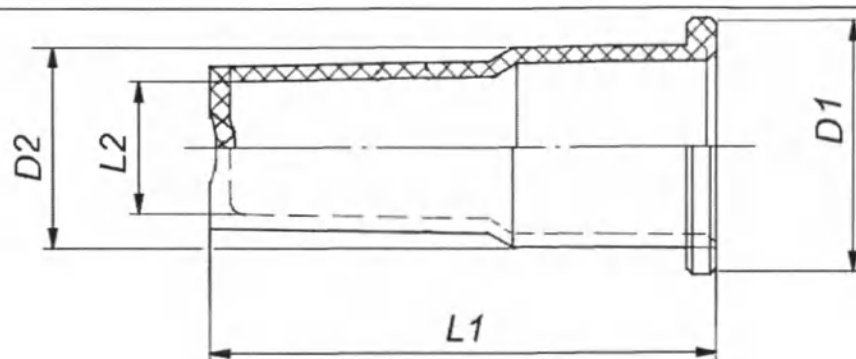
Основные геометрические размеры кюветы
