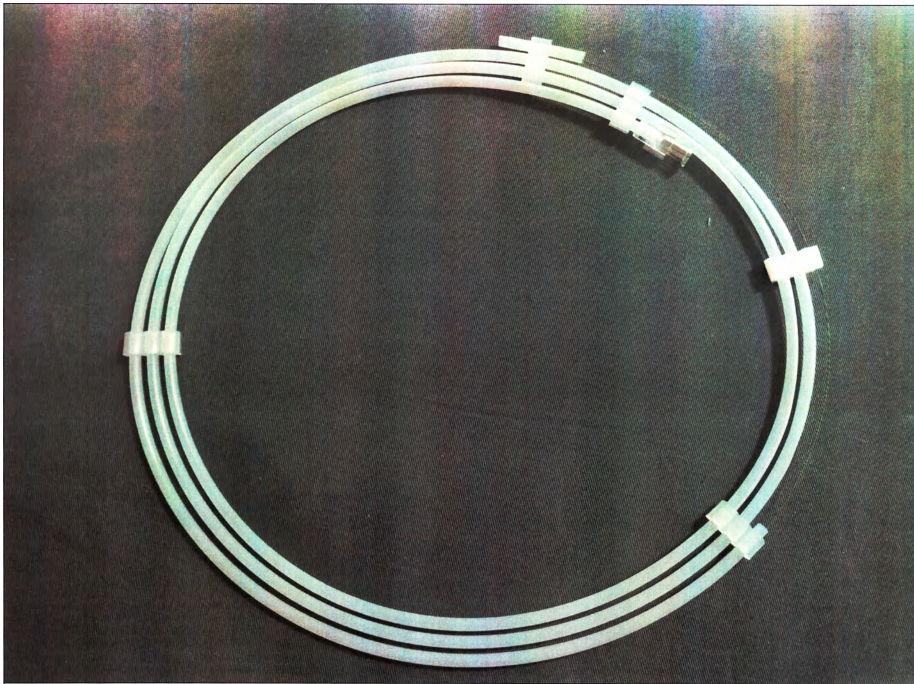
Рис. 31. Проводник периферический Shun Super-V14 с полиуретановой оболочкой и гидрофильным покрытием, диаметр 0,014 дюйма (0,36 мм), длина 200 см, со стальным сердечником, длина рентгеноконтрастного покрытия 5 см, кончик прямой, жесткость 3 г, 18 см
