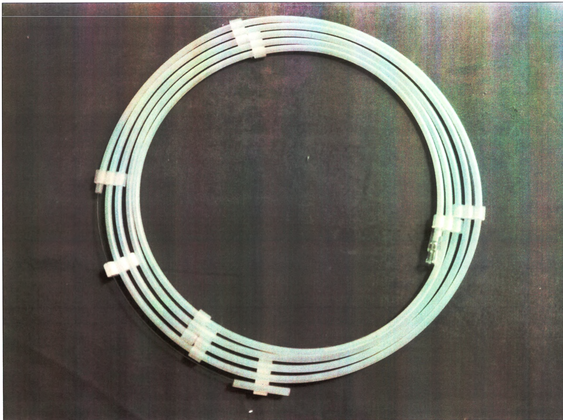
Рис. 7. Проводник периферический Shun Super-V с полиуретановой оболочкой и гидрофильным покрытием, диаметр 0,018 дюйма (0,45 мм), длина 300 см, с композитным сердечником, длина рентгеноконтрастного покрытия 5 см, кончик прямой, жесткость 3 г, 15 см
