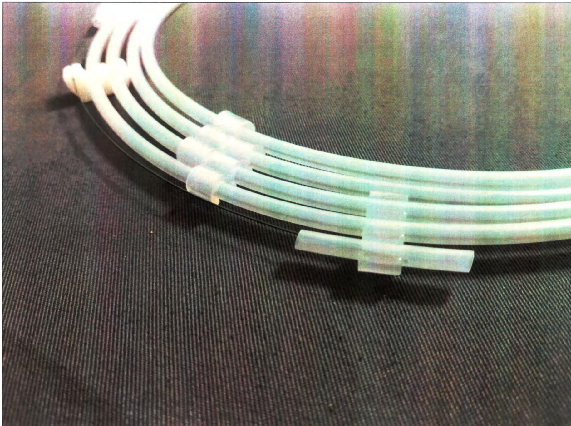
Рис. 8. Проводник периферический Shun Super-V с полиуретановой оболочкой и гидрофильным покрытием, диаметр 0,018 дюйма (0,45 мм), длина 300 см, с композитным сердечником, длина рентгеноконтрастного покрытия 5 см, кончик прямой, жесткость 3 г, 15 см
