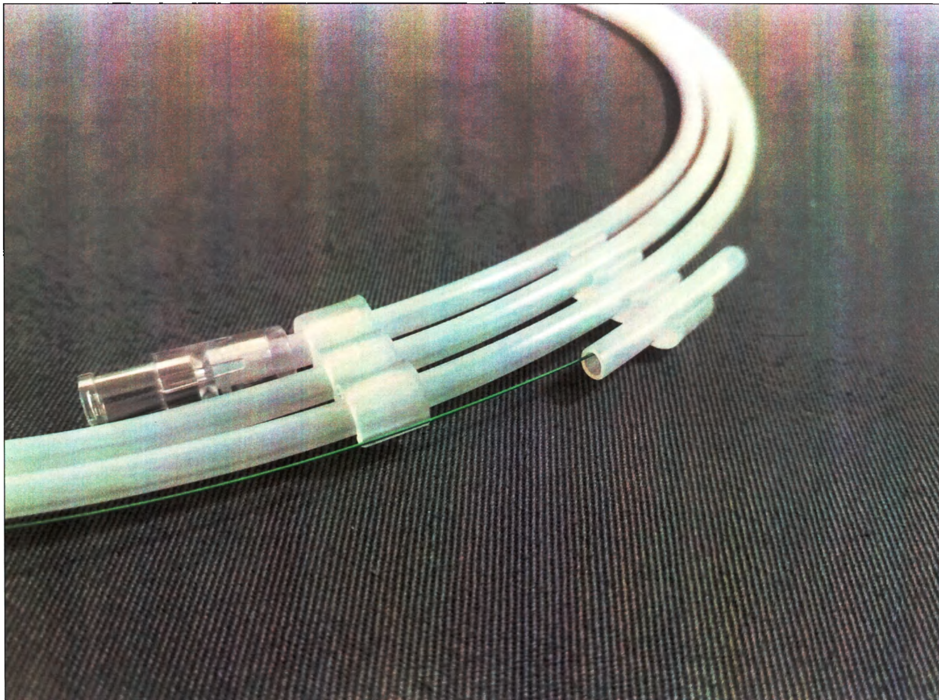
Рис. 33. Проводник периферический Shun Super-V14 с полиуретановой оболочкой и гидрофильным покрытием, диаметр 0,014 дюйма (0,36 мм), длина 200 см, со стальным сердечником, длина рентгеноконтрастного покрытия 5 см, кончик прямой, жесткость 3 г, 18 см
