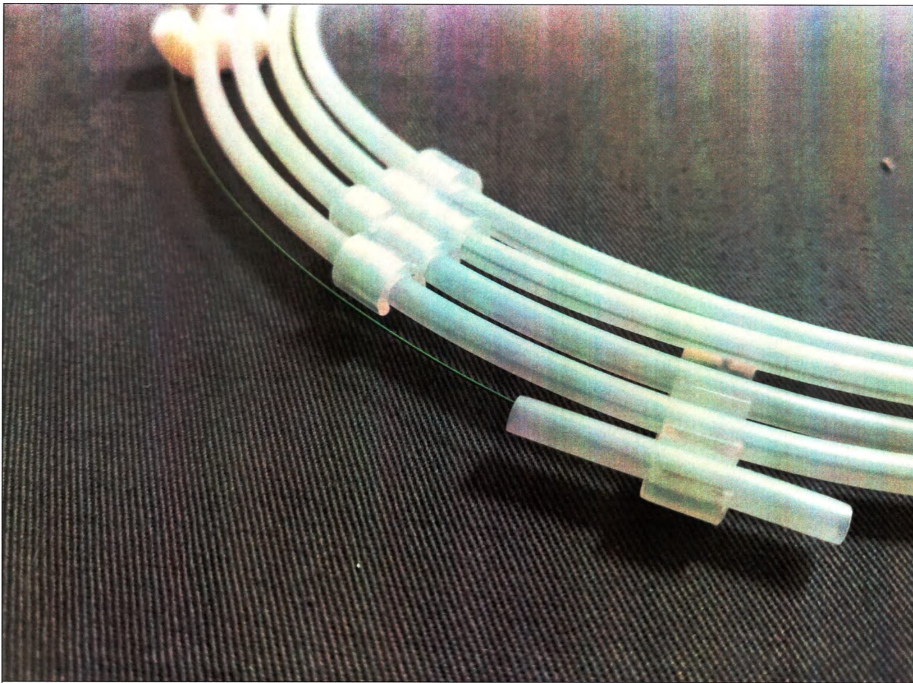
Рис. 12. Проводник периферический Shun Super-V14 с полиуретановой оболочкой и гидрофильным покрытием, диаметр 0,014 дюйма (0,36 мм), длина 300 см, со стальным сердечником, длина рентгеноконтрастного покрытия 5 см, кончик изогнутый, жесткость 3 г, 18 см
