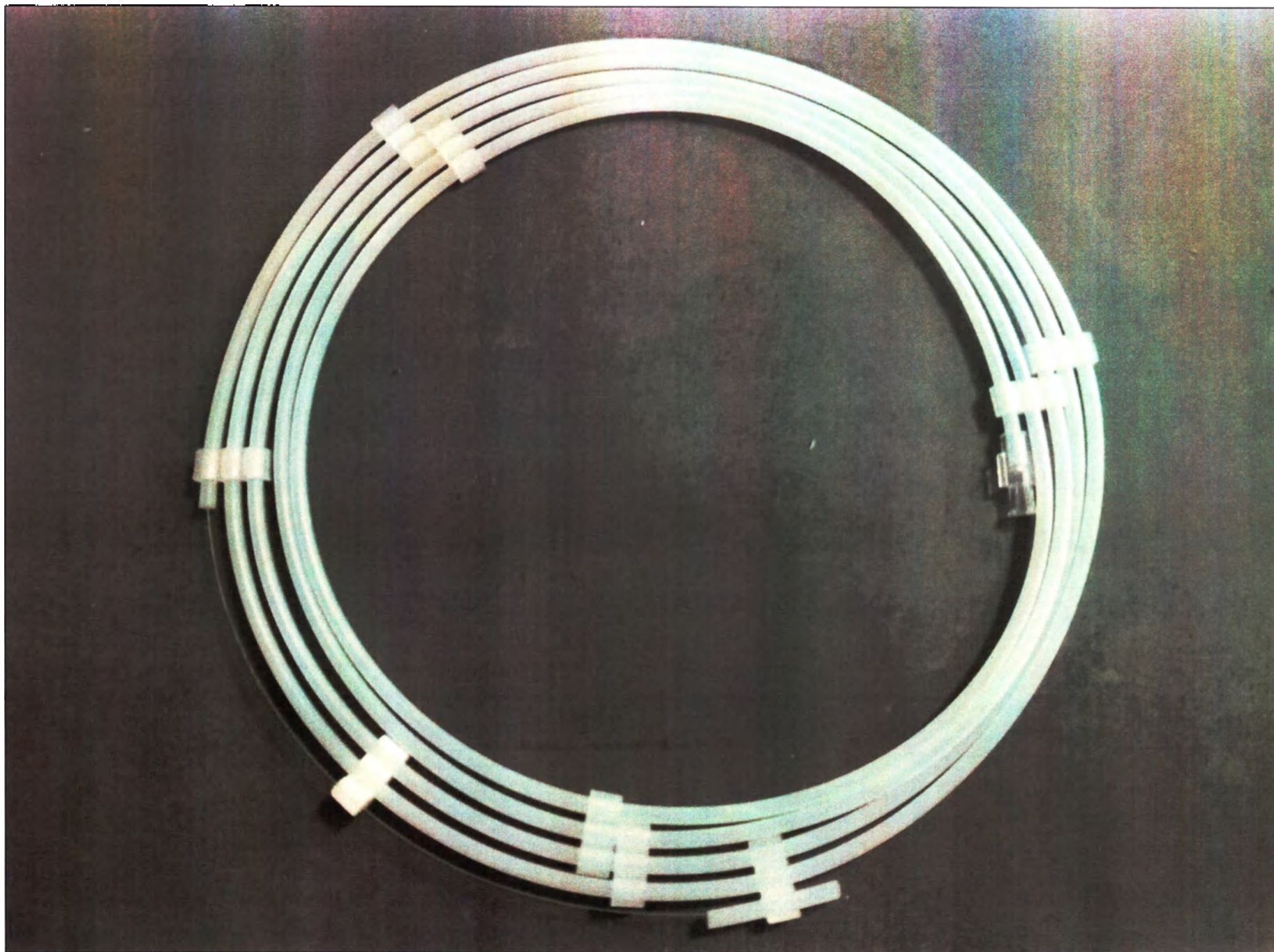
Рис. 15. Проводник периферический Shun Super-V14 с полиуретановой оболочкой и гидрофильным покрытием, диаметр 0,014 дюйма (0,36 мм), длина 300 см, со стальным сердечником, длина рентгеноконтрастного покрытия 5 см, кончик прямой, жесткость 3 г, 18 см
