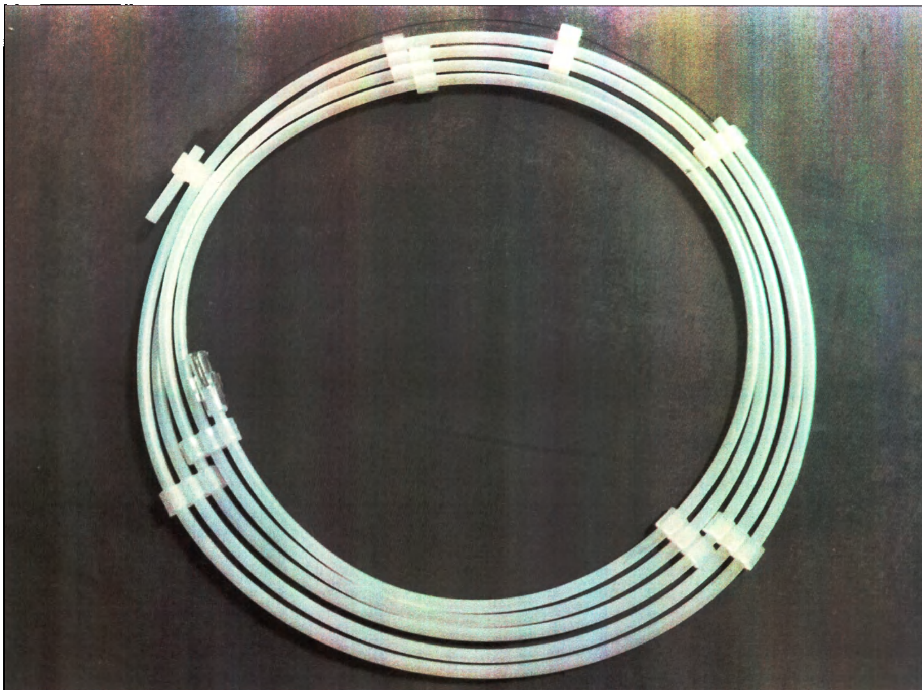
Рис. 27. Проводник периферический Shun Super-V14 с полиуретановой оболочкой и гидрофильным покрытием, диаметр 0,014 дюйма (0,36 мм), длина 300 см, со стальным сердечником, длина рентгеноконтрастного покрытия 3 см, кончик изогнутый, жесткость 6 г, 9 см
