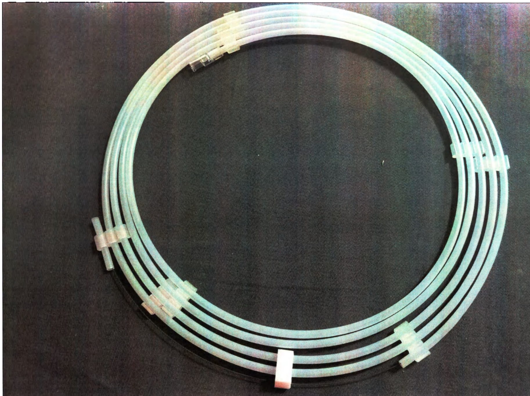
Рис. 43. Проводник периферический Shun Fore с полиуретановой оболочкой и гидрофильным покрытием, диаметр 0,018 дюйма (0,45 мм), длина 300 см, со стальным сердечником, длина рентгеноконтрастного покрытия 3 см, кончик прямой, жесткость 3 г, 46 см
