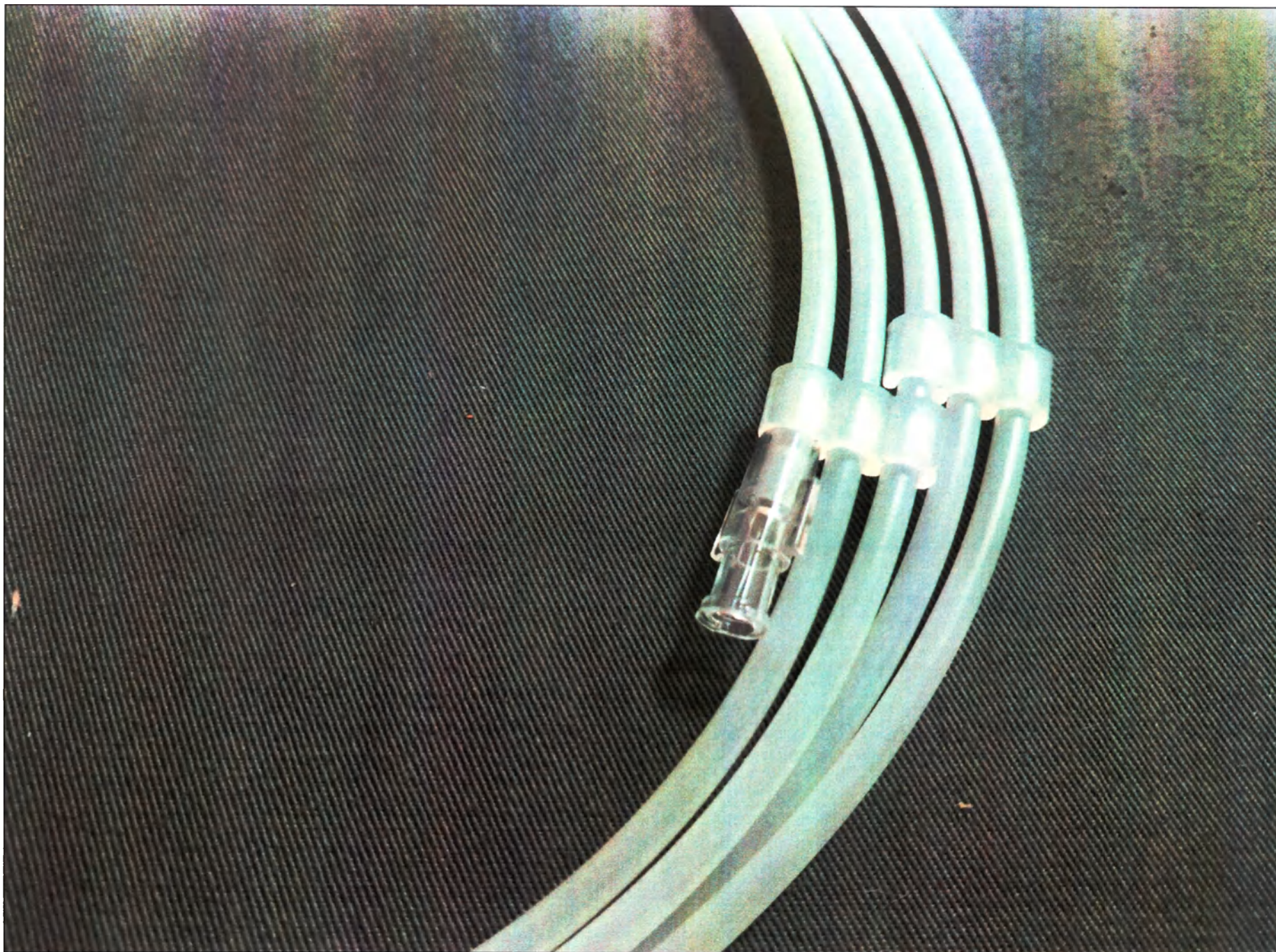
Рис. 13. Проводник периферический Shun Super-V14 с полиуретановой оболочкой и гидрофильным покрытием, диаметр 0,014 дюйма (0,36 мм), длина 300 см, со стальным сердечником, длина рентгеноконтрастного покрытия 5 см, кончик изогнутый, жесткость 3 г, 18 см
