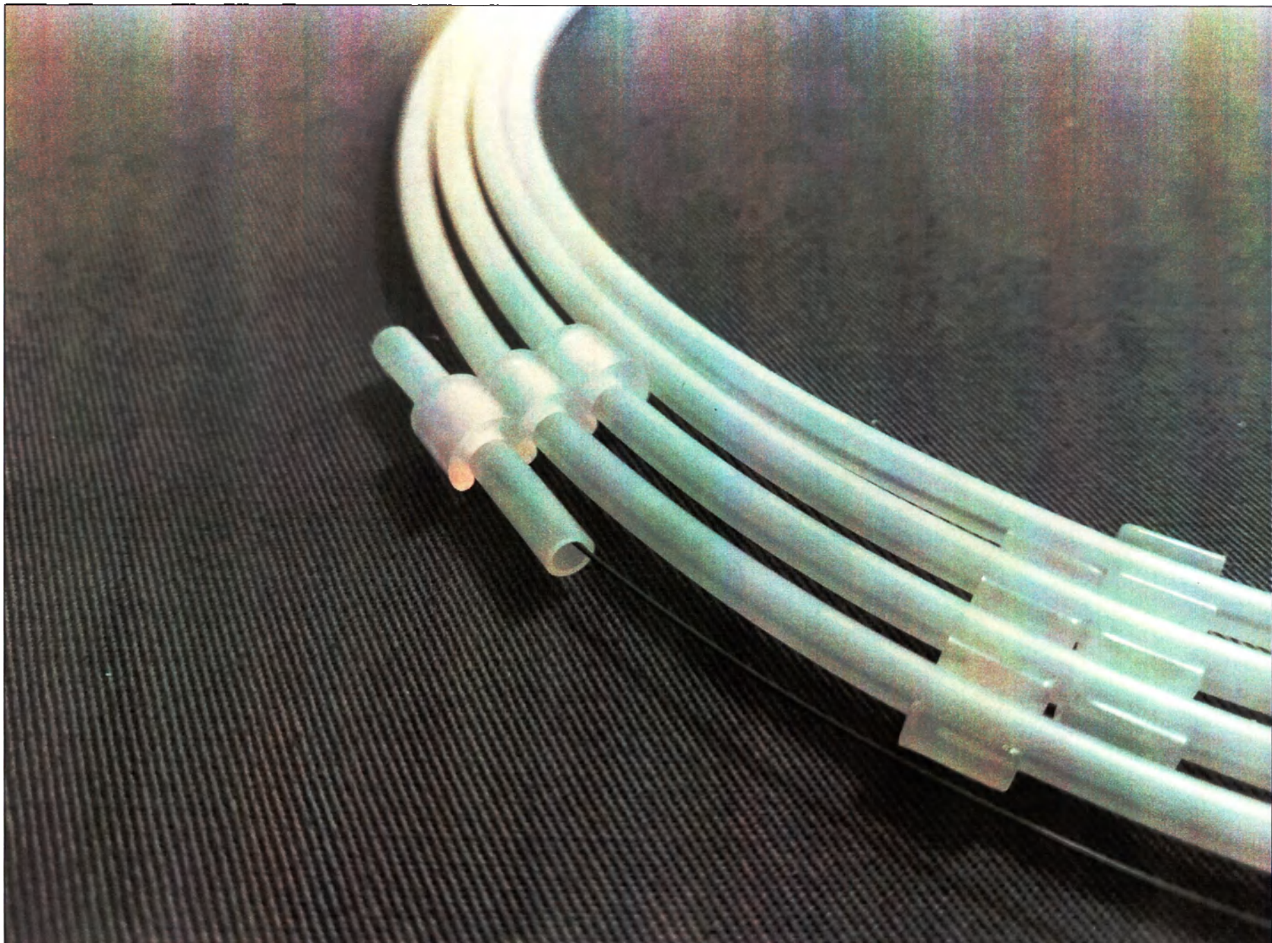
Рис. 45. Проводник периферический Shun Fore с полиуретановой оболочкой и гидрофильным покрытием, диаметр 0,018 дюйма (0,45 мм), длина 300 см, со стальным сердечником, длина рентгеноконтрастного покрытия 3 см, кончик прямой, жесткость 3 г, 46 см
