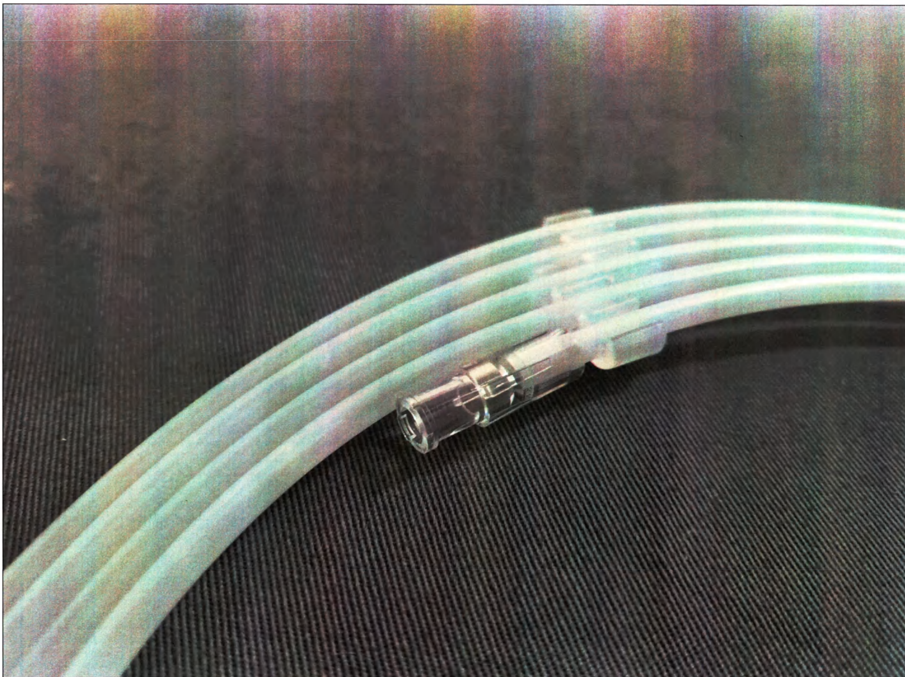
Рис. 44. Проводник периферический Shun Fore с полиуретановой оболочкой и гидрофильным покрытием, диаметр 0,018 дюйма (0,45 мм), длина 300 см, со стальным сердечником, длина рентгеноконтрастного покрытия 3 см, кончик прямой, жесткость 3 г, 46 см
