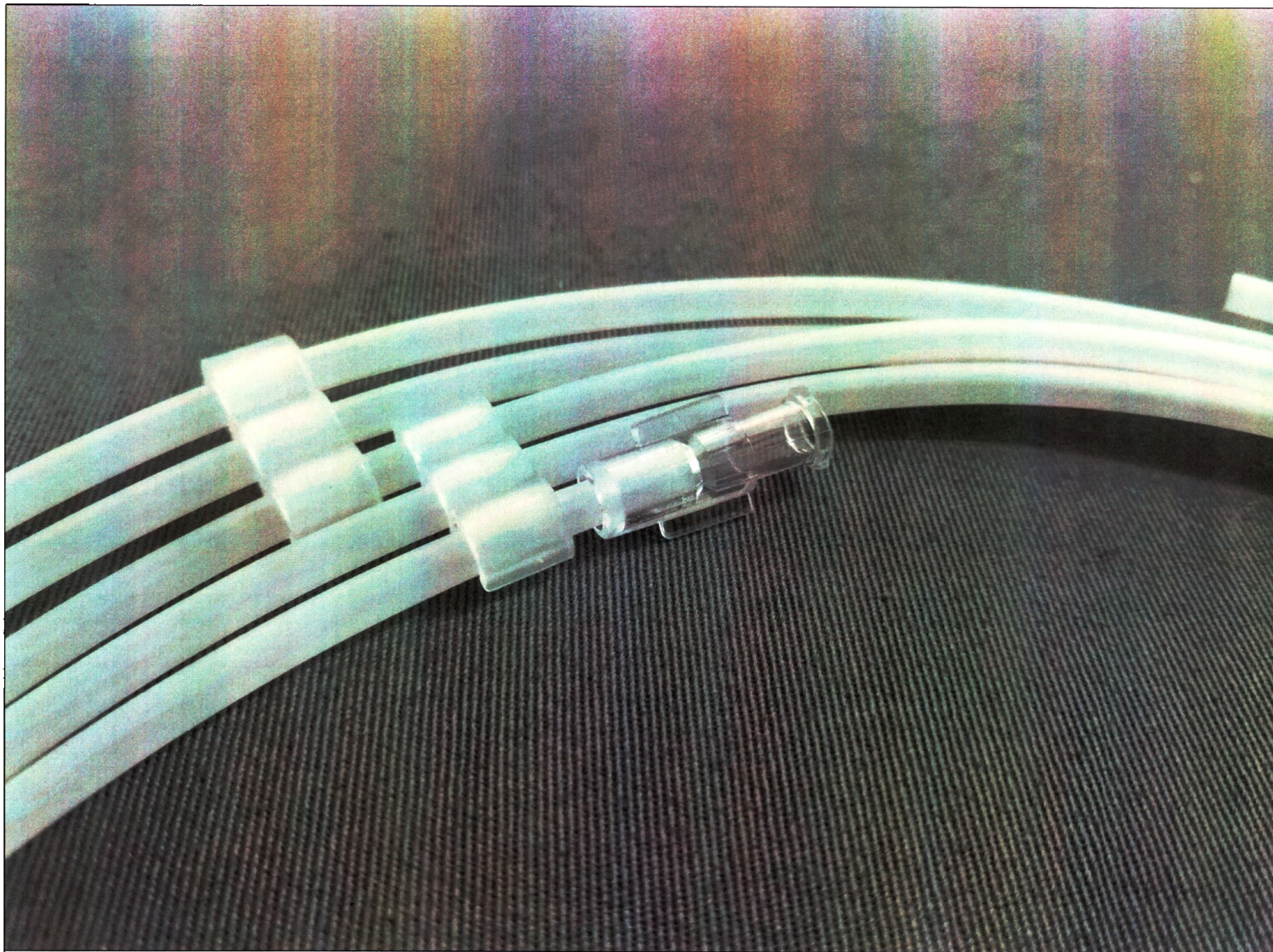
Рис. 28. Проводник периферический Shun Super-V14 с полиуретановой оболочкой и гидрофильным покрытием, диаметр 0,014 дюйма (0,36 мм), длина 300 см, со стальным сердечником, длина рентгеноконтрастного покрытия 3 см, кончик изогнутый, жесткость 6 г, 9 см
