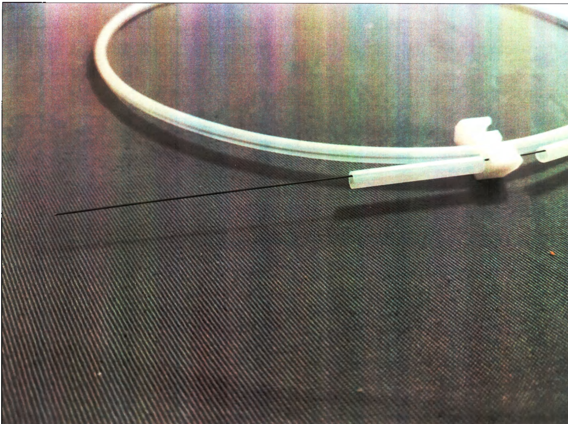
Рис. 5. Проводник периферический Shun Super-V с полиуретановой оболочкой и гидрофильным покрытием, диаметр 0,018 дюйма (0,45 мм), длина 110 см, с композитным сердечником, длина рентгеноконтрастного покрытия 5 см, кончик прямой, жесткость 3 г, 15 см
