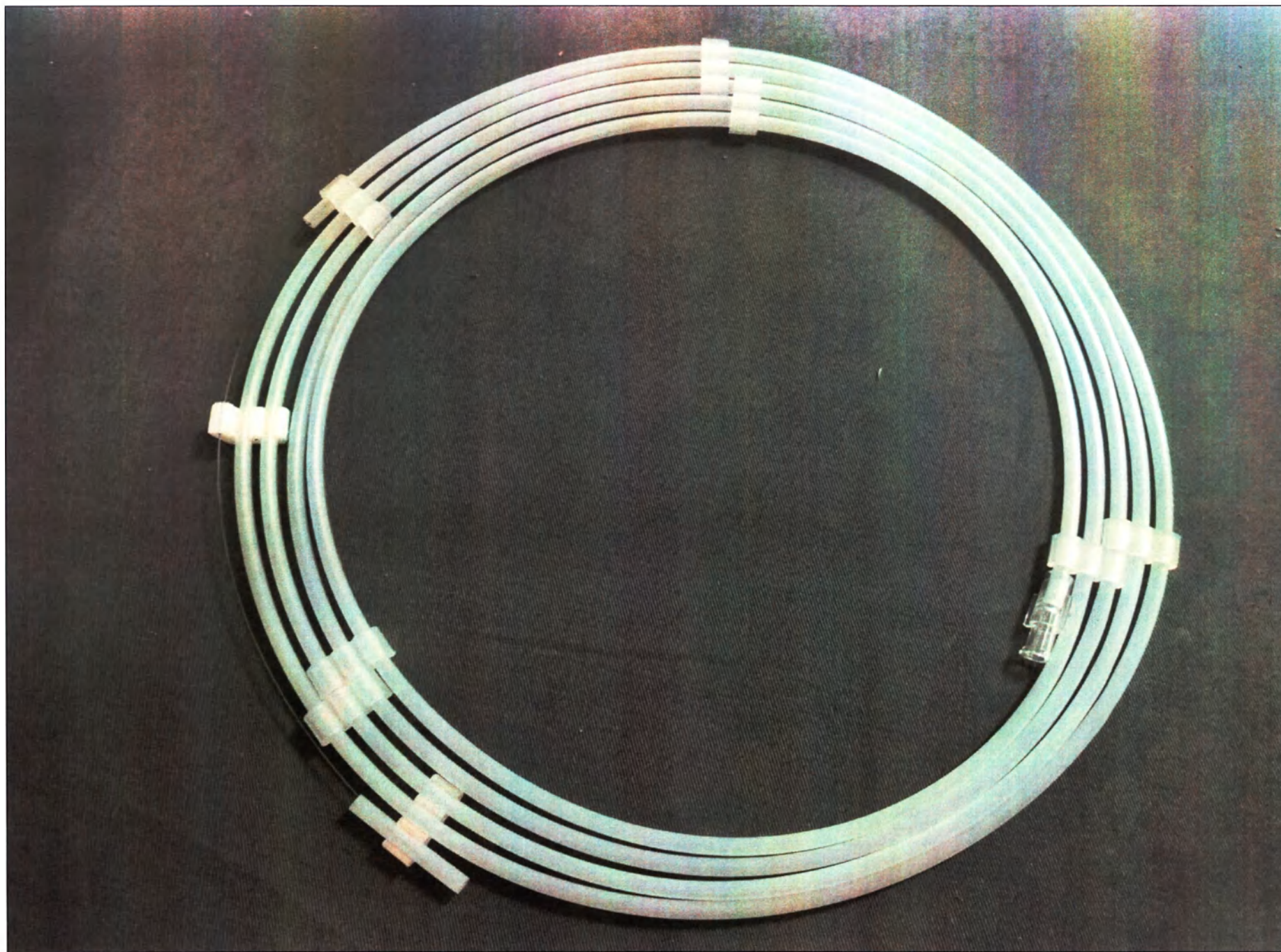
Рис. 23. Проводник периферический Shun Super-V с полиуретановой оболочкой и гидрофильным покрытием, диаметр 0,018 дюйма (0,45 мм), длина 300 см, со стальным сердечником, длина рентгеноконтрастного покрытия 3 см, кончик прямой, жесткость 6 г, 9 см
