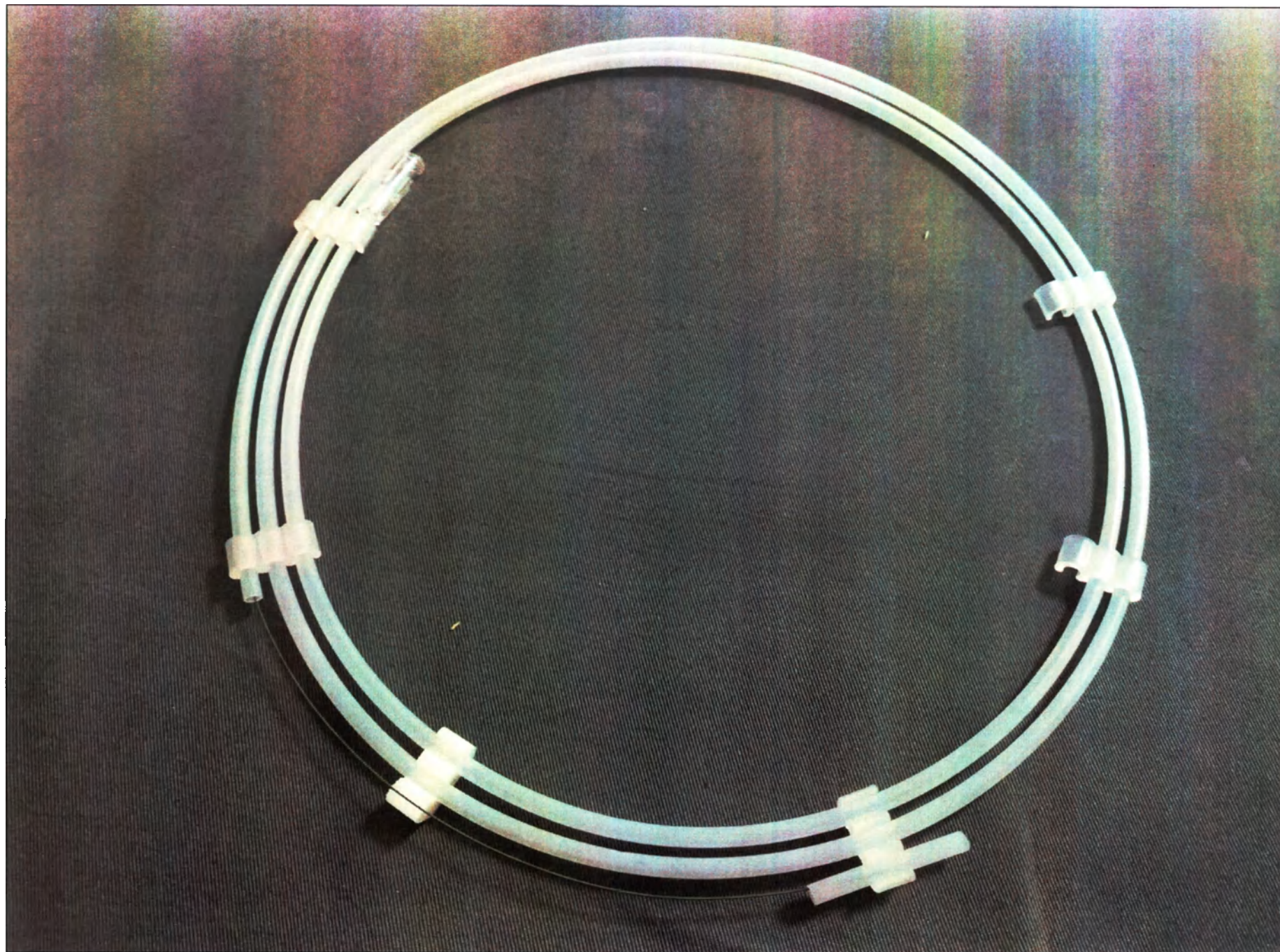
Рис. 39. Проводник периферический Shun Fore с полиуретановой оболочкой и гидрофильным покрытием, диаметр 0,018 дюйма (0,45 мм), длина 150 см, со стальным сердечником, длина рентгеноконтрастного покрытия 3 см, кончик прямой, жесткость 3 г, 46 см
