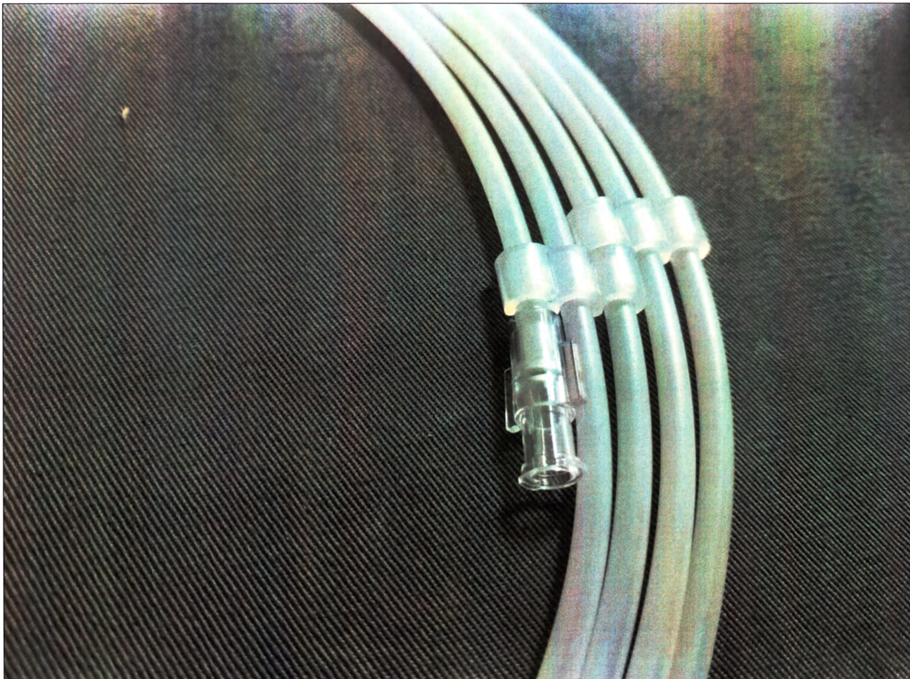
Рис. 24. Проводник периферический Shun Super-V с полиуретановой оболочкой и гидрофильным покрытием, диаметр 0,018 дюйма (0,45 мм), длина 300 см, со стальным сердечником, длина рентгеноконтрастного покрытия 3 см, кончик прямой, жесткость 6 г, 9 см
