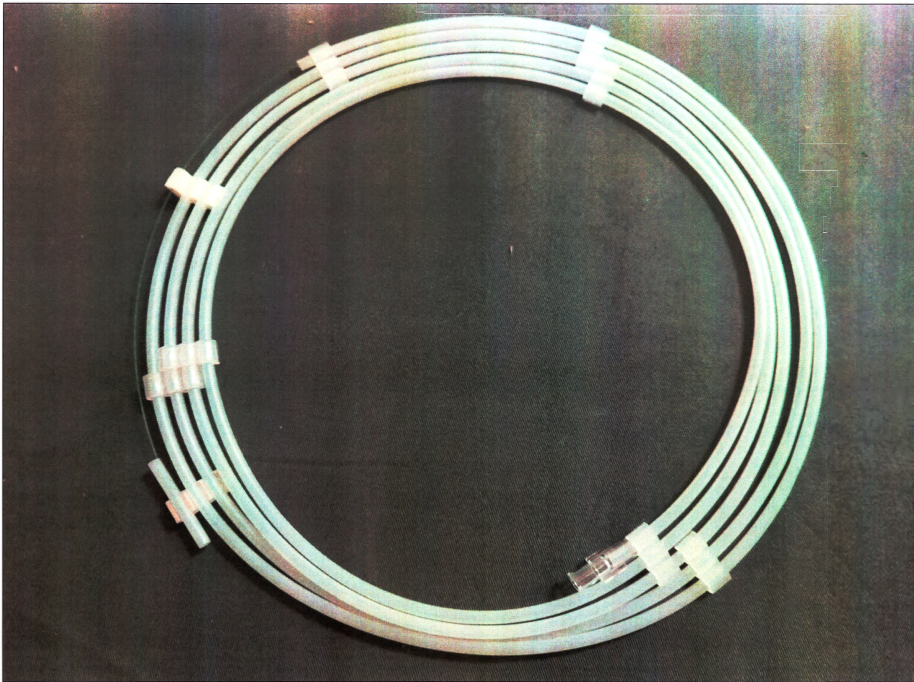
Рис. 11. Проводник периферический Shun Super-V14 с полиуретановой оболочкой и гидрофильным покрытием, диаметр 0,014 дюйма (0,36 мм), длина 300 см, со стальным сердечником, длина рентгеноконтрастного покрытия 5 см, кончик изогнутый, жесткость 3 г, 18 см
