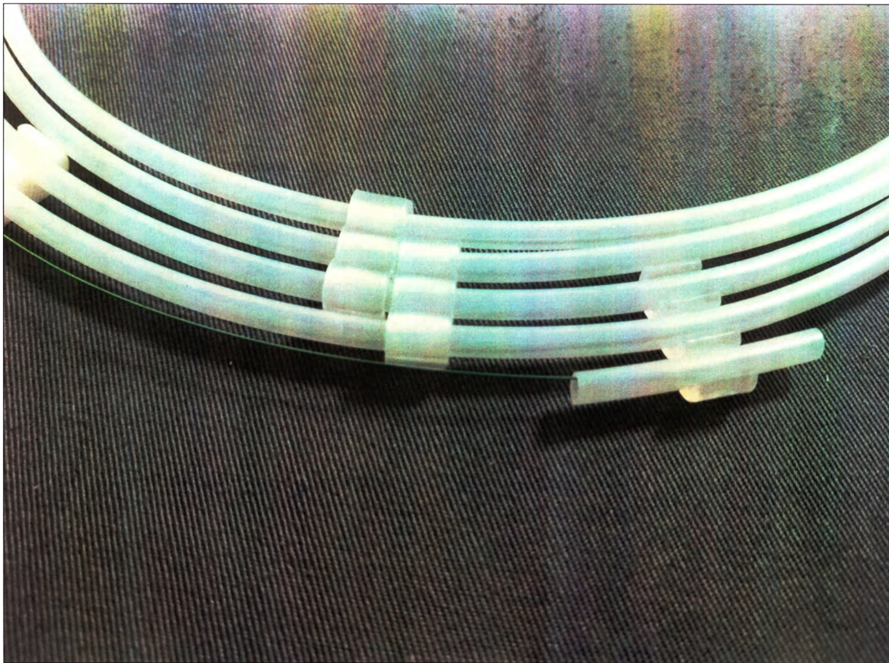
Рис. 16. Проводник периферический Shun Super-V14 с полиуретановой оболочкой и гидрофильным покрытием, диаметр 0,014 дюйма (0,36 мм), длина 300 см, со стальным сердечником, длина рентгеноконтрастного покрытия 5 см, кончик прямой, жесткость 3 г, 18 см – 1 шт
