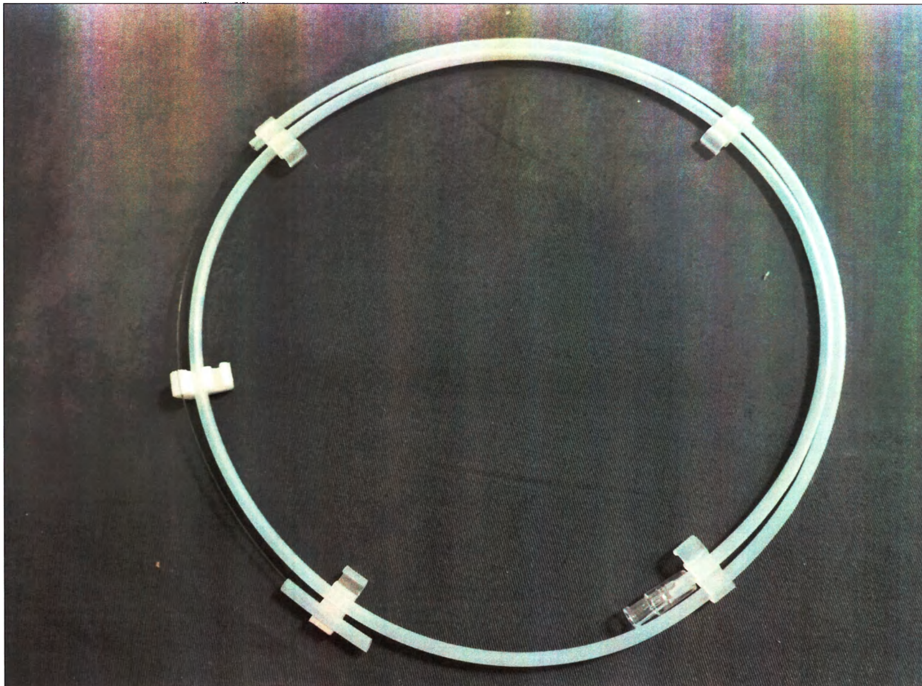
Рис. 35. Проводник периферический Shun Fore с полиуретановой оболочкой и гидрофильным покрытием, диаметр 0,018 дюйма (0,45 мм), длина 110 см, со стальным сердечником, длина рентгеноконтрастного покрытия 3 см, кончик прямой, жесткость 3 г, 46 см
