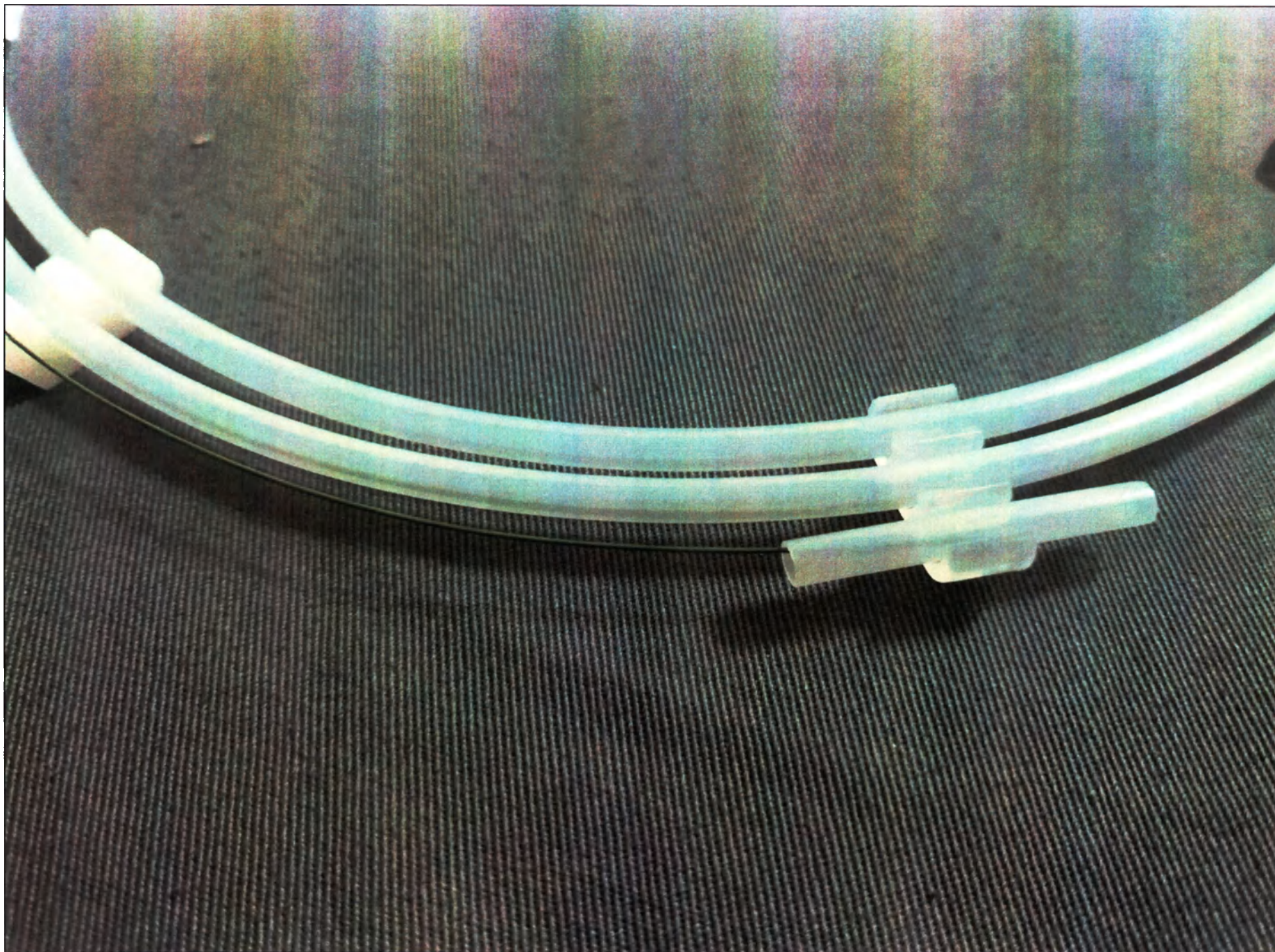
Рис. 40. Проводник периферический Shun Fore с полиуретановой оболочкой и гидрофильным покрытием, диаметр 0,018 дюйма (0,45 мм), длина 150 см, со стальным сердечником, длина рентгеноконтрастного покрытия 3 см, кончик прямой, жесткость 3 г, 46 см
