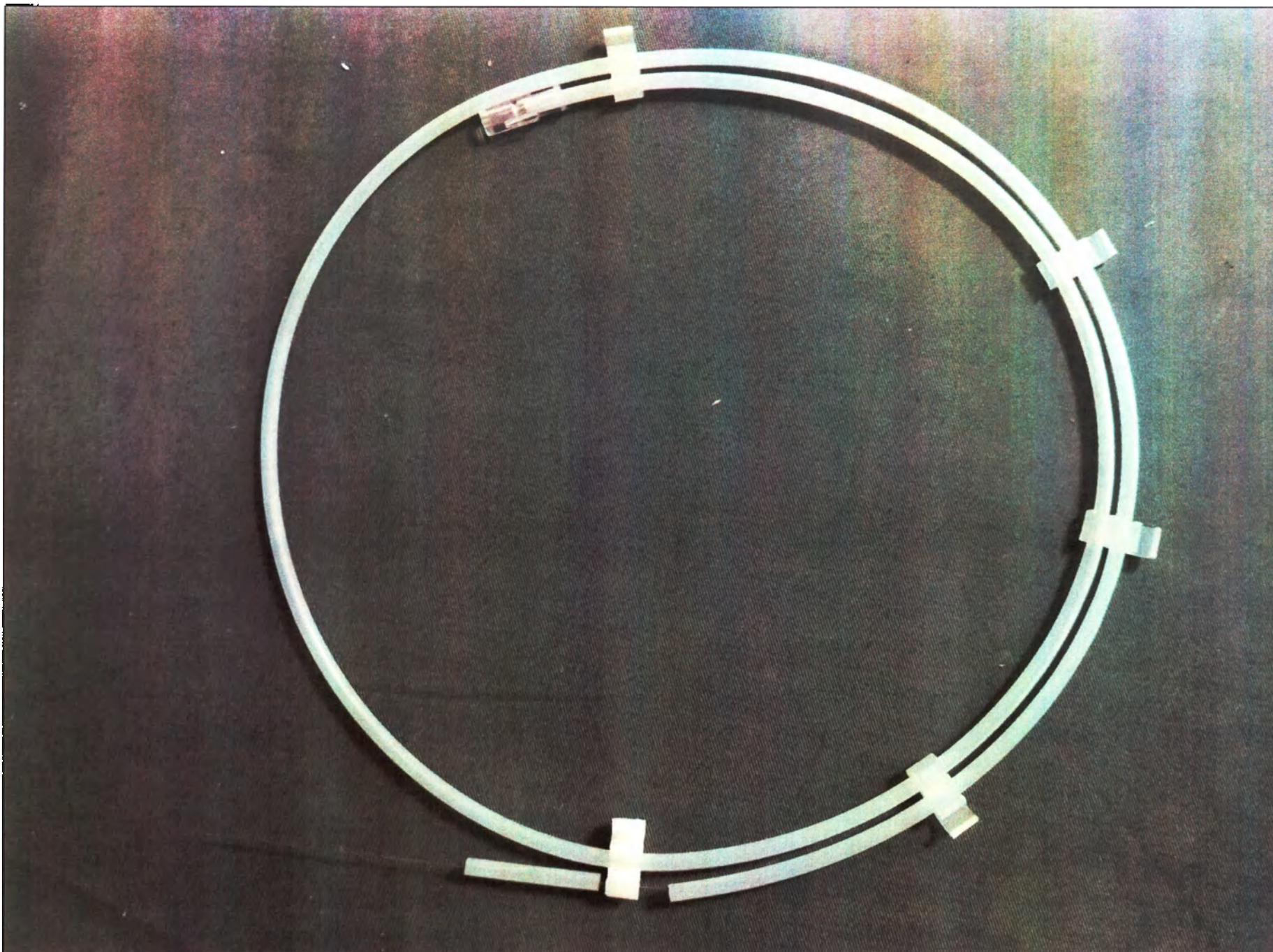
Рис. 3. Проводник периферический Shun Super-V с полиуретановой оболочкой и гидрофильным покрытием, диаметр 0,018 дюйма (0,45 мм), длина 110 см, с композитным сердечником, длина рентгеноконтрастного покрытия 5 см, кончик прямой, жесткость 3 г, 15 см
