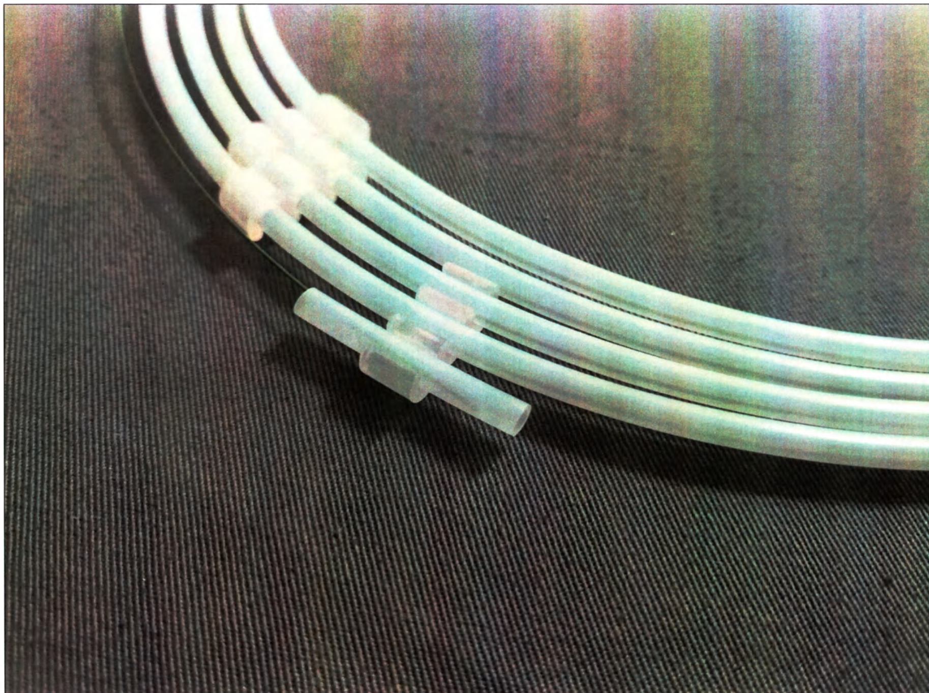
Рис. 25. Проводник периферический Shun Super-V с полиуретановой оболочкой и гидрофильным покрытием, диаметр 0,018 дюйма (0,45 мм), длина 300 см, со стальным сердечником, длина рентгеноконтрастного покрытия 3 см, кончик прямой, жесткость 6 г, 9 см
