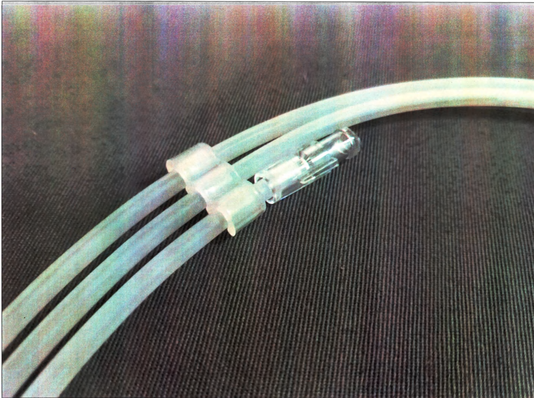
Рис. 41. Проводник периферический Shun Fore с полиуретановой оболочкой и гидрофильным покрытием, диаметр 0,018 дюйма (0,45 мм), длина 150 см, со стальным сердечником, длина рентгеноконтрастного покрытия 3 см, кончик прямой, жесткость 3 г, 46 см
