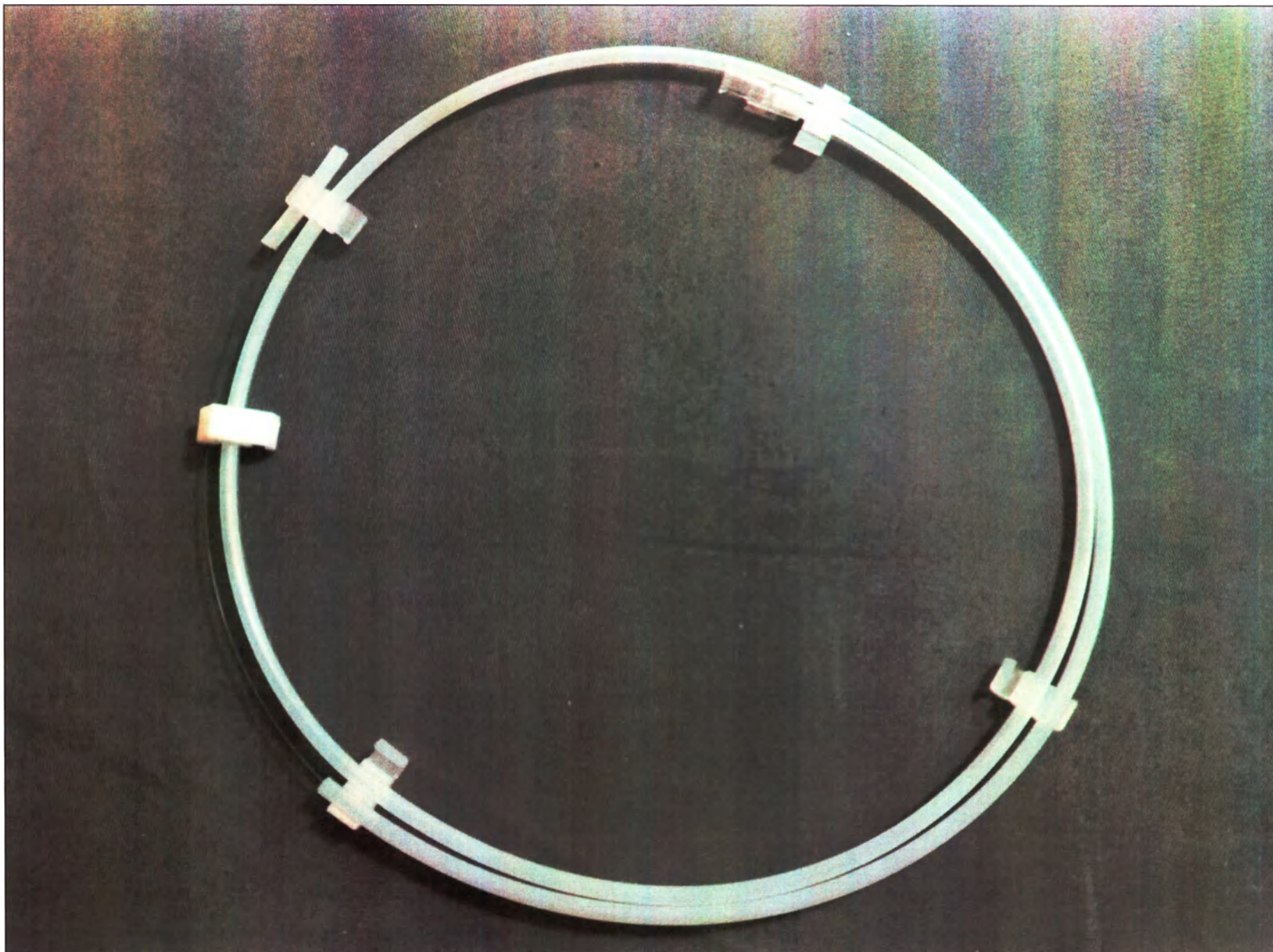
Рис. 19. Проводник периферический Shun Super-V с полиуретановой оболочкой и гидрофильным покрытием, диаметр 0,018 дюйма (0,45 мм), длина 110 см, со стальным сердечником, длина рентгеноконтрастного покрытия 3 см, кончик прямой, жесткость 6 г, 9 см
