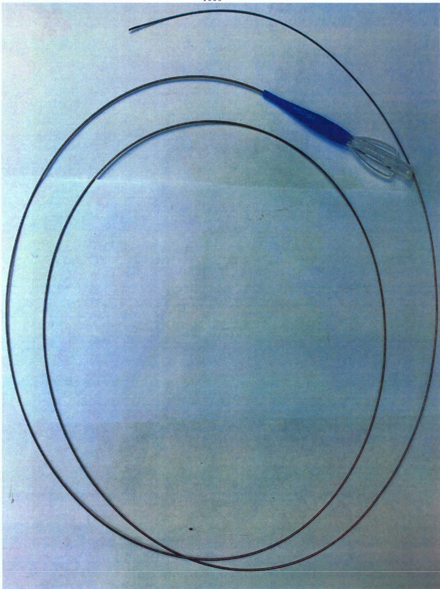
Рисунок 9. Внешний вид Микрокатетера сосудистого Teleport с рабочей длиной 135 см 220-13-1000
