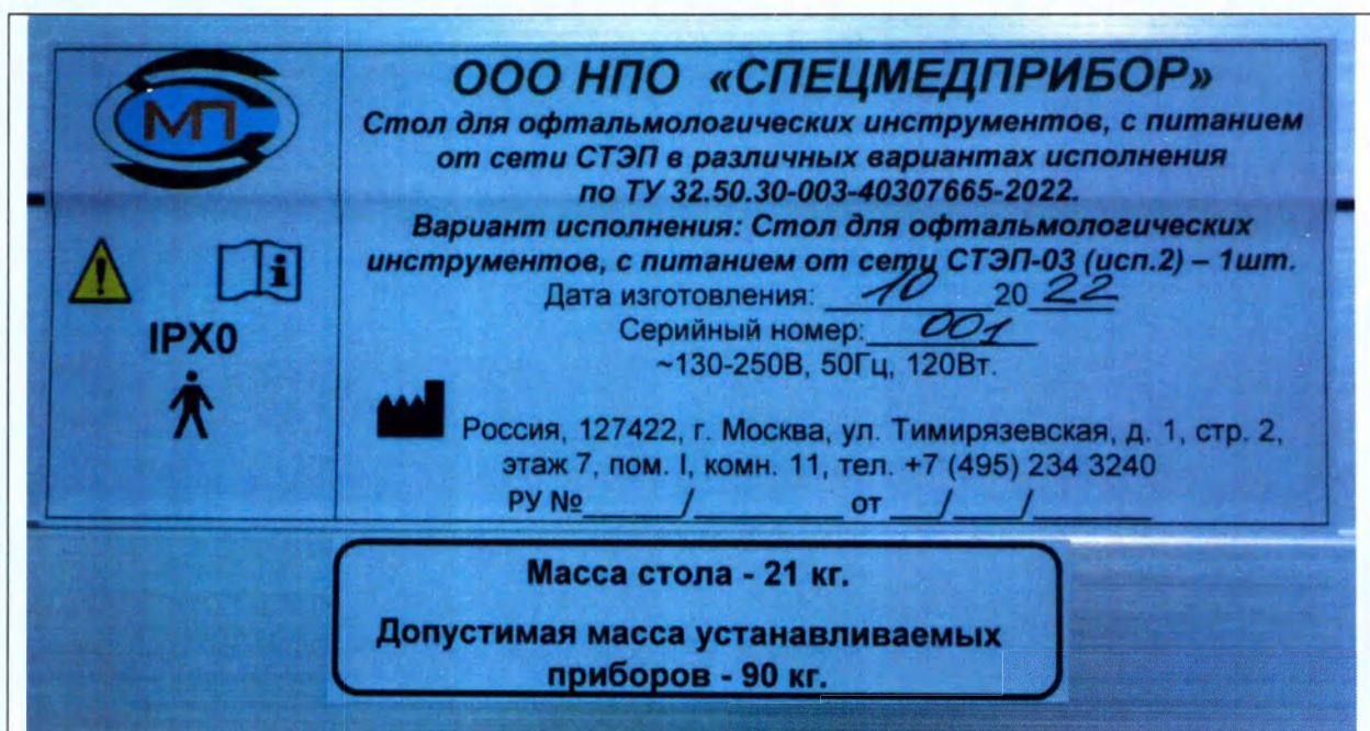
Рис.8 Шильдик СТЭП-03 (исп.2)
