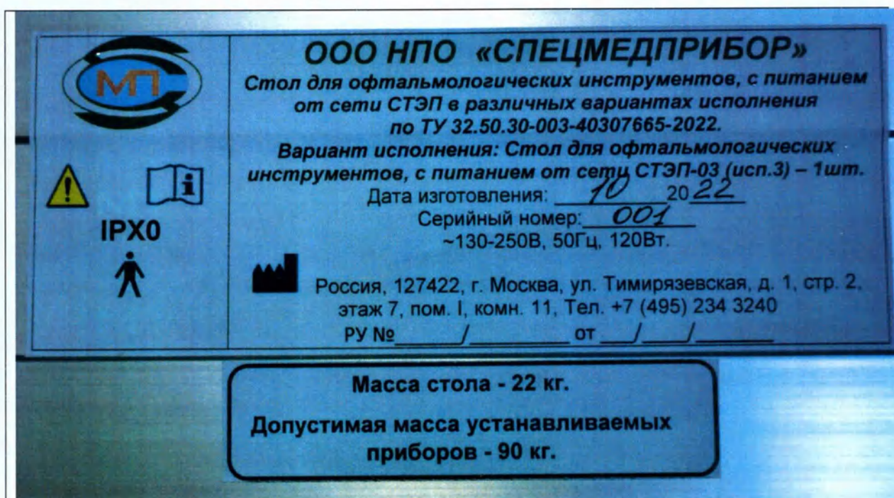
Рис.10 Шильдик СТЭП-03 (исп.3)
