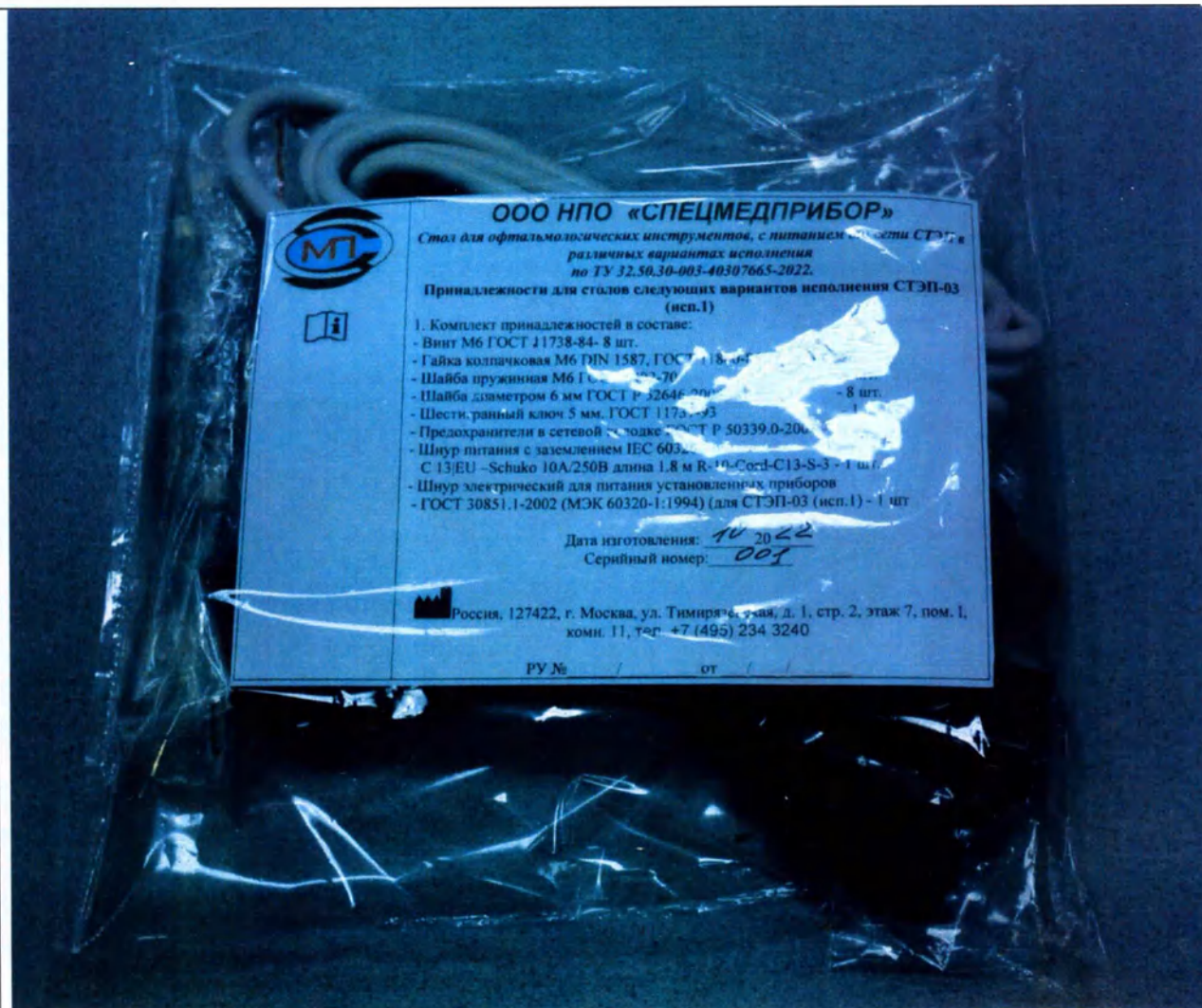
Рис.4 Комплект принадлежностей СТЭП-03 (исп.1) упакованный и промаркированный
