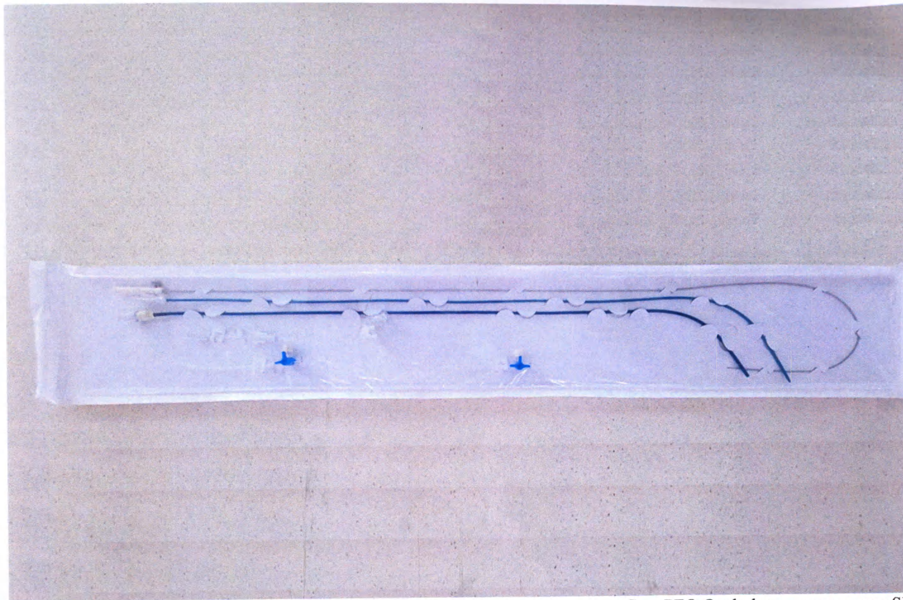
Набор SteerEase для доставки окклюдера для закрытия открытого овального окна Cera PFO Occluder, в исполнении SFA9F
